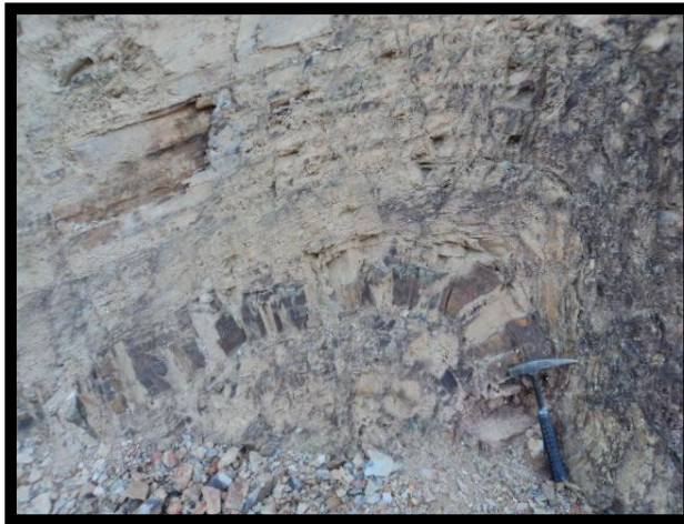
Fotografía 1.4 Intercalación de areniscas con lutitas negras.
