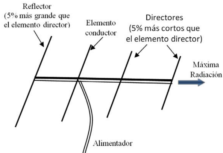
Figura 1-8 Antena tipo Yagi con reflector y directores (VHF/UHF)
