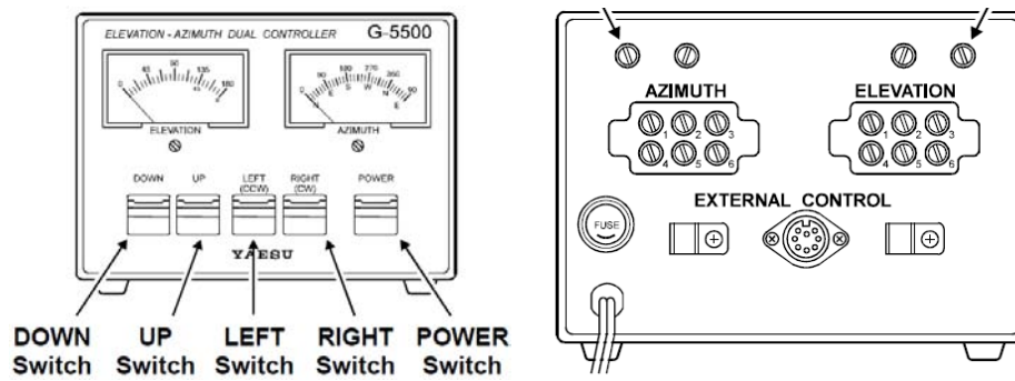
Figura 5-18 Rotor YAESU G-5500 en azimut / elevación
