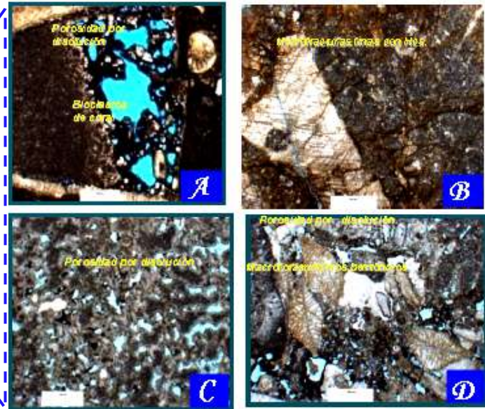
Figura 3.9. Registro de resistividad del pozo GS-1 y láminas delgadas del intervalo de interés. A. Porosidad por disolución en Bioclastos de coral., B. Microfracturas con hidrocarburos., C. Porosidad por disolución., D. Porosidad por disolución en microforaminíferos bentónicos.
