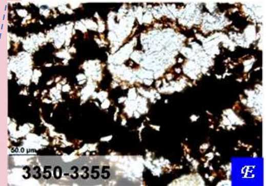
Figura 3.10. Registro Litológico del Pozo GS-2 y lámina delgada del intervalo de interés. Packstone a Grainstone de bioclastos, foraminíferos bentónicos y fragmentos de algas, café claro y gris claro, recristalizado, con porosidad primaria interfosilar y secundaria intercrystalina por microfracturas algunas selladas por calcita; se observa buena impregnación de aceite pesado.
