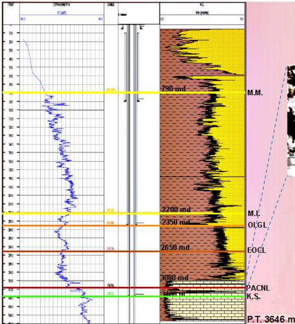
Figura 3.10. Registro Litológico del Pozo GS-2 y lámina delgada del intervalo de interés. Packstone a Grainstone de bioclastos, foraminíferos bentónicos y fragmentos de algas, café claro y gris claro, recristalizado, con porosidad primaria interfosilar y secundaria intercrystalina por microfracturas algunas selladas por calcita; se observa buena impregnación de aceite pesado.
