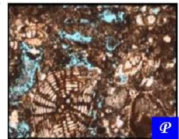
Figura 3.16. Lámina delgada del intervalo 3680-3688m. O-P. 3688m Packstone a Grainstone de briozoarios, moluscos.
