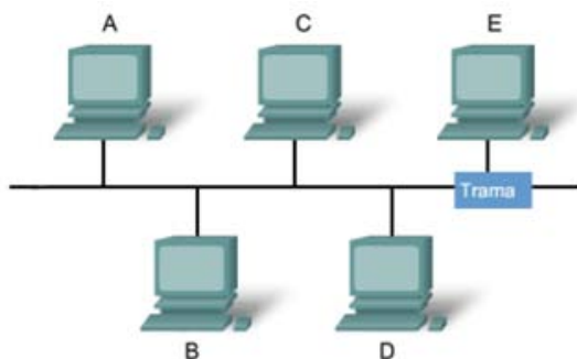
Figura 1. 3 Topología Multiacceso
