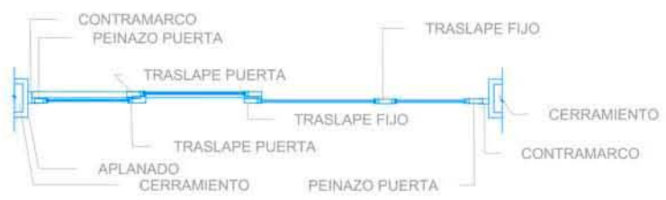
SECCION HORIZONTAL
