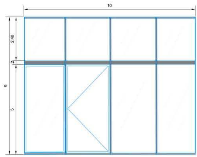
PUERTA TIPO ①
