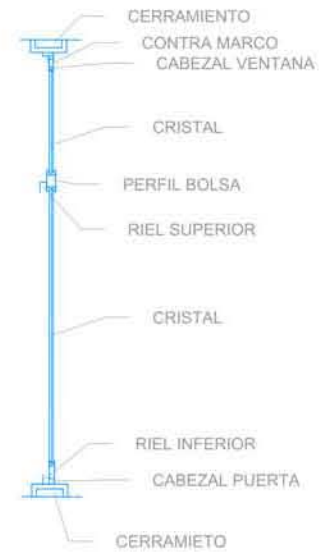
SECCION VERTICAL
