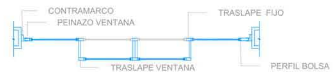
SECCION HORIZONTAL
