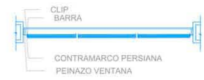
SECCION HORIZONTAL
