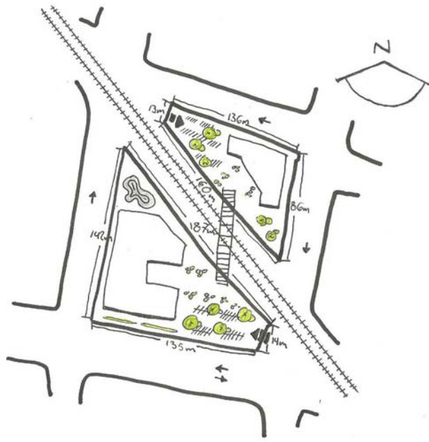
MPLAZAMIENTO
