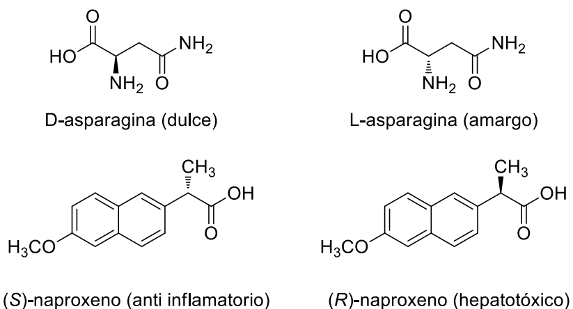
Figura 3. Estructuras enantioméricas de naproxeno y asparagina.
