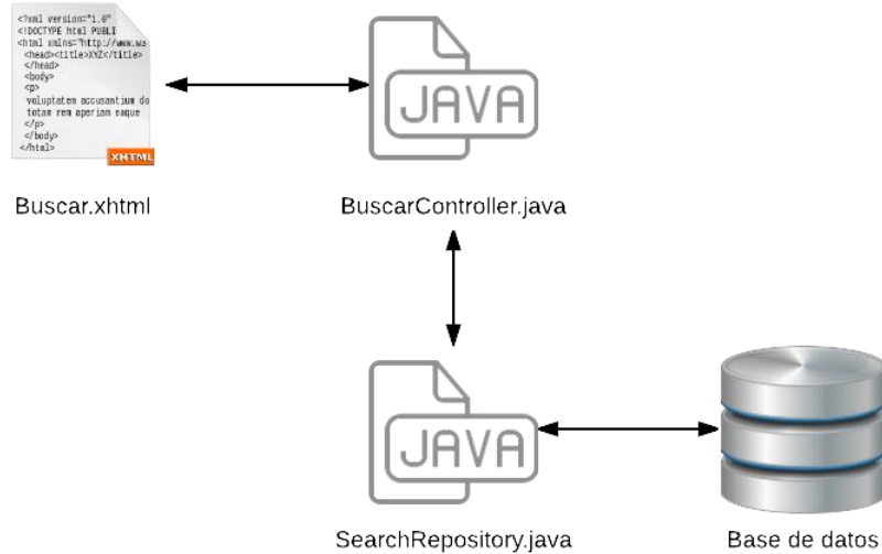
Figura 21: Modelo vista controlador
