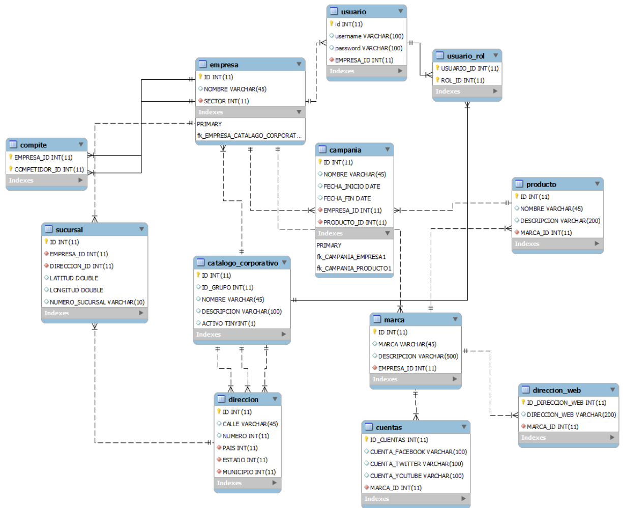
Figura 8: Diagrama de la base de datos del sistema
