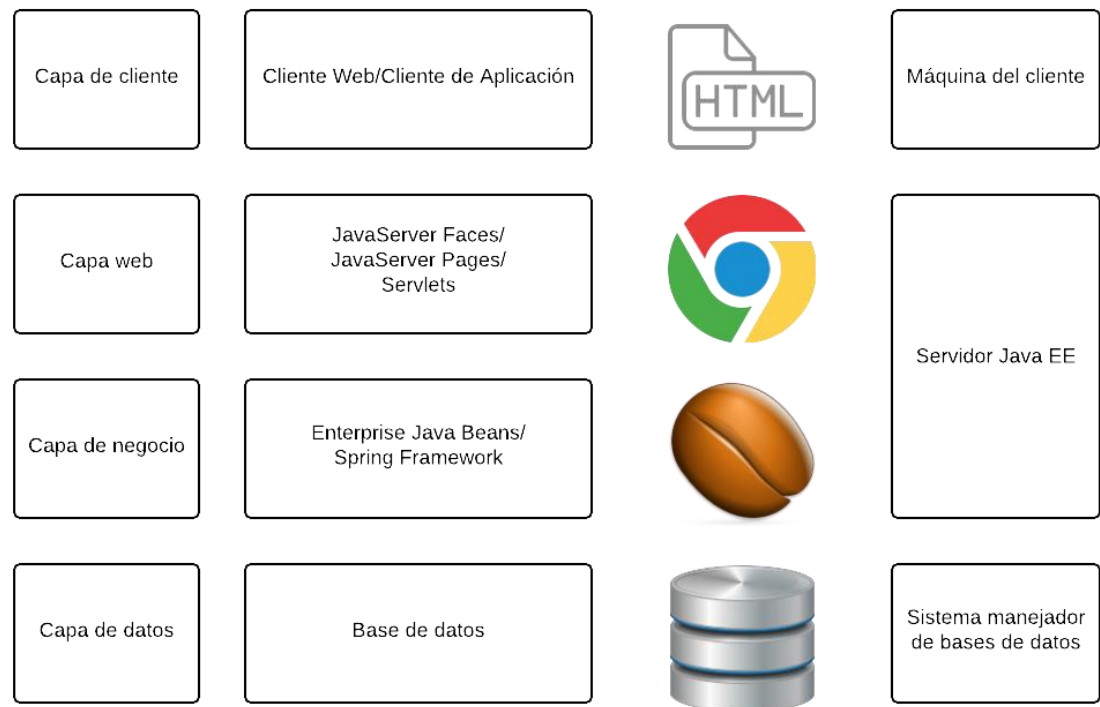
Figura 4: Diseño de capas en Java Enterprise Edition
