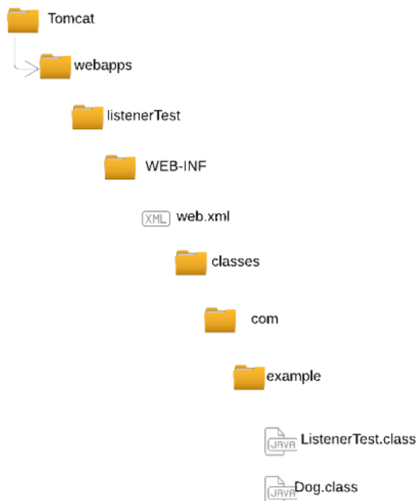
Figura 56: Estructura de directorios Apache Tomcat
