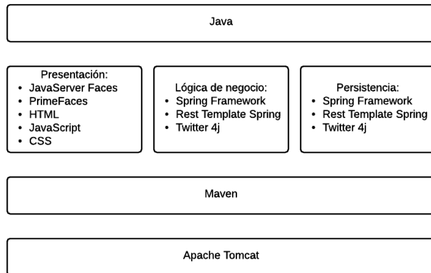
Figura 7: Arquitectura del sistema
