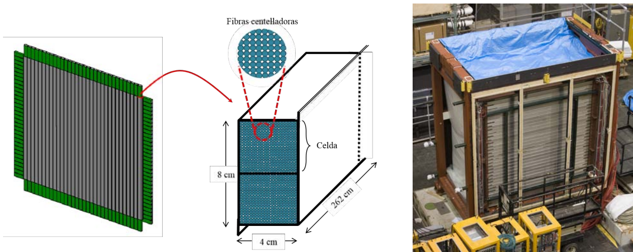
(a) Esquema del detector de electrones y de la sección transversal de uno de sus módulos.
