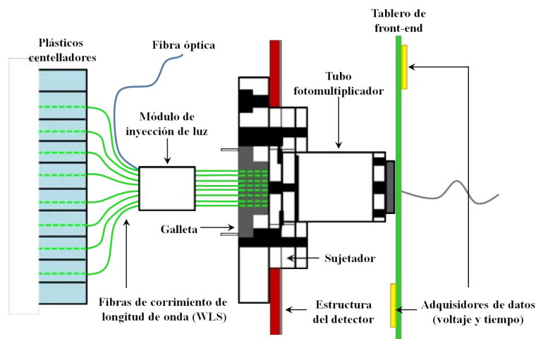
Figura 2.5: Las fibras de corrimento de longitud de onda se acoplan a los tubos fotomultiplicadores a través de un artefacto conocido como galleta . El módulo de inyección de luz se localiza entre los plásticos centelladores y los fototubos. Cada fototubo está montado sobre un tablero de front-end.
