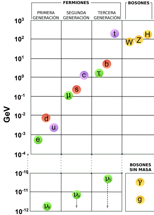
Figura 1.4: Escala de masas en el modelo estándar.
