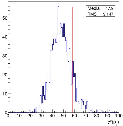
(a) Distribución de valores en el punto de nula oscilación \mathbf{p}_v = (0, 0\text{eV}^2) .
