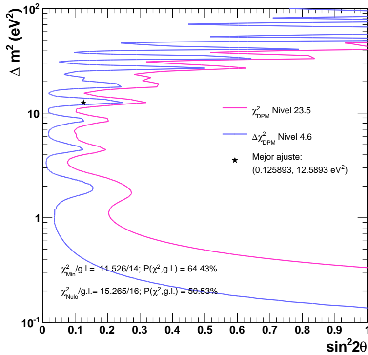
Figura 5.1: Límites al 90% N.C. de los parámetros de oscilación \sin^2 2\theta y \Delta m^2 obtenida con el método de Pearson considerando únicamente las observaciones en el detector de MiniBooNE. Las regiones excluidas se obtuvieron cortando las superficies \chi^2_{DPM} y \Delta\chi^2_{DPM} con planos a 23.5 y 4.6 respectivamente.
