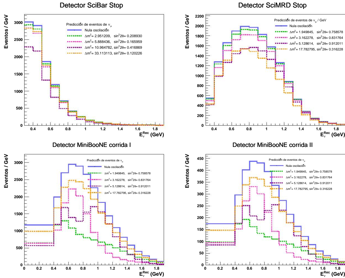
Figura 4.1: Predicción de distribuciones de E_{\nu_\mu}^{Rec} en los detectores SciBar (esquina superior izquierda), en SciMRD (esquina superior derecha) y en MiniBooNE corrida I y corrida II (esquina inferior izquierda y derecha, respectivamente) para distintos parámetros de oscilación.
