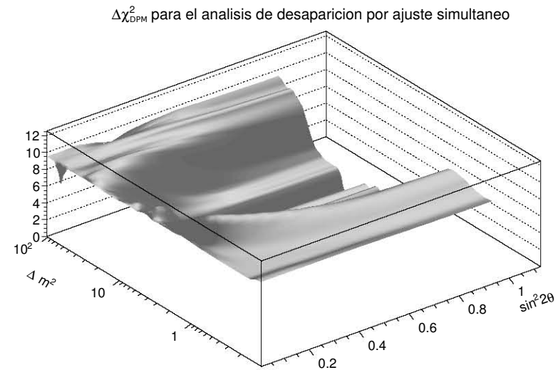
(b) Superficie \Delta\chi_{DPM}^2 frequentista
