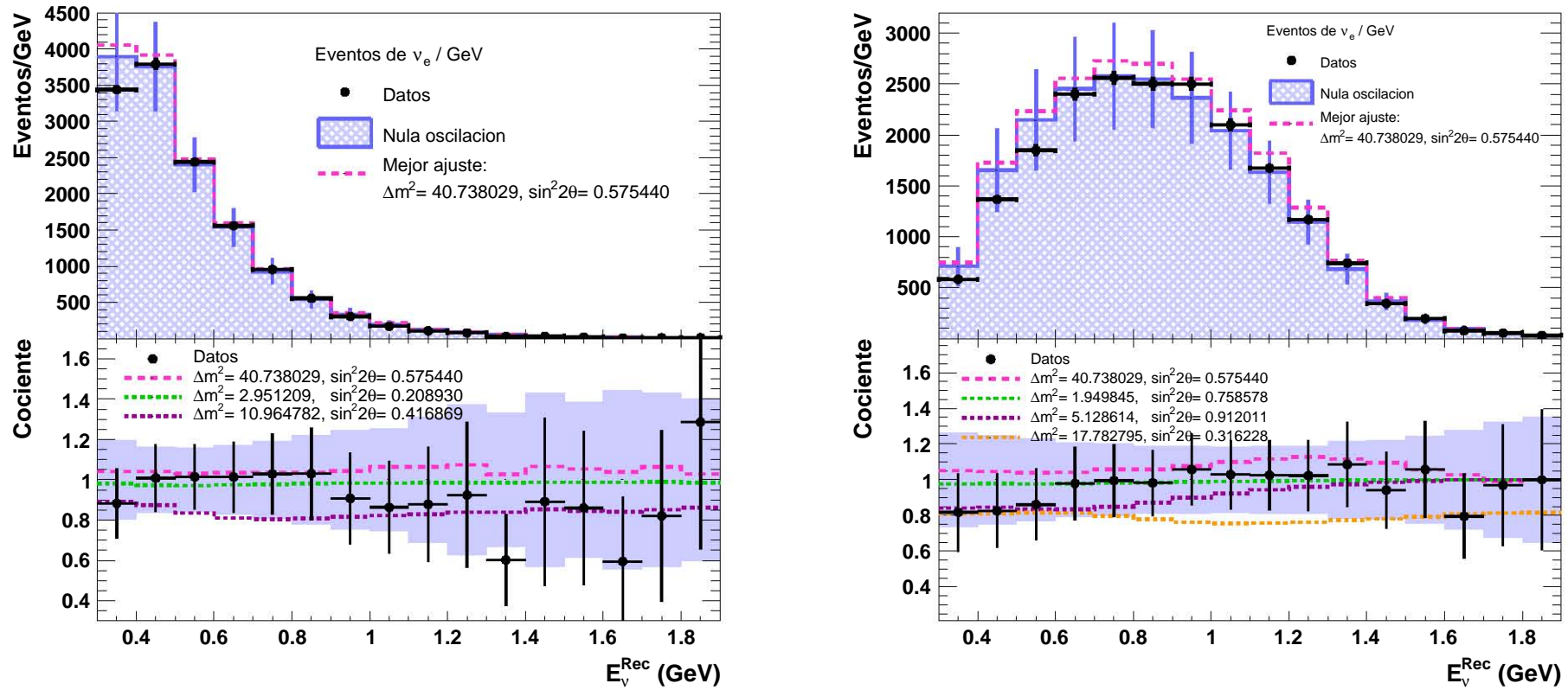
Figura 5.6: Histogramas de eventos de \nu_{\mu} observados en los detectores de SciBooNE y cociente de las predicciones con respecto al punto de nula oscilación. Arriba a la izquierda: Distribución de E_{\nu}^{Rec} para \nu_{\mu} detectados en SciBar (puntos con error estadístico), distribución para la hipótesis de nula oscilación relativamente normalizada a los datos de SciBooNE (histograma sombreado con incertidumbre sistemática) y distribución para el mejor ajuste de forma (histograma punteado). Abajo a la izquierda: Cociente con respecto a la hipótesis de nula oscilación para predicciones con distintos parámetros de oscilación \sin^2 2\theta, \Delta m^2 . La banda sombreada corresponde al tamaño de la diagonal de la matriz de error sistemático. A la derecha: Lo análogo para el detector SciMRD.
