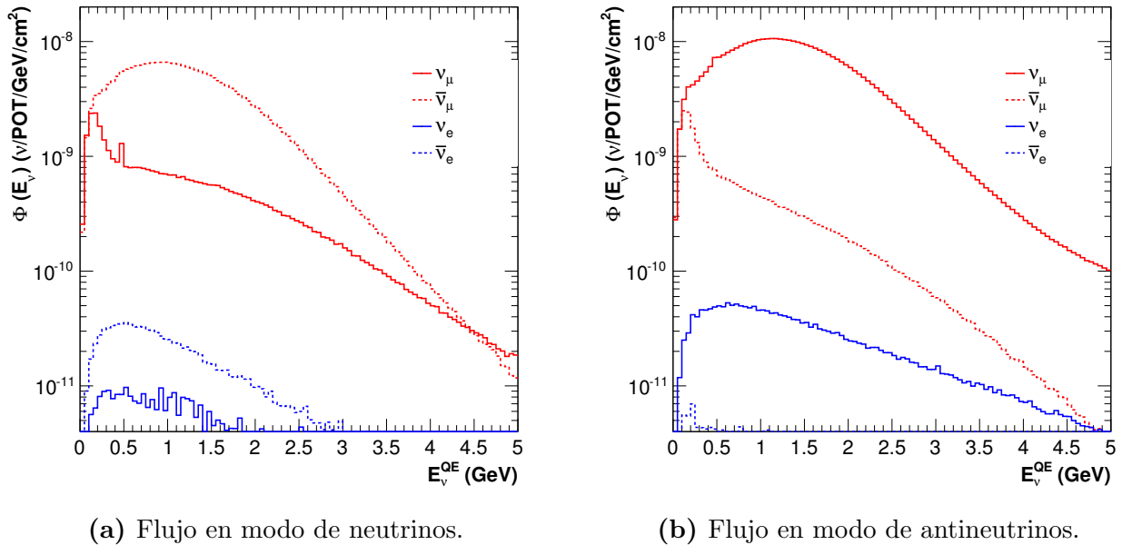
Figura 3.1: Predicción del flujo de neutrinos en SciBooNE para el corno en polaridad positiva (modo de neutrinos) y negativa (modo de antineutrinos).
