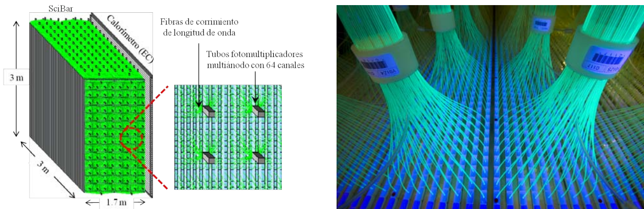
(a) Esquema de la estructura de SciBar. El haz de neutrinos incide por la izquierda de la figura [76].
