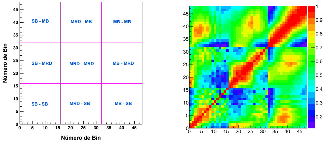
(a) Esquema de la correlación entre bins de los detectores SciBar (SB), SciMRD (MRD) y MiniBooNE (MB).
