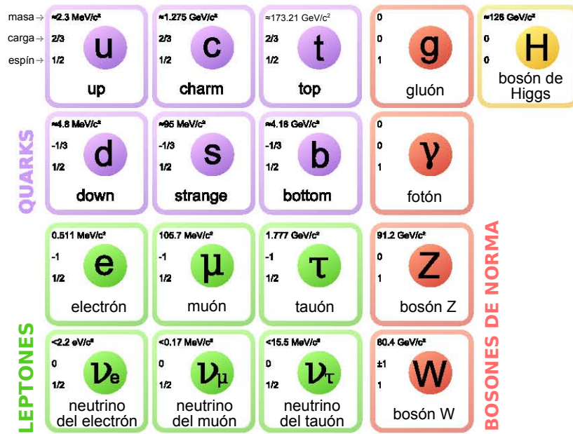
Figura 1.3: Modelo estándar de partículas elementales. Las primeras tres columnas representan las tres generaciones de partículas en donde las primeras dos filas corresponden a los quarks y el siguiente par a los leptones. La cuarta columna muestra a los bosones de norma y en la quinta el bosón de Higgs.
