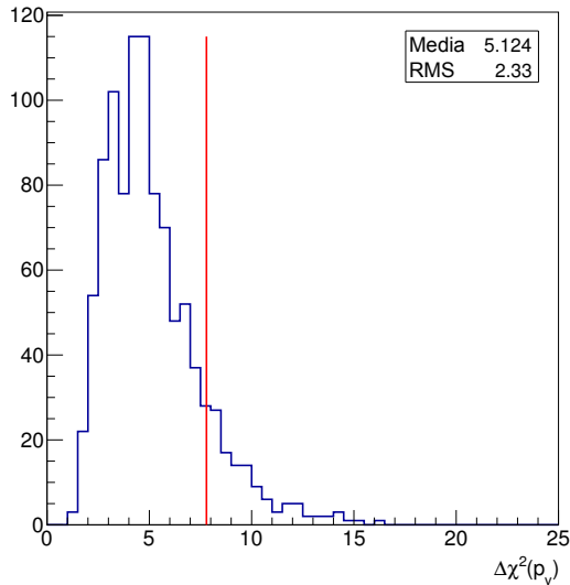
(c) Distribución de valores \Delta\chi^2(\mathbf{p}_v) en el punto de nula oscilación \mathbf{p}_v = (0, 0\text{eV}^2) .
