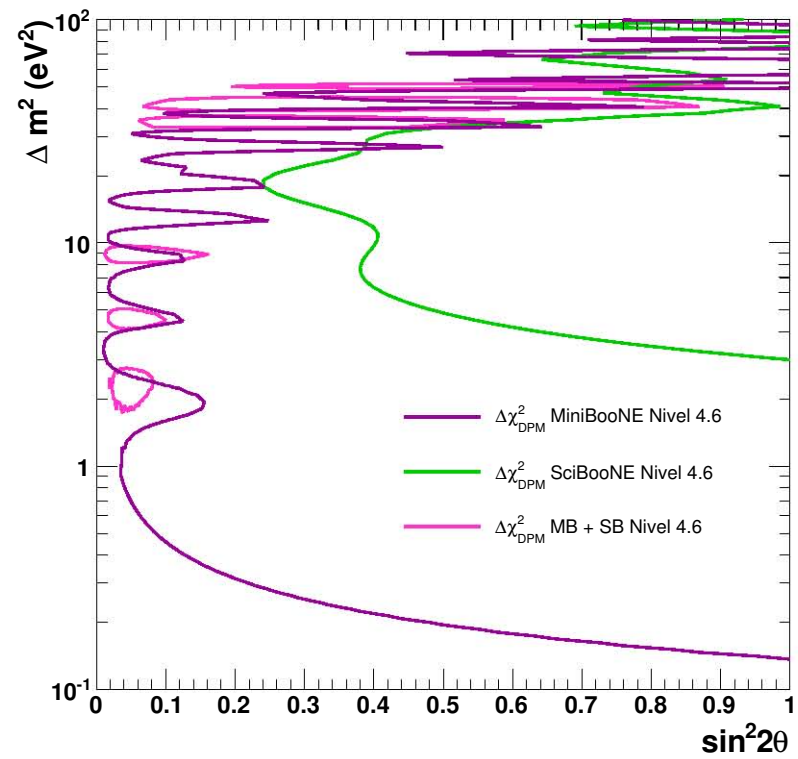
Figura 5.4: Límites de exclusión de (\sin^2 2\theta, \Delta m^2) al nivel 90% N.C. En la imagen izquierda se muestran las regiones obtenidas cortando los estadísticos \chi^2 con planos en 23.5, 42.6 y 60.8 para MiniBooNE, SciBooNE y MiniBooNE + SciBooNE, respectivamente. A la derecha se presentan las regiones obtenidas al cortar \Delta\chi^2 en 4.6 para los tres casos (solo MiniBooNE, solo SciBooNE y MiniBooNE + SciBooNE).
