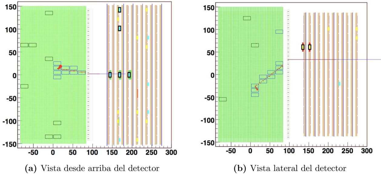
Figura 3.4: Evento de dispersión cuasi-elástica de corriente cargada \nu_{\mu}n \rightarrow \mu^{-}p en SciBooNE. La región verde corresponde a la región de SciBar, pegada a su derecha, la línea vertical representa al EC y la región más oscura a la derecha es el MRD; la escala está en centímetros. La traza roja más pequeña corresponde a la traza de un protón; la más larga es la asociada a un muón.
