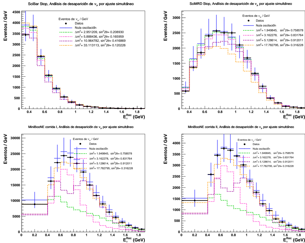
Figura 4.5: Predicción de distribuciones normalizadas a los datos de SciBooNE en los detectores en SciBar (esquina superior izquierda), en SciMRD (esquina superior derecha) y en MiniBooNE corrida I y corrida II (esquina inferior izquierda y derecha, respectivamente) para distintos parámetros de oscilación. Los puntos corresponden a los datos con su incertidumbre estadística. Las líneas verticales asociadas a la predicción en el punto de nula oscilación corresponden a la incertidumbre sistemática.
