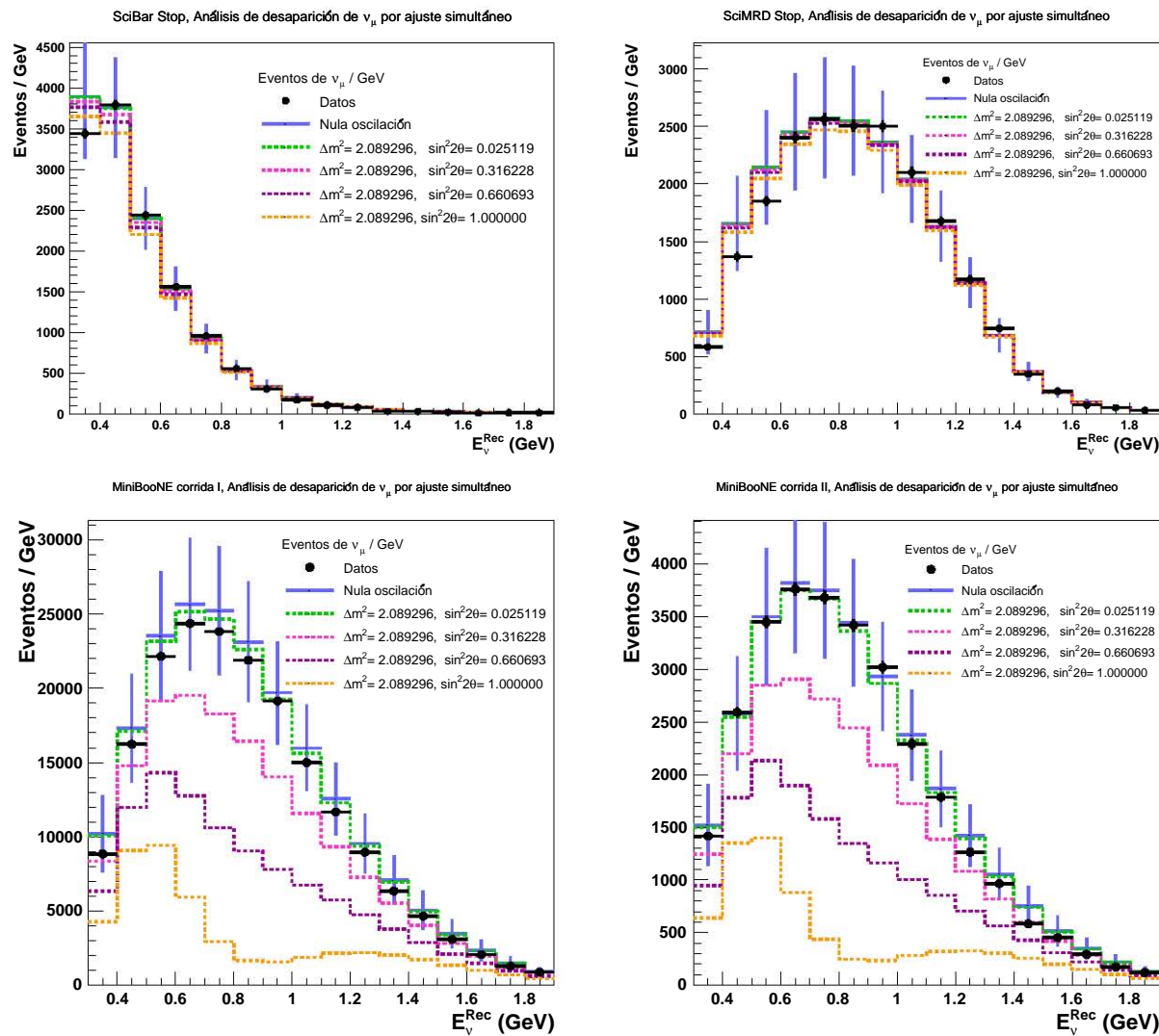
Figura 4.6: Predicción de distribuciones normalizadas a los datos de SciBooNE en los detectores SciBar (esquina superior izquierda), SciMRD (esquina superior derecha) y en MiniBooNE corrida I y corrida II (esquina inferior izquierda y derecha, respectivamente) para \Delta m^2 fijo y distintos valores de \sin^2 2\theta . Los puntos corresponden a los datos con su incertidumbre estadística. Las líneas verticales asociadas a la predicción en el punto de nula oscilación corresponden a la incertidumbre sistemática.
