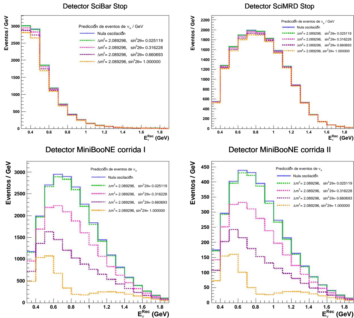
Figura 4.2: Predicción de distribuciones de E_{\nu_{\mu}}^{Rec} en los detectores SciBar (esquina superior izquierda), SciMRD (esquina superior derecha) y en MiniBooNE corrida I y corrida II (esquina inferior izquierda y derecha, respectivamente) para \Delta m^2 fijo y distintos valores de \sin^2 2\theta .
