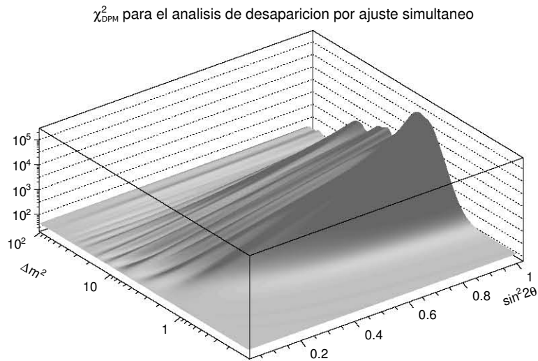
(a) Superficie \chi_{DPM}^2 de Pearson.
