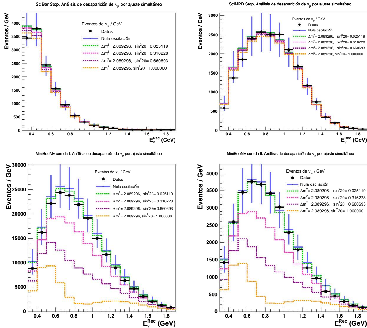
Figura 4.4: Predicción de distribuciones normalizadas con el factor en el punto de nula oscilación en los detectores SciBar (esquina superior izquierda), SciMRD (esquina superior derecha) y en MiniBooNE corrida I y corrida II (esquina inferior izquierda y derecha, respectivamente) para \Delta m^2 fijo y distintos valores de \sin^2 2\theta . Los puntos corresponden a los datos con su incertidumbre estadística. Las líneas verticales asociadas a la predicción en el punto de nula oscilación corresponden a la incertidumbre sistemática.
