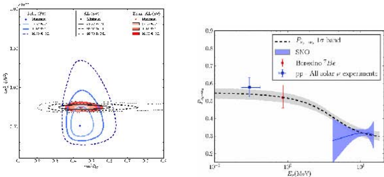
Figura 1.10: Resultado global de experimentos con neutrinos solares. A la izquierda se muestra el resultado del análisis de oscilación de neutrinos solares con un modelo de 3 neutrinos combinando los datos de SNO, KamLAND y de experimentos a cortas distancias. A la derecha se muestra la probabilidad de supervivencia de \nu_e solares como función de la energía [32].
