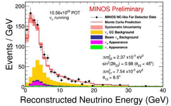
(b) Resultado preliminar del espectro de energías de neutrinos en MINOS+ comparado con la predicción de eventos de corriente neutra en el detector cercano incluyendo el ruido y las incertidumbres sistemáticas totales. La predicción asume un modelo de 3 sabores de neutrinos con parámetros \Delta m_{21}^2 = 7.59 \times 10^{-5} \text{eV}^2 , \Delta m_{32}^2 = 2.41 \times 10^{-3} \text{eV}^2 , \sin^2 \theta_{13} = 0.024 , \sin^2 2\theta_{23} = 0.319 y \sin^2 2\theta_{23} = 0.388 en donde no se encuentra evidencia de una desviación del modelo con tres neutrinos.
