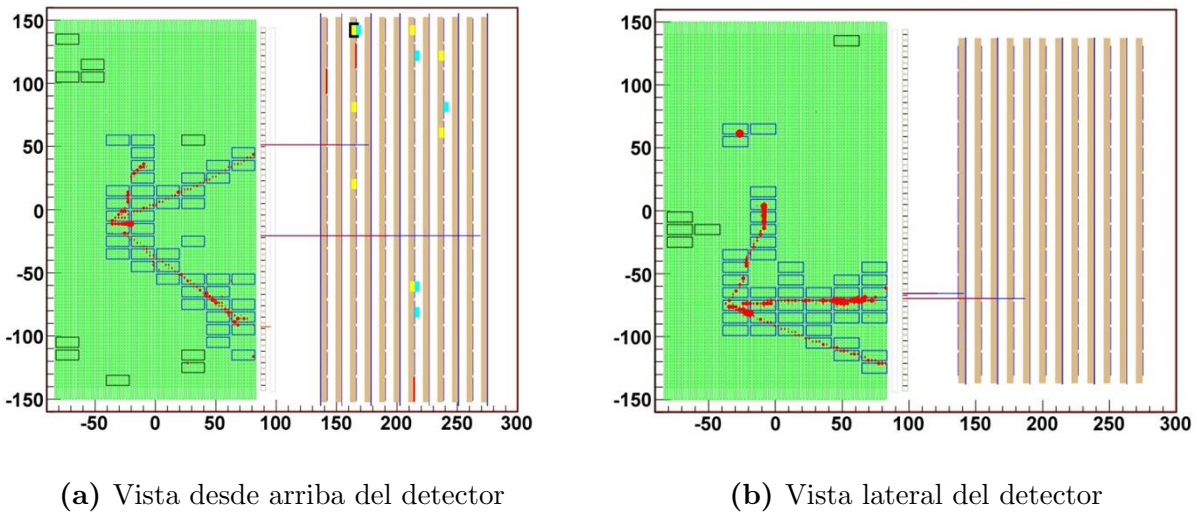
Figura 3.5: Evento con tres trazas en SciBooNE: producción de piones \nu_{\mu}p \rightarrow \mu^{-}p\pi^{+} . La región verde corresponde a la región de SciBar, pegada a su derecha, la línea vertical representa al EC y la región más oscura a la derecha es el MRD. En la imagen (b) la traza roja más pequeña corresponde a la traza de un protón; la línea horizontal correspondiente a un muón que llega hasta el MRD mientras que la restante es la traza de un pión.
