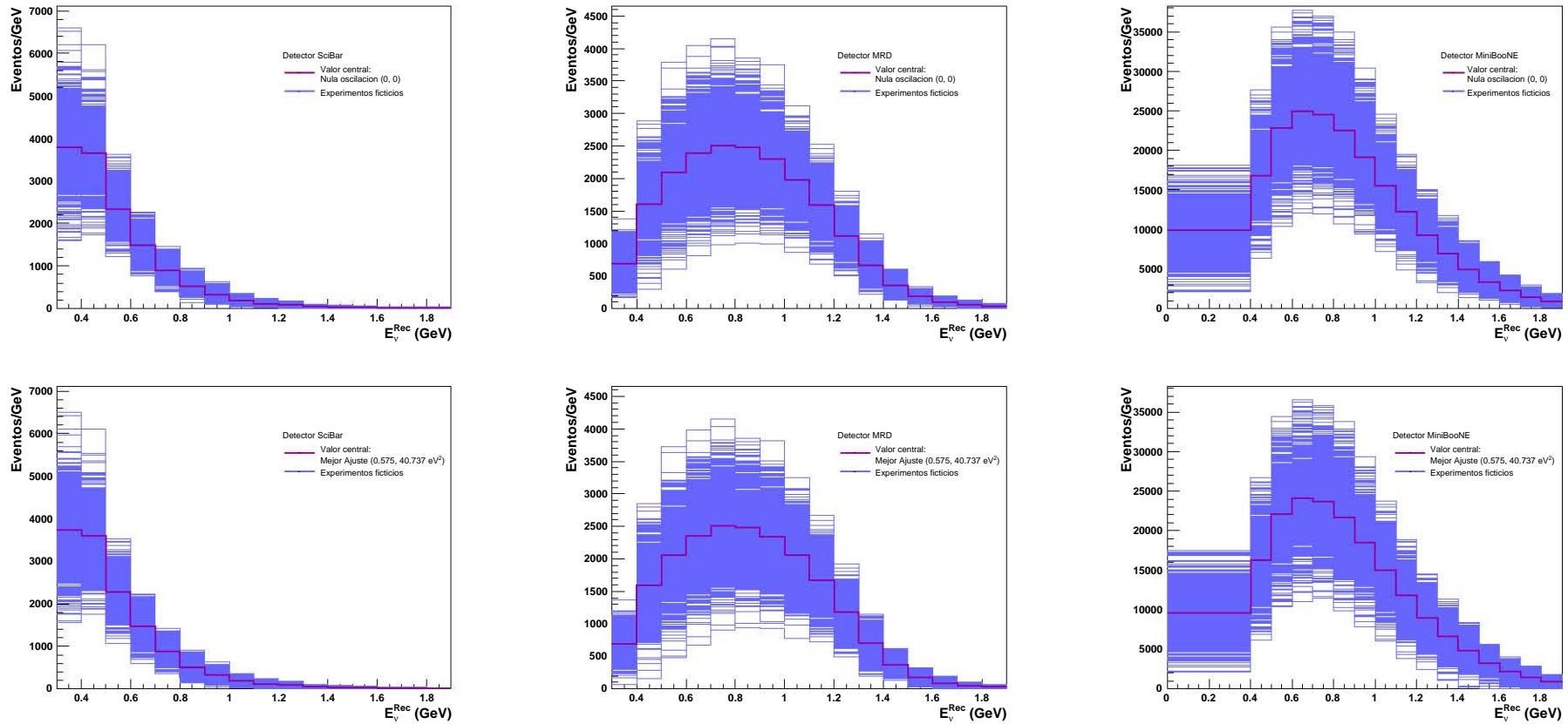
Figura 4.8: Efecto de la perturbación alrededor de los histograma de predicción con los parámetros ( \sin^2 2\theta = 0, \Delta m^2 = 0\text{eV}^2 ) y ( \sin^2 2\theta = 0.575, \Delta m^2 = 40.738\text{eV}^2 ), primera y segunda hilera respectivamente. Se muestra el efecto que tiene sumar un vector aleatorio con media en 0 y \sigma = 1 en el vector de predicción \mathbf{P} , mostrado en rojo, para generar vectores de experimentos ficticios \mathbf{F} que cumplan con la misma pareja ( \sin^2 2\theta, \Delta m^2 ) en los detectores SciBar (izquierda), SciMRD (centro) y MiniBooNE (derecha).
