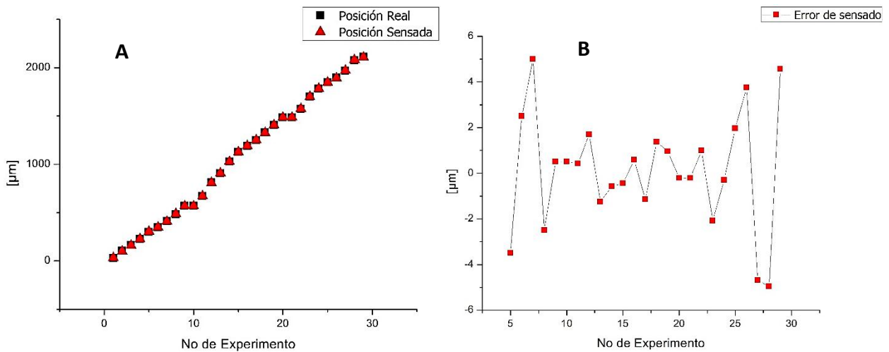
Figura 66. (A) Comparación del desplazamiento medido por el sistema de sensado y el por el proyector de perfiles en 30 posiciones diferentes. (B) Errores de posición sensada con respecto a la posición real.
