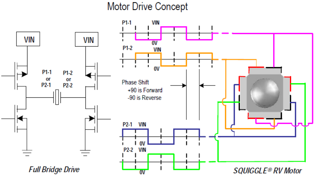
Figura 45. Concepto del control del motor SQL-RV-1.8 con el driver NSD-2101 [22].
