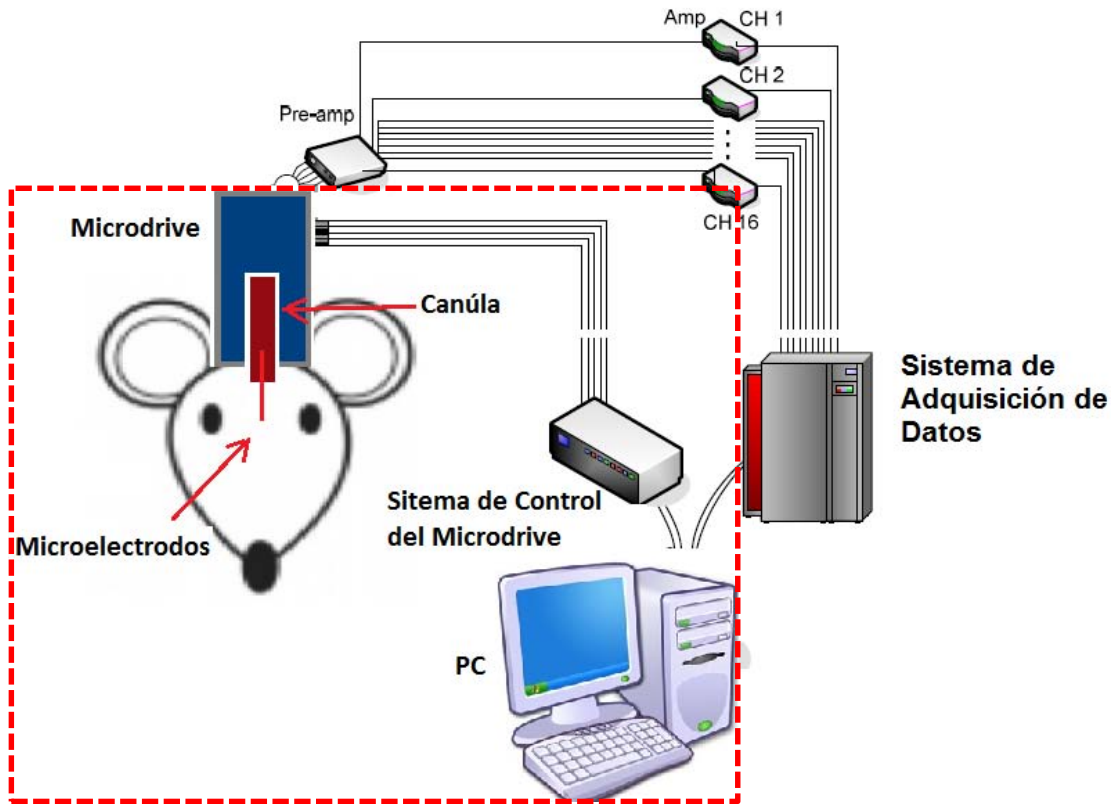
Figura 42. Diagrama esquemático de un sistema completo de registro de actividad neuronal [15]. El recuadro de línea punteada delimita el sistema de microposicionamiento y el resto corresponde al sistema de adquisición de las señales eléctricas de las neuronas.
