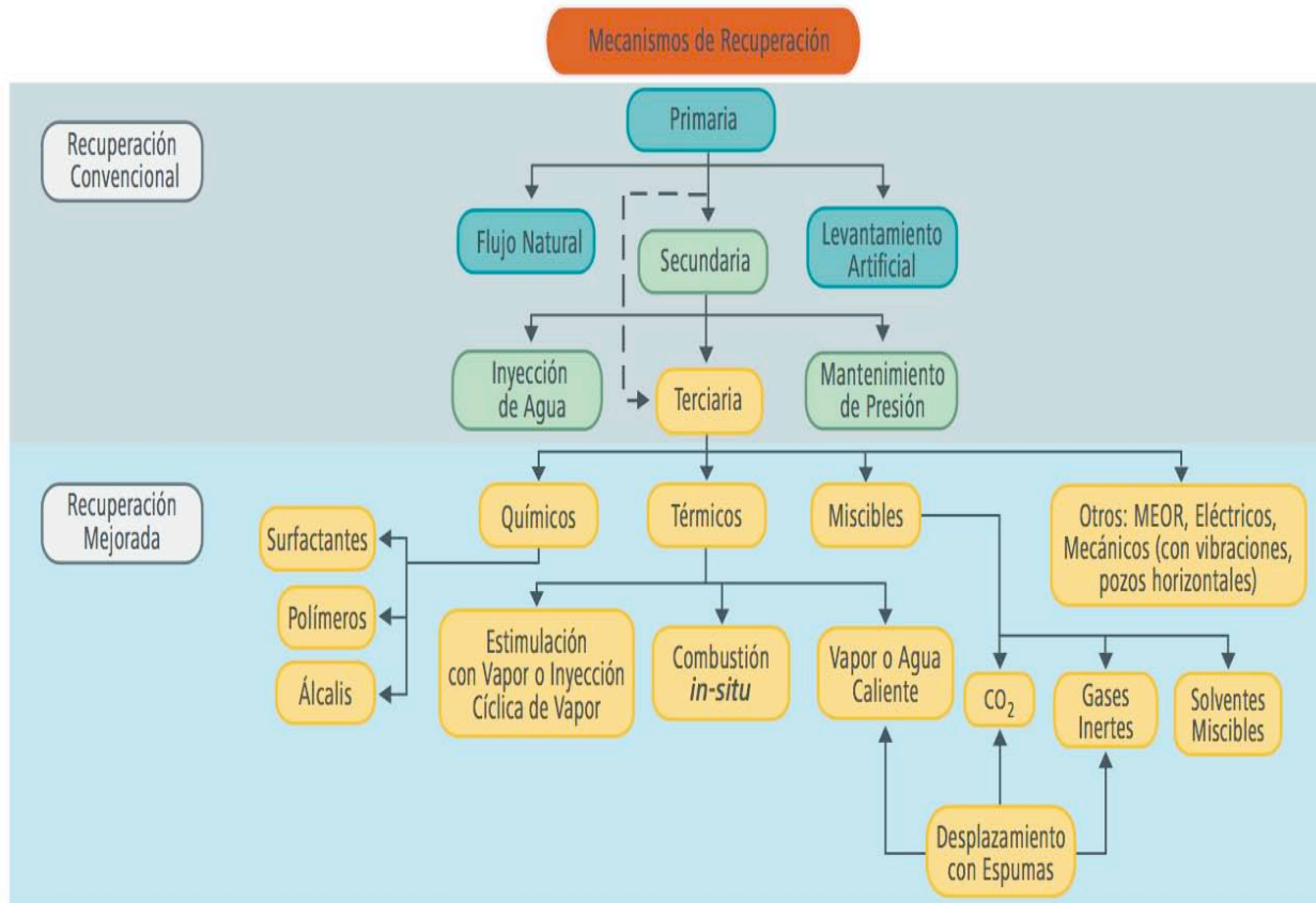
Figura 5.4 Clasificación tradicional de los métodos de recuperación (Tomada de CNH, 2012).
