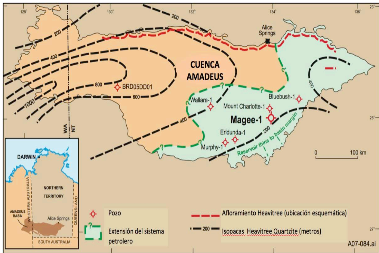
Figura 3.18 Mapa que muestra la extensión del sistema petrolero Gillen Member-Heavitree Quartzite. El play se limita a la porción sur de la cuenca debido a las grandes profundidades de sepultamiento de la porción norte (Tomada de Young y Ambrose, 2010).
