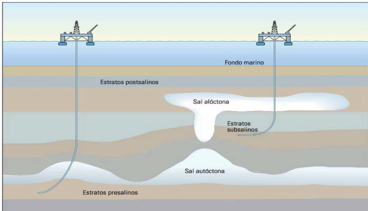
Figura 1.3 Estratos subsalinos y presalinos. Las estructuras de sal alóctona se forman a partir de las capas de sal autóctona de gran espesor. Ambos tipos de sal pueden formar trampas para los hidrocarburos en migración (Tomada de Beasley et al., 2010).
