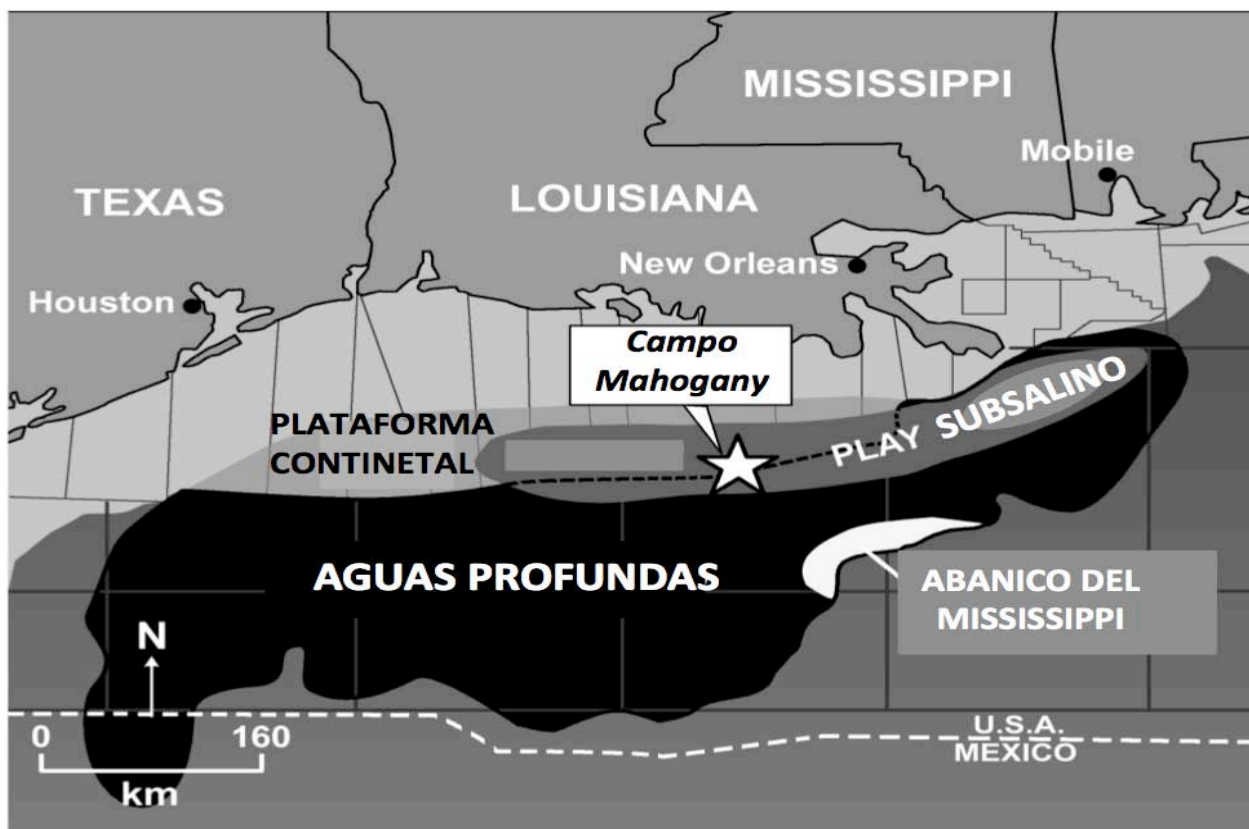
Figura 3.13 Ubicación del Campo Mahogany y el área del play subsalino costa afuera del Golfo de México. La zona potencial de plays se extiende hasta 240 km al sur del margen actual de la plataforma hacia el Escarpe Sigsbee (Modificada de Camp, 1998).
