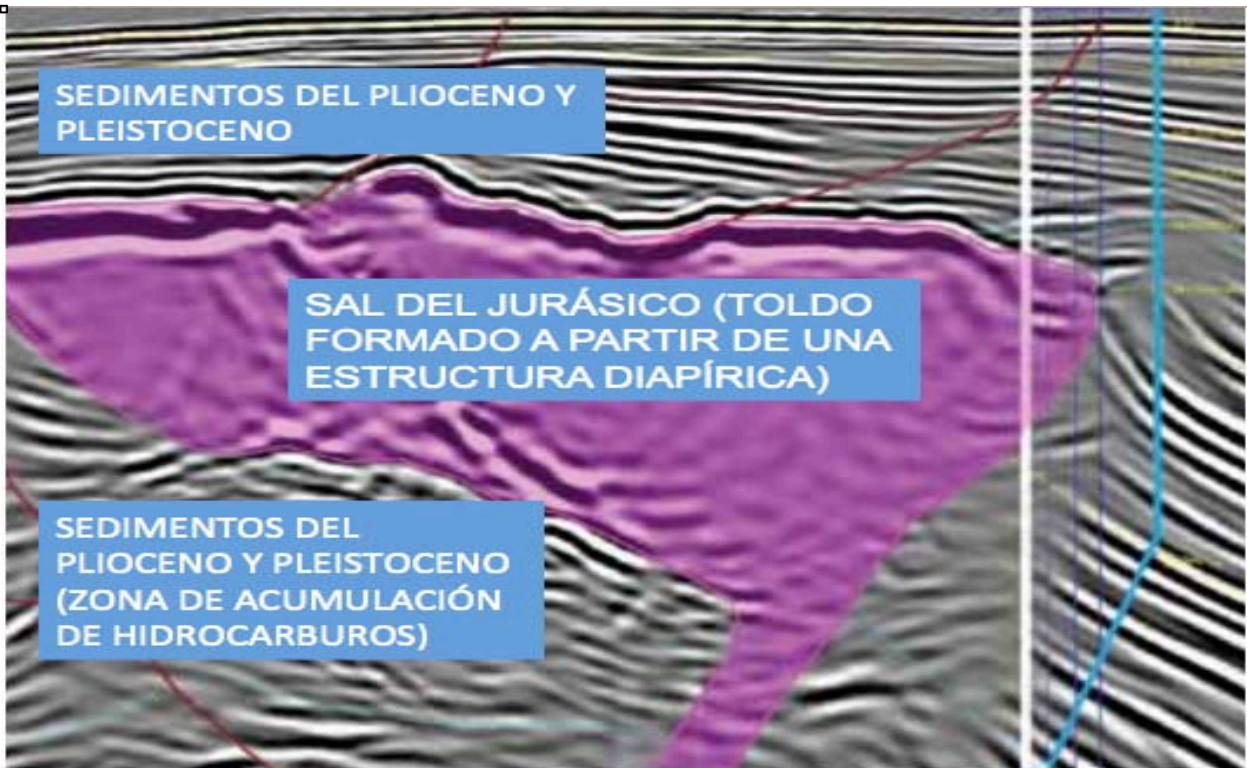
Figura 2.3 Toldo o canopy cubriendo una zona de acumulación de hidrocarburos en sedimentos mucho más jóvenes que la sal (Modificada de Vallejo et al., 2013).
