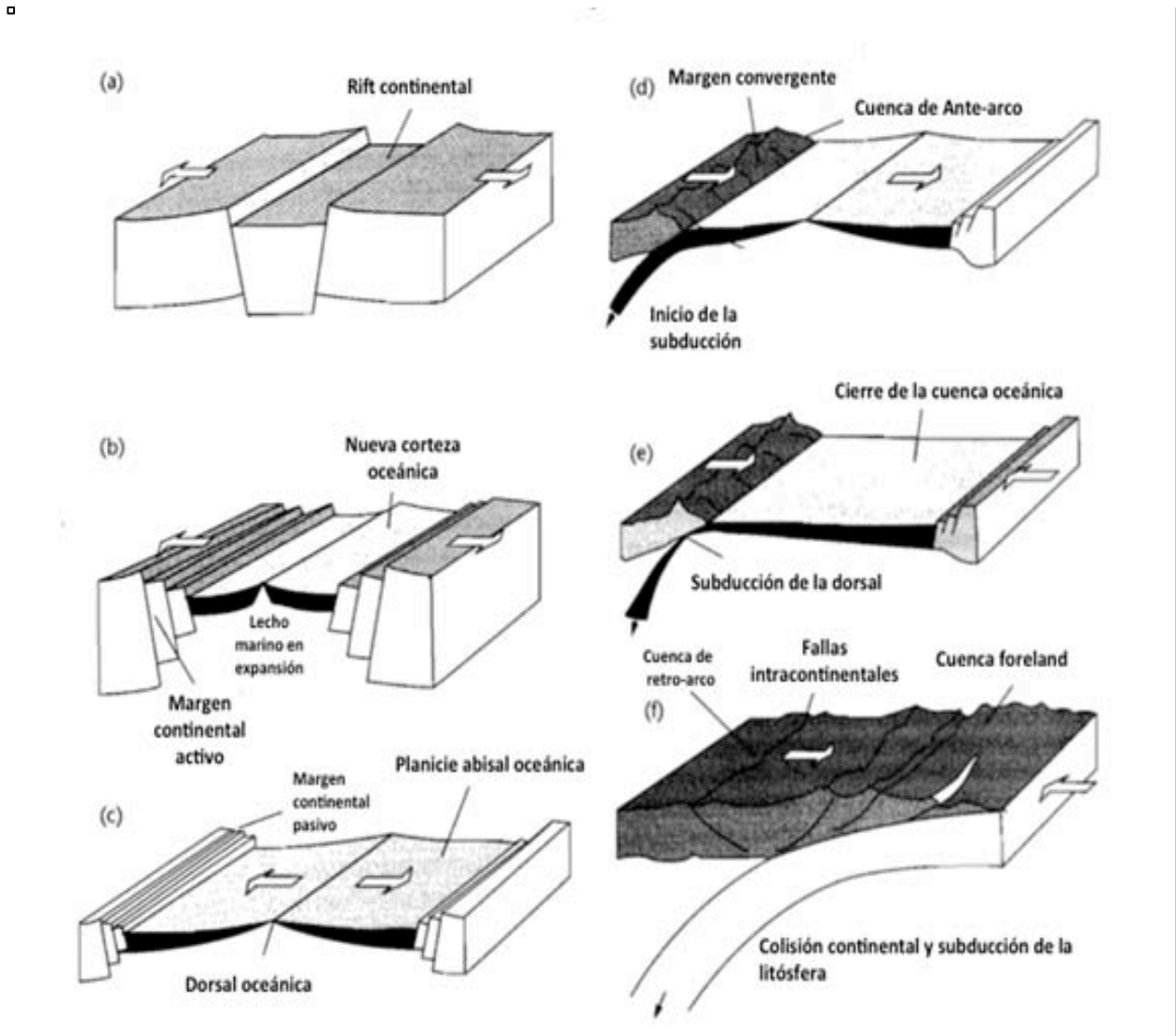
Figura 1.2 Ciclo de Wilson de formación y cierre oceánicos. La extensión continental (a) es seguida por la creación de nueva corteza oceánica (b) y la expansión de la misma (c). La subducción del piso oceánico (d) lleva al cierre de la cuenca. La subducción de la dorsal oceánica (e) tiene lugar antes de la colisión continente-continente (f) (Modificada de Allen y Allen, 2005).
