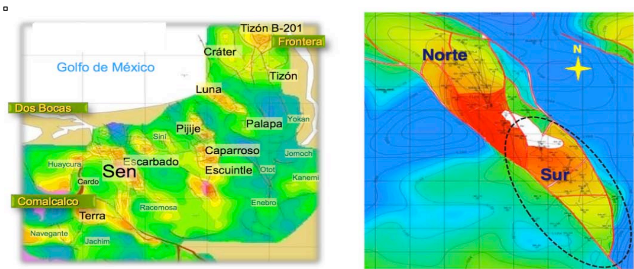
Figura 3.5 Ubicación del Campo Sen a 50 km al NE de Villahermosa (izquierda), integrado principalmente por los bloques Norte y Sur (derecha), (Modificada de Fernández et al., 2012).
