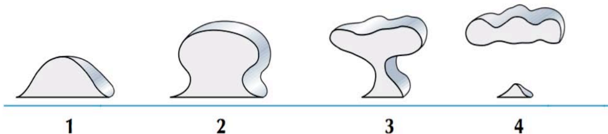
Figura 2.6 Evolución de los diapiros de sal hasta formar toldos o lengüetas. Al igual que las paredes de sal, pueden o no estar unidos al cuerpo autóctono. (Modificada de Farmer et al., 1996).
