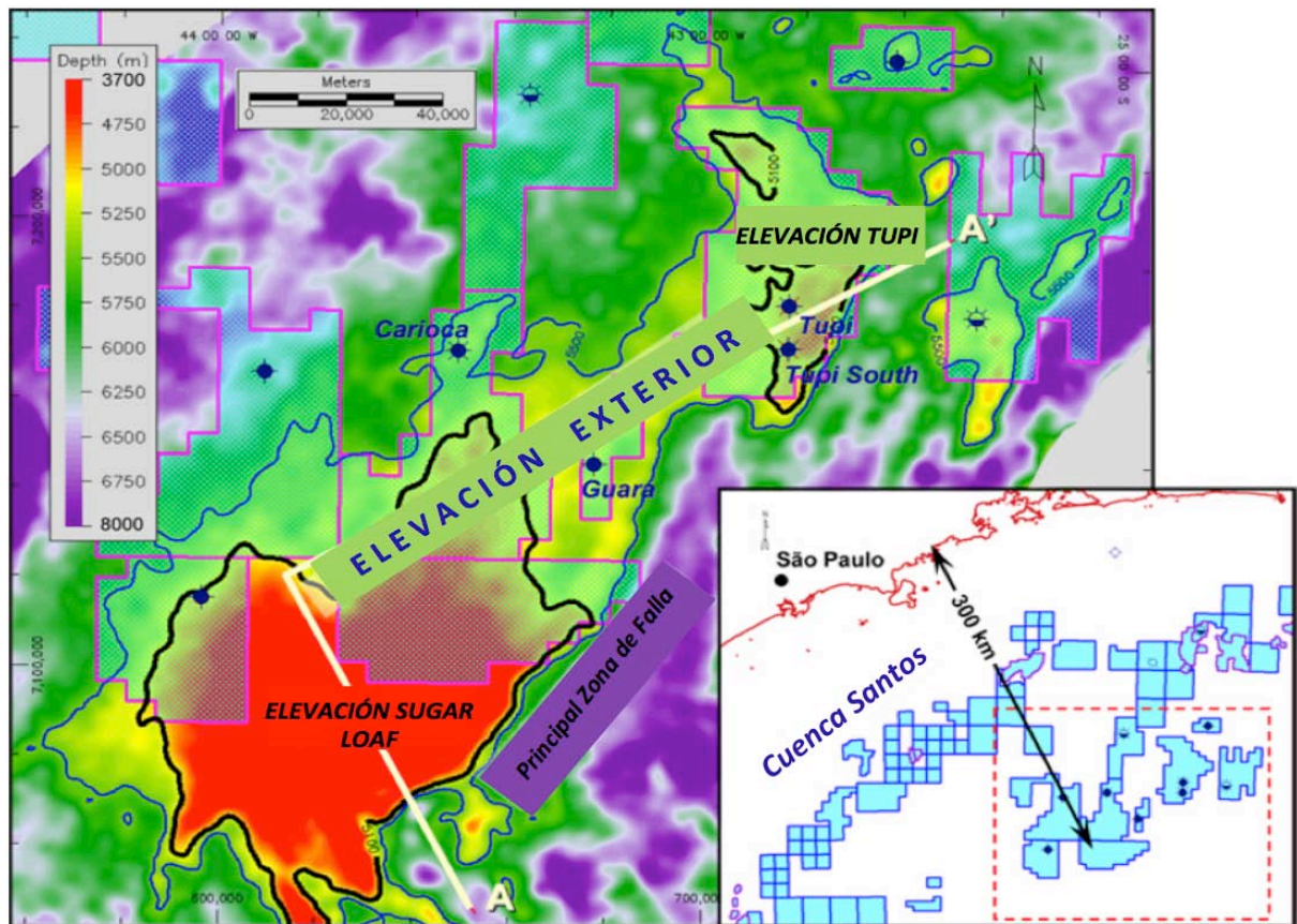
Figura 3.8 La Elevación Exterior de la Cuenca Santos (OHSB) es la característica tectónica más importante de esta cuenca y esta directamente relacionada con la ocurrencia del play presalino (el corte transversal de la sección AA' se muestra en la Figura 3.9), (Modificada de Gomes et al., 2009).
