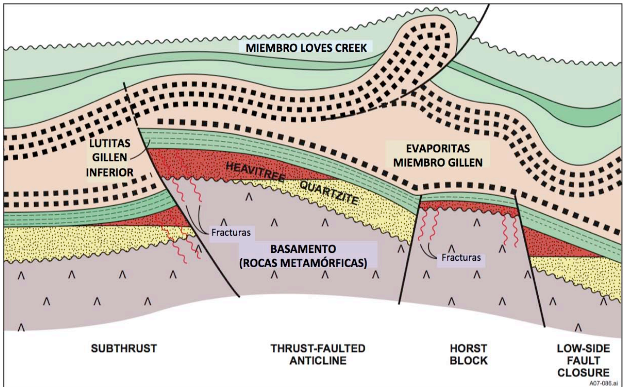
Figura 3.19 Sección transversal esquemática para ilustrar los tipos de trampas potenciales en el play Heavtree Quartzite (Tomada de Young y Ambrose, 2010).
