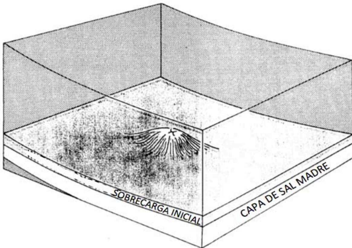
Figura 2.2 El movimiento ascendente de la sal comienza hasta que se haya depositado una cantidad suficiente de sedimentos sobre la capa madre, la cual además debe tener cuando menos un espesor aproximado de 100 m (Modificada de Halbouty, 1979).
