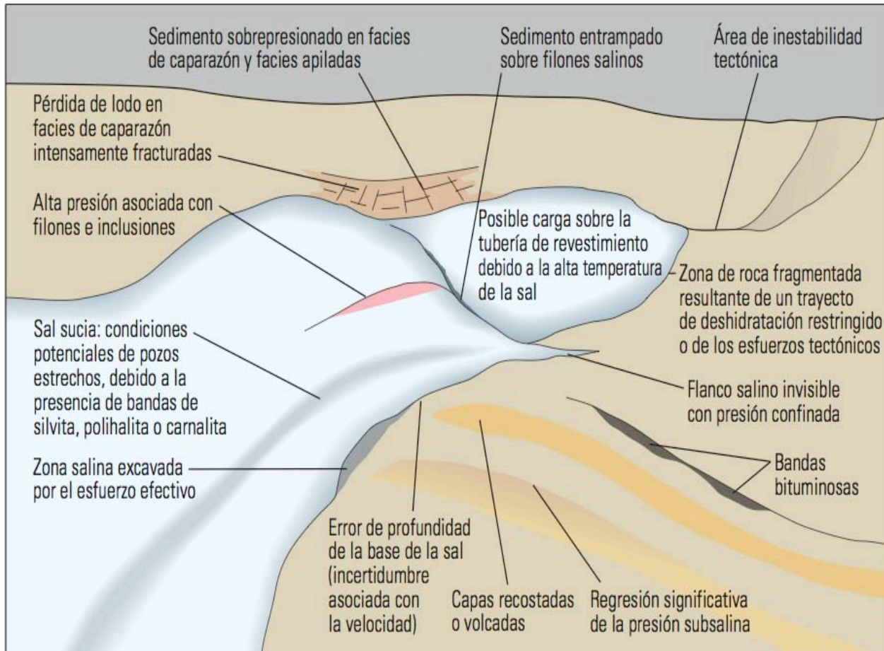
Figura 4.1 Riesgos potenciales de perforación en la sal y sus adyacencias. La probabilidad de que surjan problemas al momento de perforar, atravesar y salir de las estructuras salinas es muy alta, debido esencialmente a la tendencia al movimiento propia de la sal (Tomada de Aburto et al., 2008).
