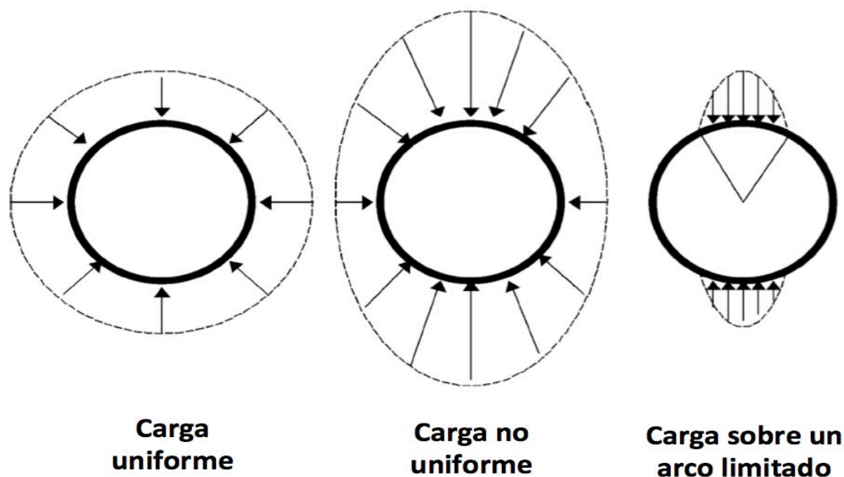
Figura 4.6 La presencia de cargas no uniformes sobre la tubería de revestimiento podría provocar su deformación y colapso. La mejor forma de evitar las cargas no uniformes es manteniendo una buena calidad de pozo en cuanto a geometría y realizando una buena cementación (Modificada de Israel et al., 2008).
