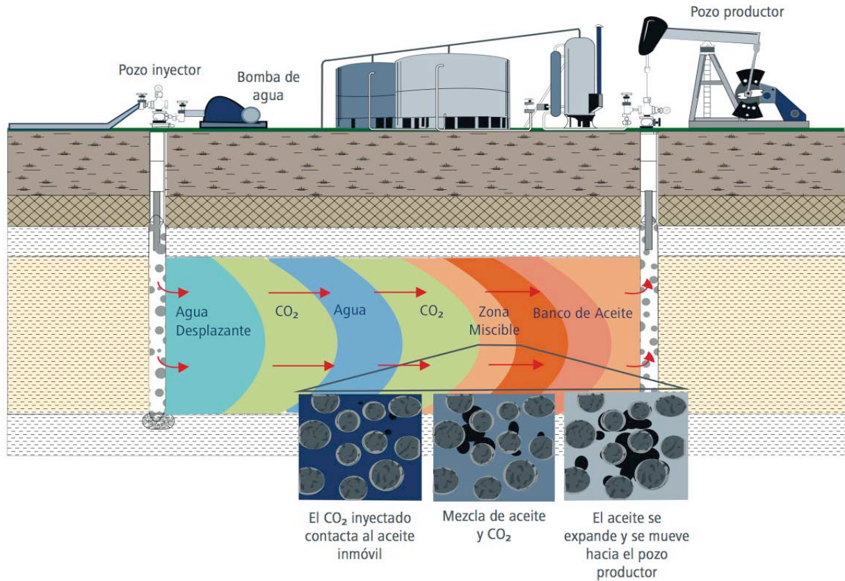
Figura 5.5 Proceso de inyección de dióxido de carbono. El dióxido de carbono se disuelve en el aceite, disminuyendo su viscosidad e incrementando la eficiencia de barrido mediante un bache de fluido desplazante (Tomada de CNH, 2012).
