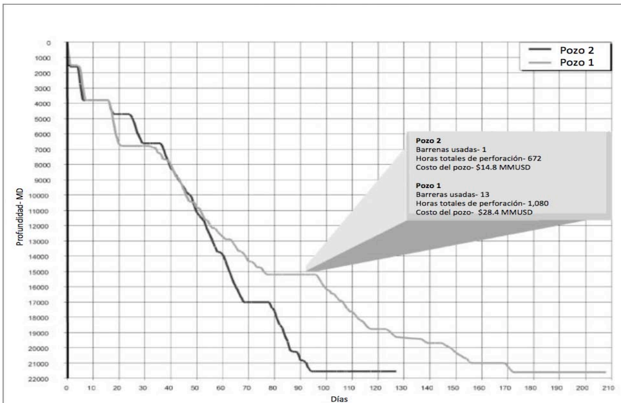
Figura 4.5 El gráfico muestra el progreso de la perforación de dos pozos en el Golfo de México. El Pozo 1 fue perforado utilizando una salmuera saturada mientras que el Pozo 2 mostró una gran ventaja, en cuanto a tiempo y costo, al ser perforado con un lodo SOBMs (Modificada de Meize et al., 2000).
