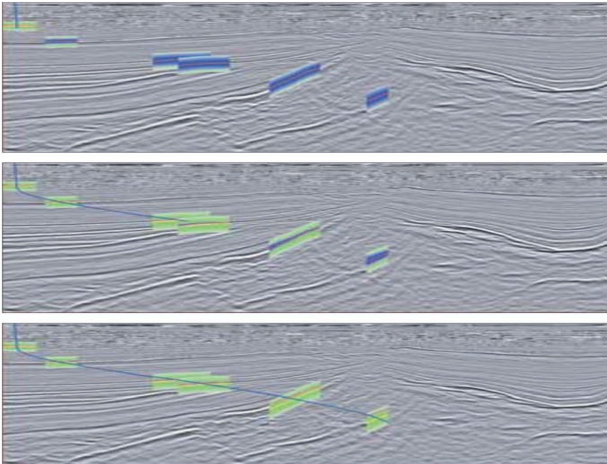
Figura 4.2 El mapa sísmico en tiempo real permite presentar información compleja como una trayectoria de pozo. Los datos en tiempo real se utilizan para actualizar los pronósticos de presión de poro y predecir los riesgos de perforación (Tomada de Aburto et al., 2008).
