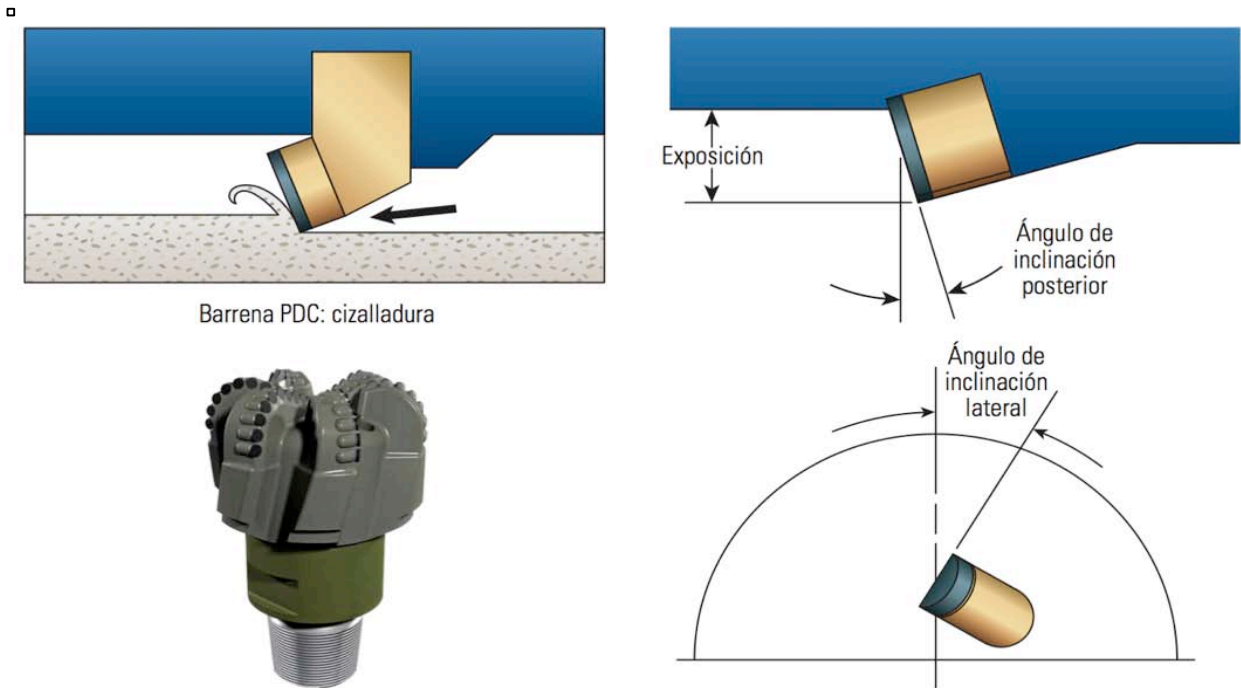
Figura 4.3 Las barrenas PDC son las más eficientes al perforar secciones salinas, debido a su acción de corte por cizalladura. El ángulo de inclinación posterior, la exposición de la herramienta de corte y el ángulo de inclinación lateral definen el grado de agresividad con que estas barrenas contactan la formación (Modificada de Aburto et al., 2008).
