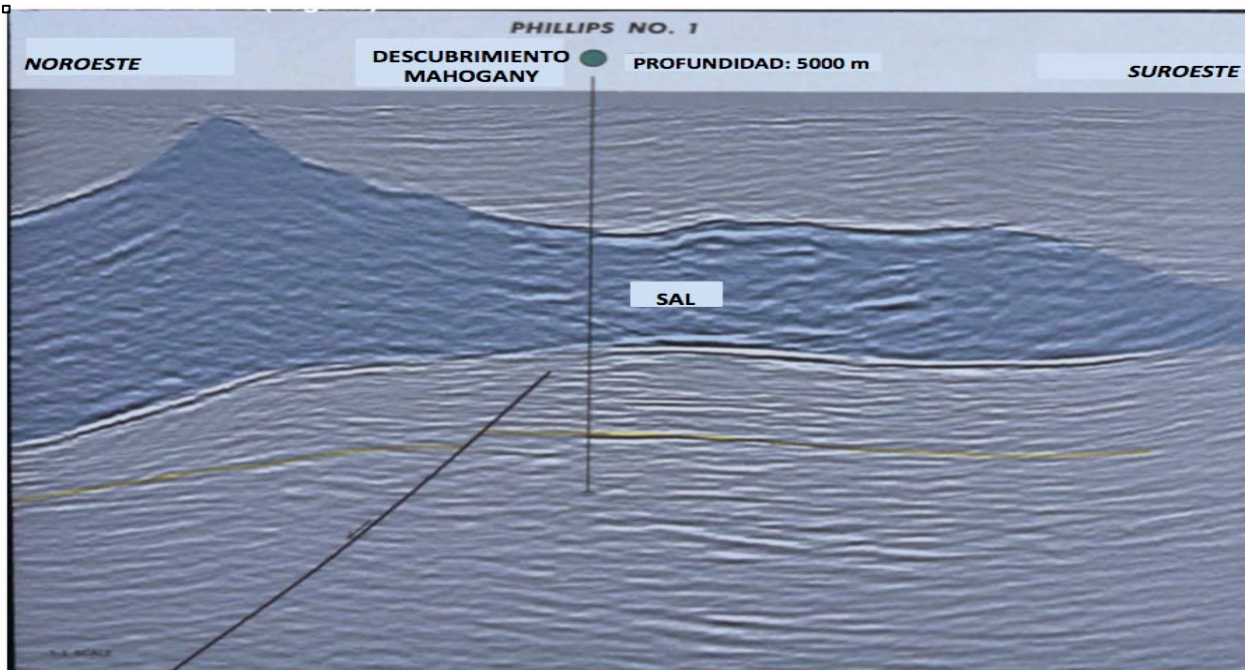
Figura 3.15 La base y la cima del canopy de sal se pueden apreciar en esta sección sísmica. La base se inclina hacia el noroeste (en dirección de la sal autóctona). También se puede apreciar claramente la falla que corta el anticlinal (Modificada de Harrison et al., 2010).
