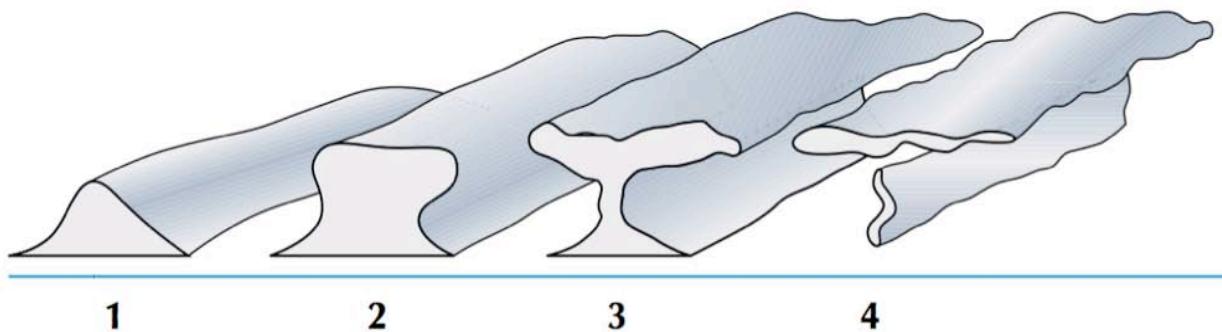
Figura 2.4 Evolución de las paredes de sal hasta formar toldos o canopies, los cuales pueden estar cubriendo zonas de acumulación de hidrocarburos (Modificada de Farmer et al., 1996).
