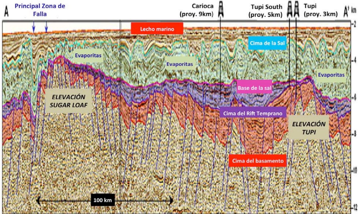
Figura 3.9 Sección transversal de la Elevación Exterior de la Cuenca Santos (OHSB) en la que se puede observar el campo presalino Tupi en el margen este de la estructura (la vista de planta de la OHSB se muestra en la Figura 3.8), (Modificada de Gomes et al., 2009).
