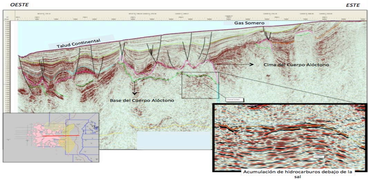
Figura 3.12 Sección sísmica regional de la Cuenca Essaouira en donde se puede apreciar la presencia de hidrocarburos debajo de una estructura de sal Alóctona. El mapa de la izquierda muestra la ubicación del estudio; las manchas rosas representan estructuras salinas someras (Modificada de Davison et al., 2010).
