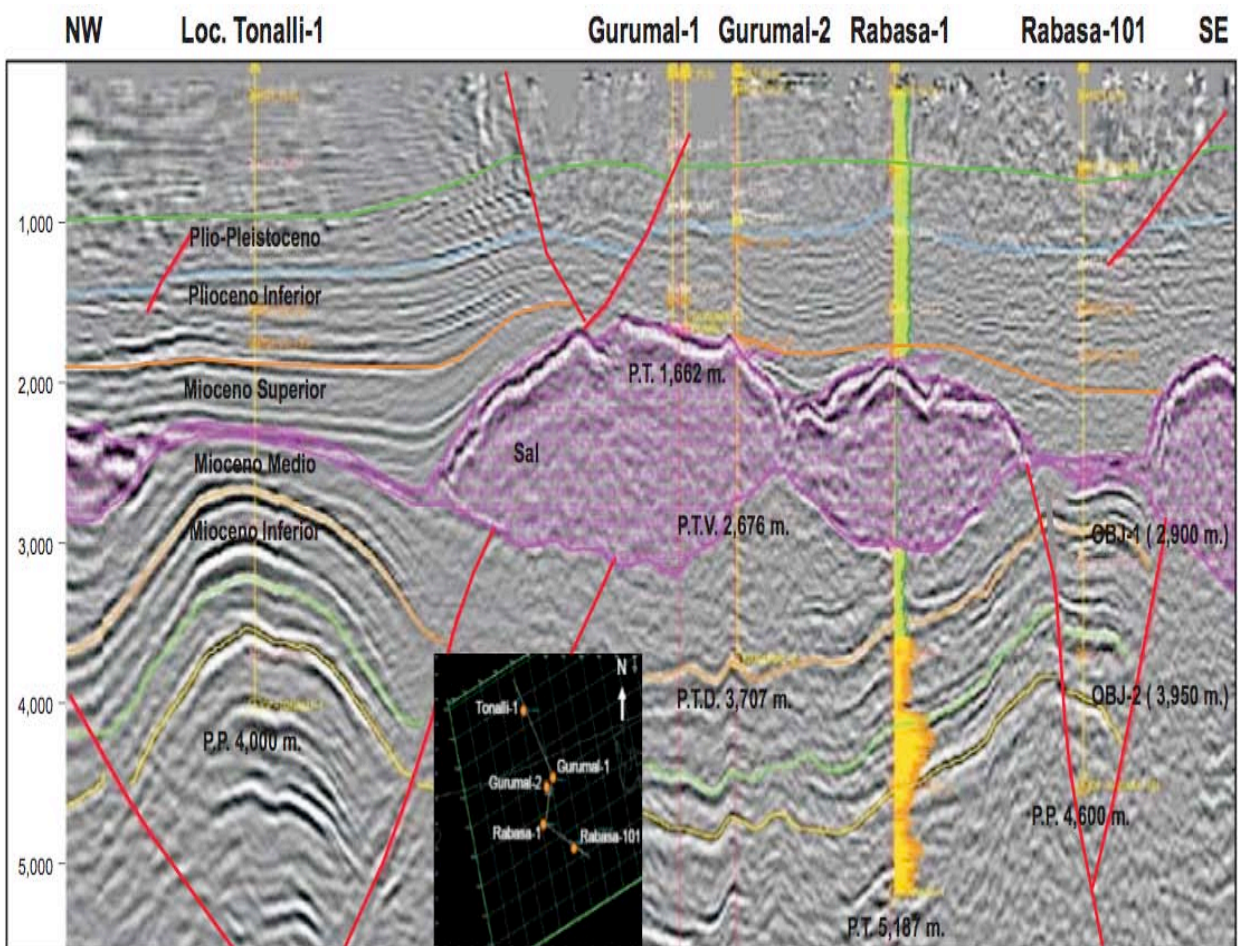
Figura 3.4 Línea sísmica que ilustra el comportamiento estructural del yacimiento (Tomada de PEMEX, 2009).
