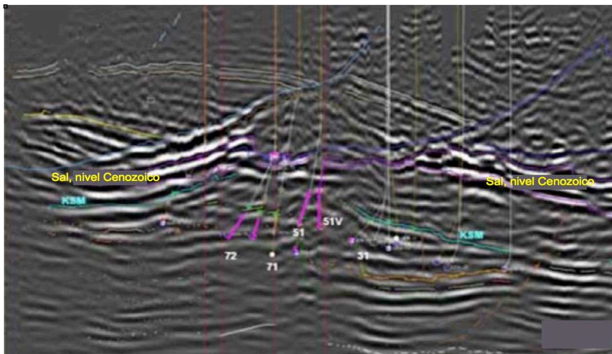
Figura 3.6 Línea sísmica que ilustra las secciones de sal intrusión en rocas del Cenozoico, cuya secuencia fue perforada por algunos pozos del Campo Sen. Se interpreta que los cuerpos de sal son lengüetas independientes sin ninguna correlación horizontal (Modificada de Baños y Sánchez, 2009).
