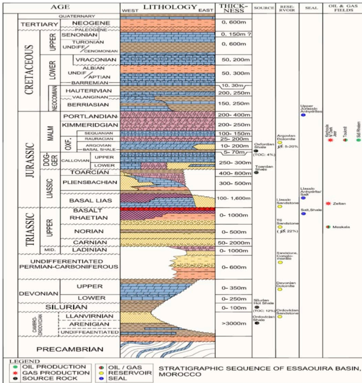
Figura 3.11 Columna estratigráfica de la Cuenca Essaouira (Tomada de PEL, 2010).
