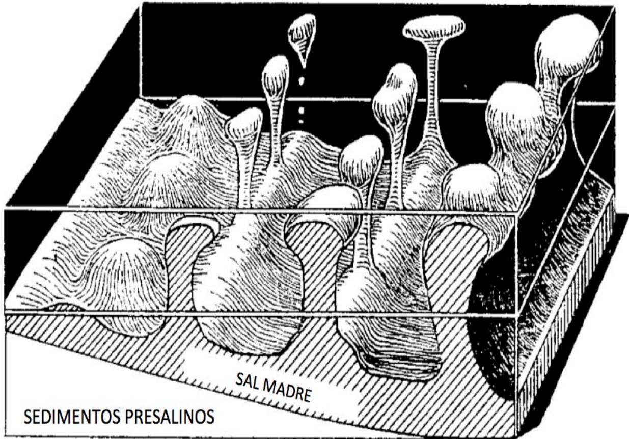
Figura 2.5 Troncos de sal. Pueden o no estar unidos a la sal madre por medio del vástago. Su desplazamiento horizontal puede dar origen a toldos y lengüetas (Modificada de Halbouty, 1979).
