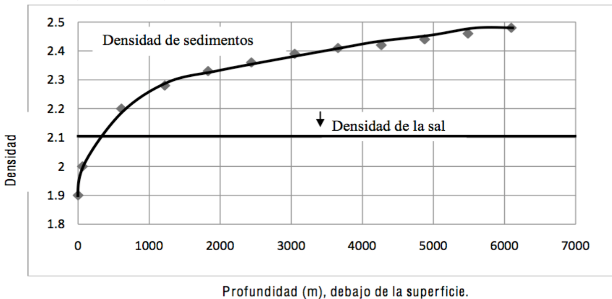
Figura 2.1 Esta gráfica muestra la variación de la densidad con respecto a la profundidad. Se aprecia como la densidad de los sedimentos varía fuertemente mientras que la de la sal permanece prácticamente constante (Tomada de Rojas, 2010).
