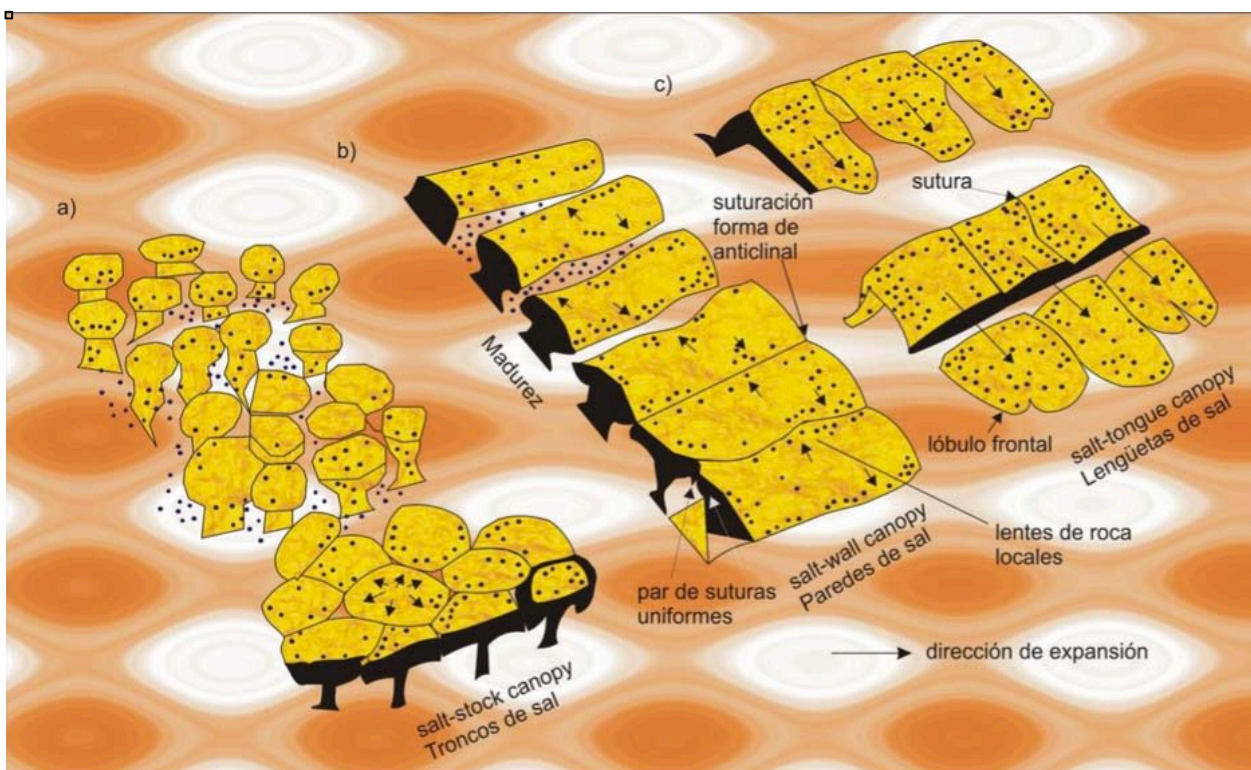
Figura 2.7 Se muestran los tipos principales de toldos o canopies de sal formados por la coalescencia de a) troncos de sal, b) paredes de sal y c) lengüetas de sal (Tomada de Rojas, 2010).
