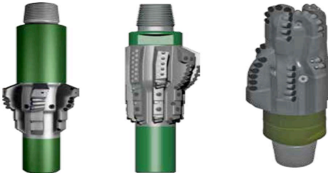
Figura 4.4 La figura muestra, de izquierda a derecha, un rectificador concéntrico, un rectificador excéntrico y una barrena bicéntrica. Estas herramientas permiten la implementación de la técnica EWD (Modificada de Schlumberger, 2013).
