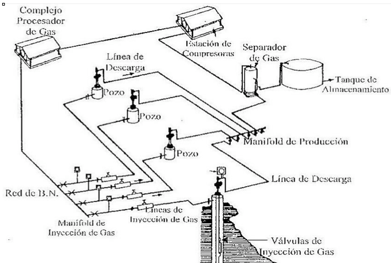
Figura 5.2 El esquema muestra los principales componentes de un sistema de bombeo neumático (Tomada de Téllez, 2014).
