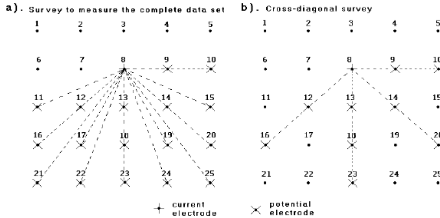
Figura 4 Electrodos en forma de rejilla cuadrada. Tomado de Loke y Barker 1996
