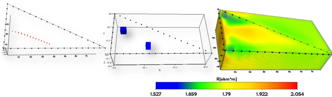
Figura 39 Modelo sintético del arreglo DD. Las anomalías que pasan cercanas a la distribución de puntos de atribucion serán detectadas, ya que esta distribución de puntos se localiza hacia el centro y a profundidad “iluminando” un area considerable.
