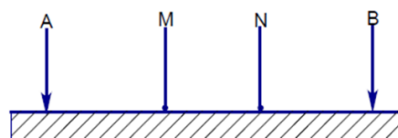
Figura 3. Electrodo de corriente A, B y electrodos de potencial M y N. Tomado de Iirte Sierra 2012
