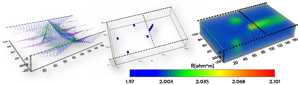
Figura 52. Respuesta para el arreglo de doble herradura con secuencias WS, ESQ, EQ y MA, para un modelo sintético con cuatro cubos de 4m^3 a z = -5m y una falla ubicada a z = -3m , todos con 1000[ohm*m] de resistividad en un medio de 100[ohm*m] .
