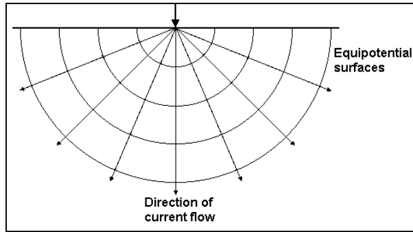
Figura 2. Flujo de corriente para una fuente puntual y la forma de distribución del potencial. Tomado de Loke (2010).
