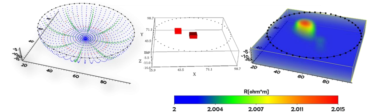
Figura 24 Respuesta de la combinación de todas las configuraciones para dos modelos sintéticos cúbicos, al centro en z=-2 y a un costado en z=-3 .
