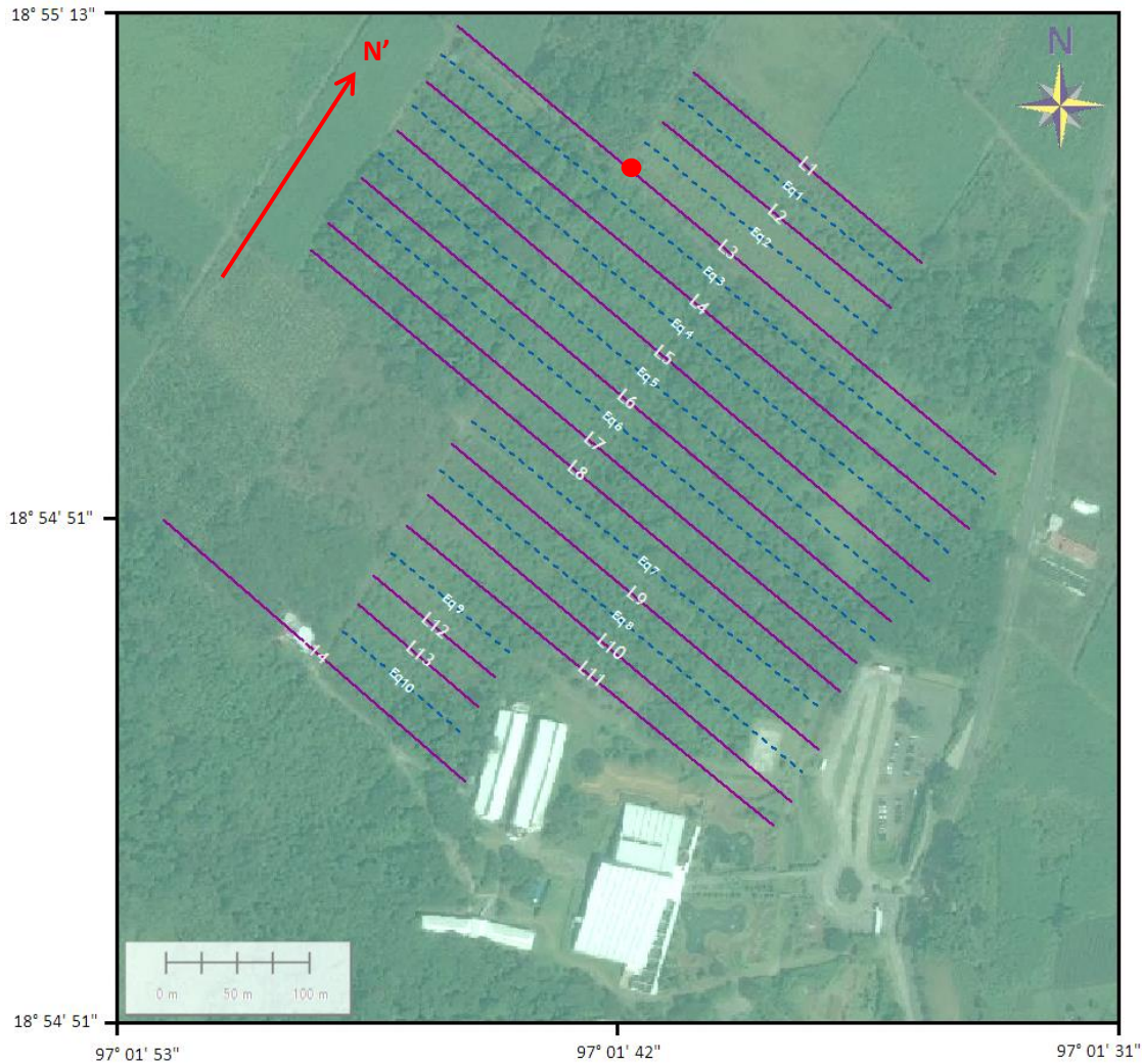
Figura 4.3.1 Modelo final de adquisición, donde las líneas continuas representan las adquiridas con arreglo W-S y las líneas punteadas son adquisición ecuatorial (Global Mapper).
