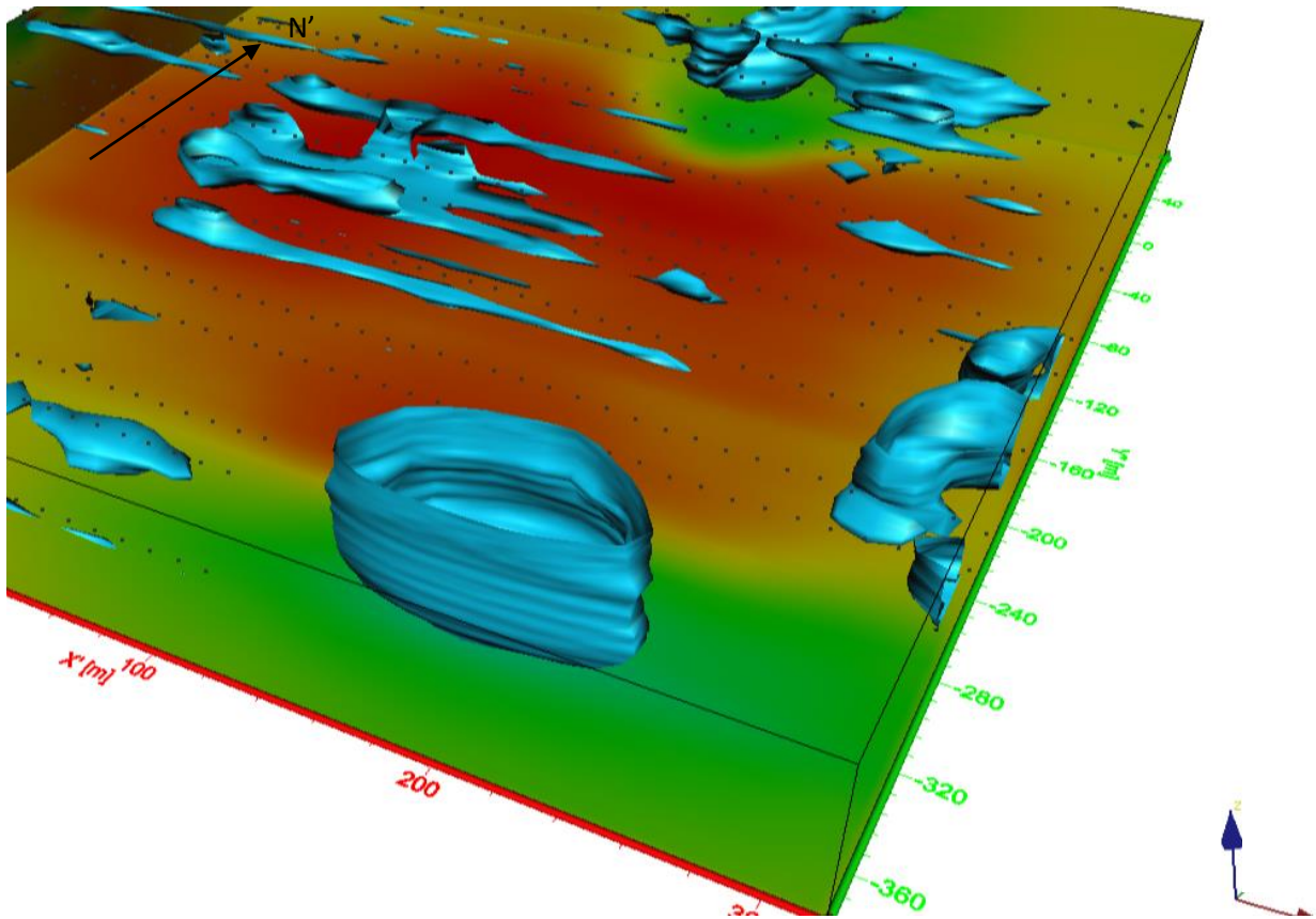
Figura 6.3.4. Superficie de Isovalor \rho = 60 [\Omega \cdot m]
