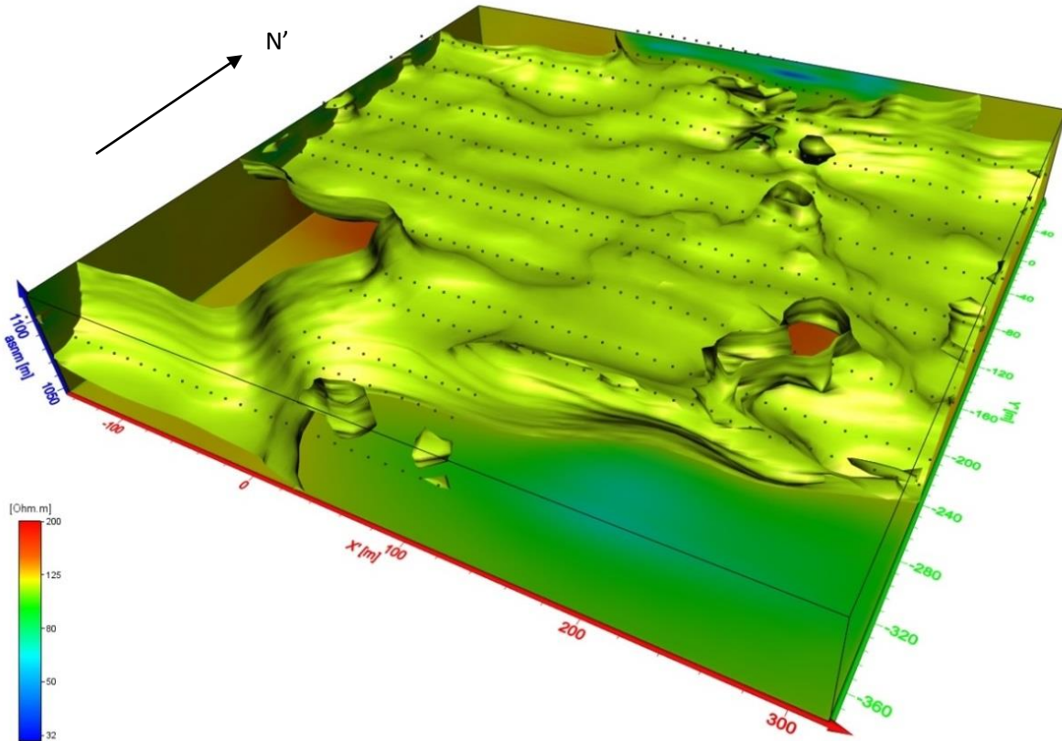
Figura 6.3.5. Superficie de Isovalor \rho = 95 [\Omega \cdot m]
