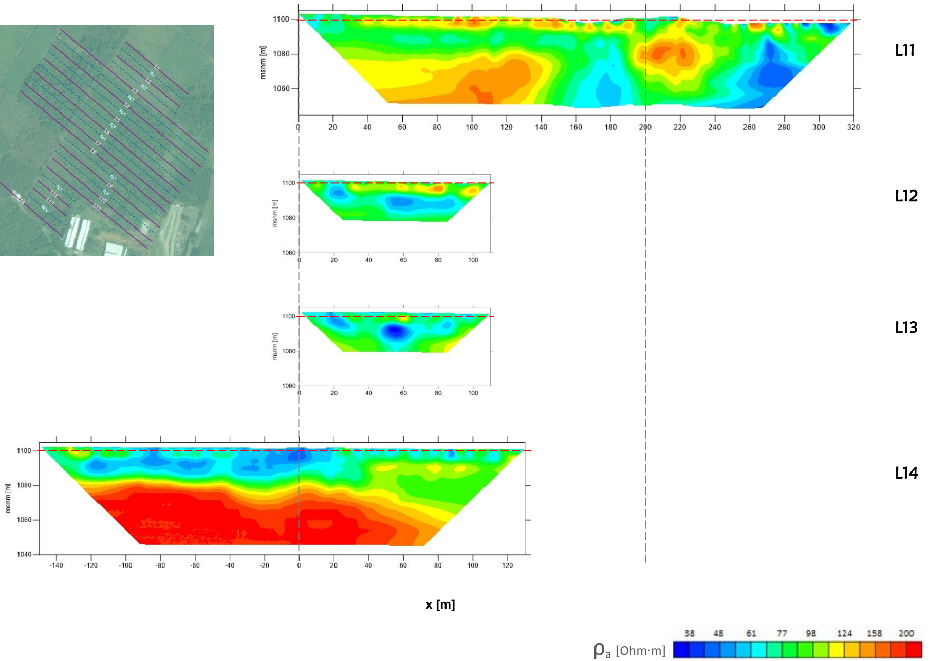
Figura 6.1.4 Resultados de la inversión de los perfiles L11, L12, L13 y L14.
