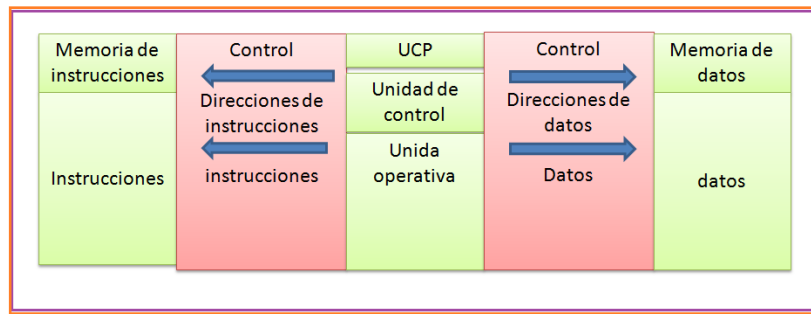
Fig.5.3.b. Arquitectura Harvard
