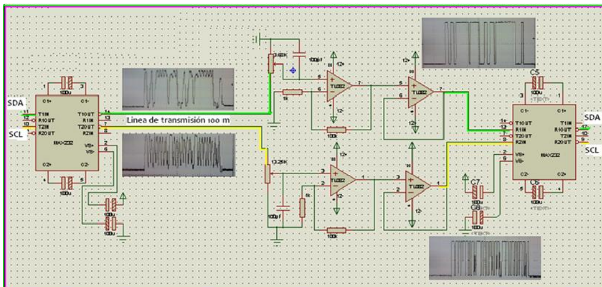
Fig. 4.3.i implementación de filtros paso- bajas y seguidores de voltaje con el TLo82 a la entrada del dispositivo esclavo
