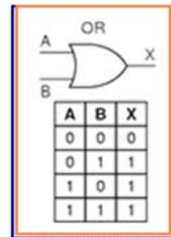
Fig. 5.2.c compuerta OR
