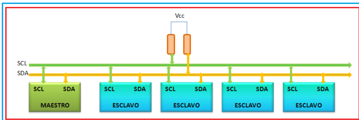
Fig. 2.1.a Estructura del BUS I2C
