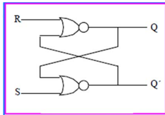
Fig. 5.2.1 Biestable S.R
