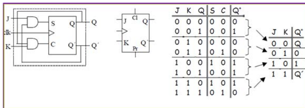
Fig. 5.2.v Biestable j-k sincronizado por flanco ascendente con entradas asincrónicas
