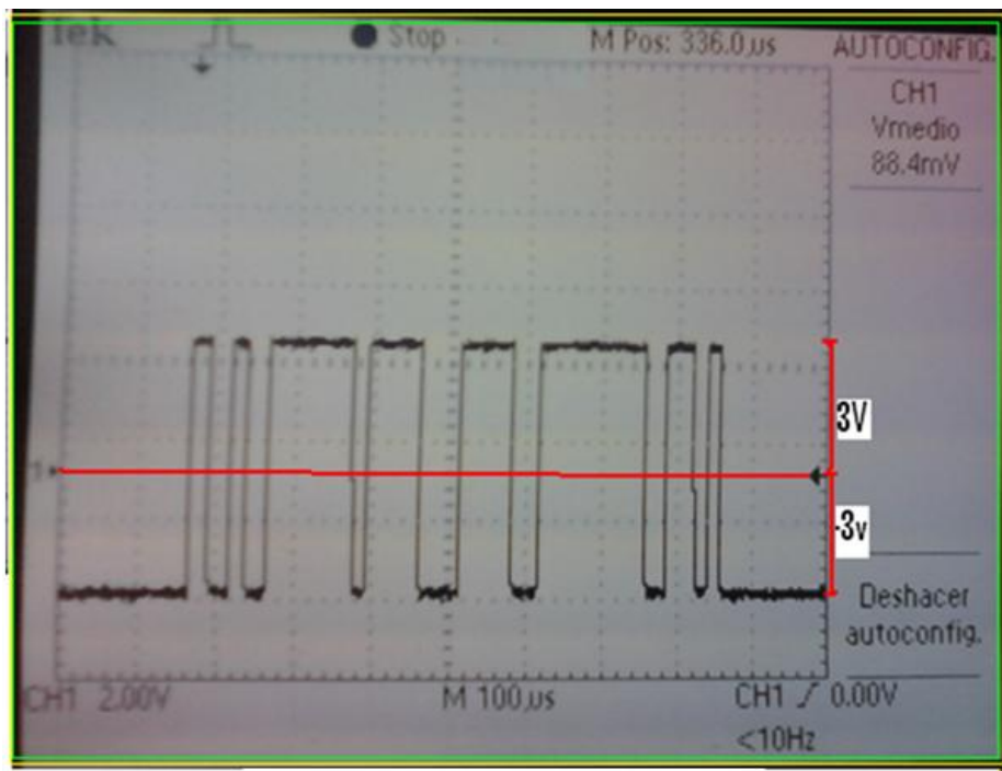
Fig. 4.3.c Señal SDA en nivel de voltaje RS232
