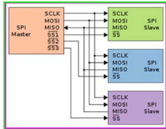
Fig. 1.2.a Comunicación SPI
