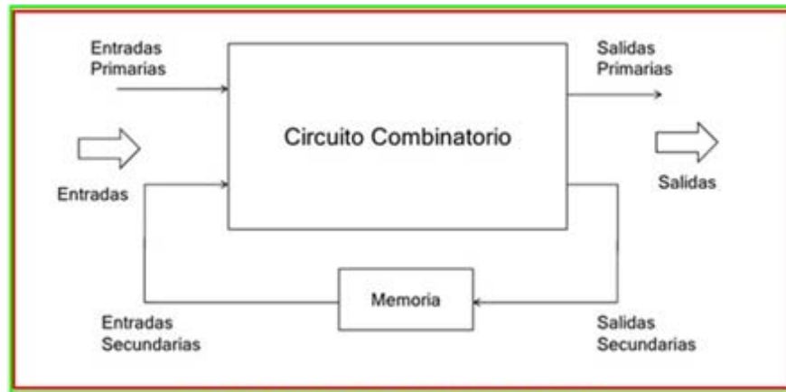
Fig. 5.2.h Modelo de circuito secuencial
