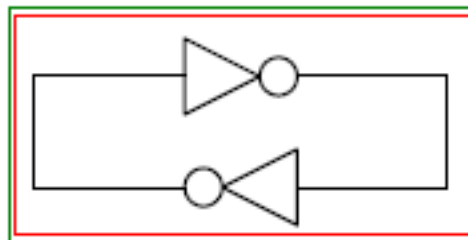
Fig. 5.2.i Biestable elemental
