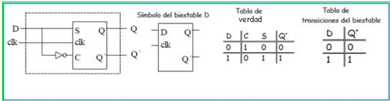
Fig. 5.2.w Biestable D sincronizado por nivel 1
