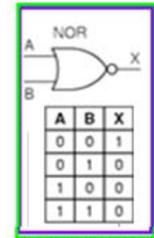
Fig. 5.2.g compuerta NOR
