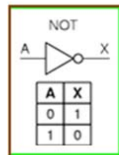
Fig. 5.2.d compuerta NOT
