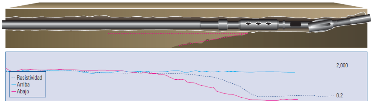
Figura.4.7: El mismo ejemplo de la Fig.4.6, pero disponiendo de mayor información. Las curvas azimutales permiten inferir que el pozo se aproxima a las lutitas por la parte inferior del pozo 39 .
