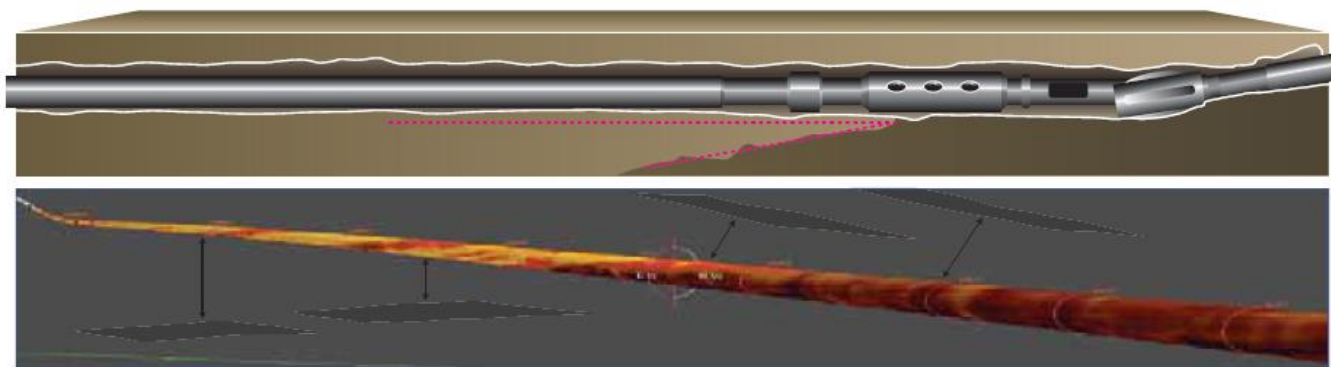
Figura.4.8: El pozo para calcular los echados, lo cual permite reprogramar la trayectoria del pozo para retornar al yacimiento. Mismo ejemplo de la Fig. 4.7, pero ahora incluyendo el uso de imágenes de la pared del pozo 40 .
