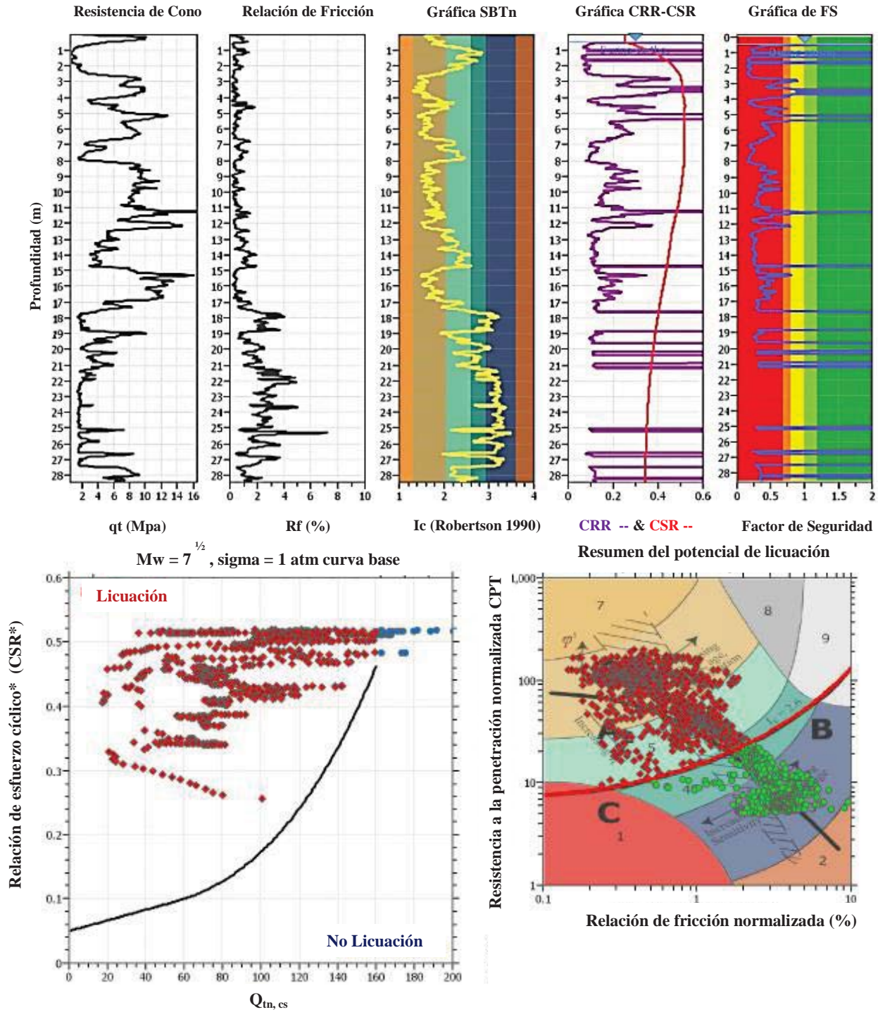
Figura 4.9. Resultados del análisis del potencial de licuación del CPT-SH4.
