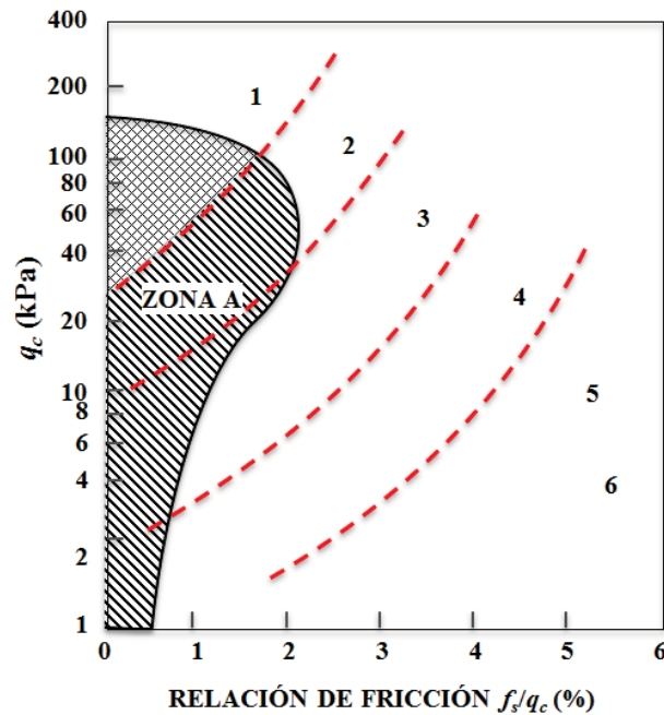
Figura 3.11. Determinación del potencial de licuación en función de la relación de fricción y q_c , (Robertson y Campanella, 1985).
