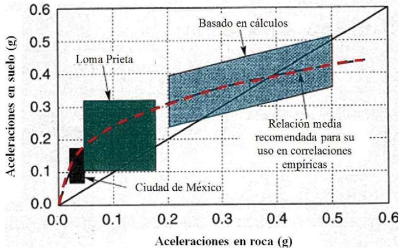
Figura 4.5 Curva desarrollada por Idriss para aproximar la relación entre la aceleración máxima en roca y suelo blando (tomado de Kramer, 1996).
