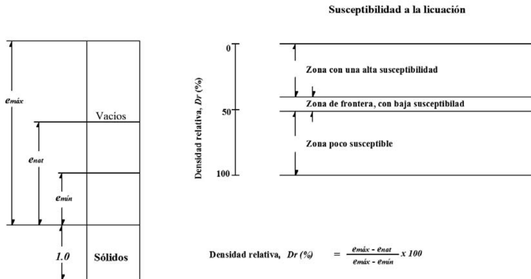
Figura 2.18. Concepto de densidad relativa (Henríquez, 2007).
