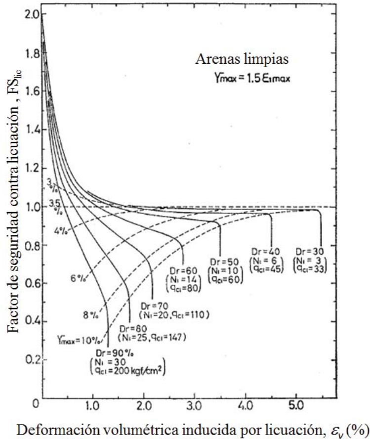
Figura 3.25. Carta para la deformación volumétrica en función del factor de seguridad (Ishihara y Yoshimine, 1992).
