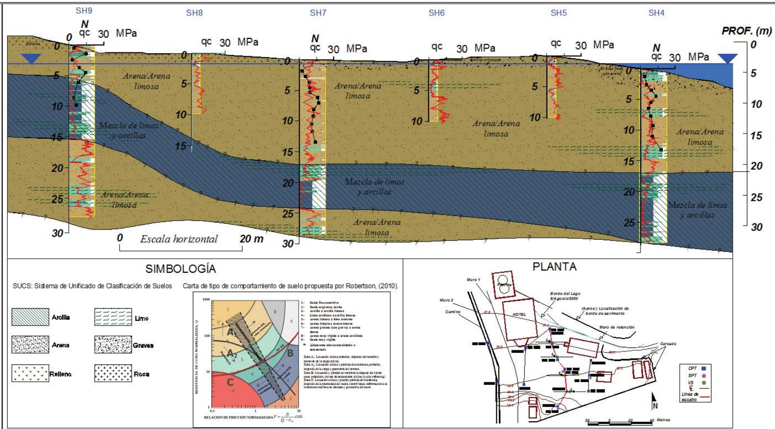
Figura 4.15. Perfil característico del suelo con base en los resultados de la prueba CPT.
