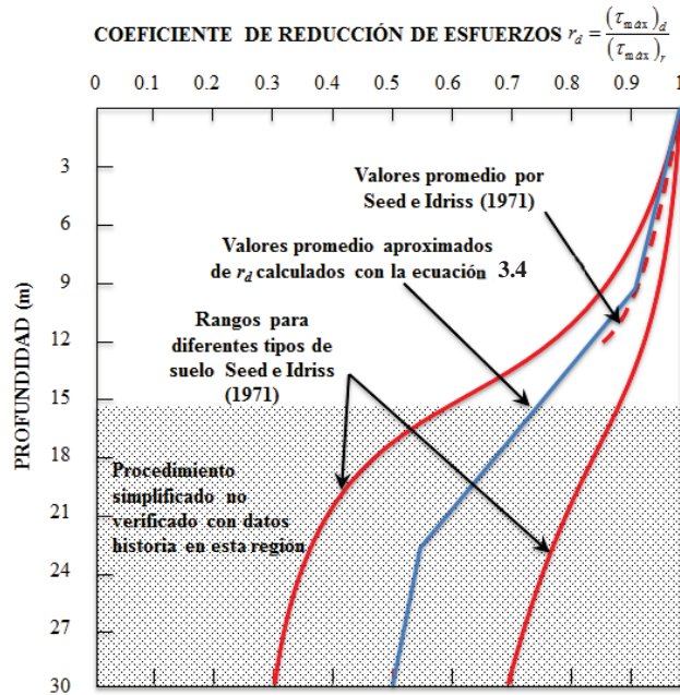
Figura 3.2. Curvas de valores de r_d contra profundidad (Youd et al. , 2001).
