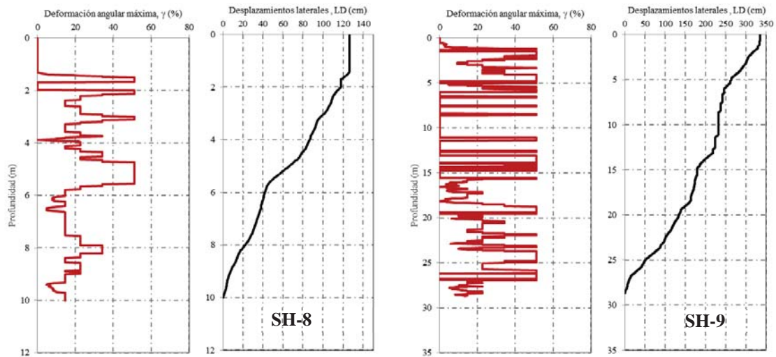
Figura 4.37. Desplazamientos laterales y deformaciones angulares máximas correspondientes a los sondeos SH-8 y SH-9.
