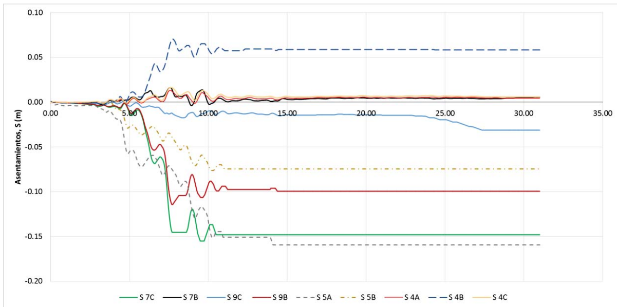
Figura 5.34 Asentamientos en función del tiempo
