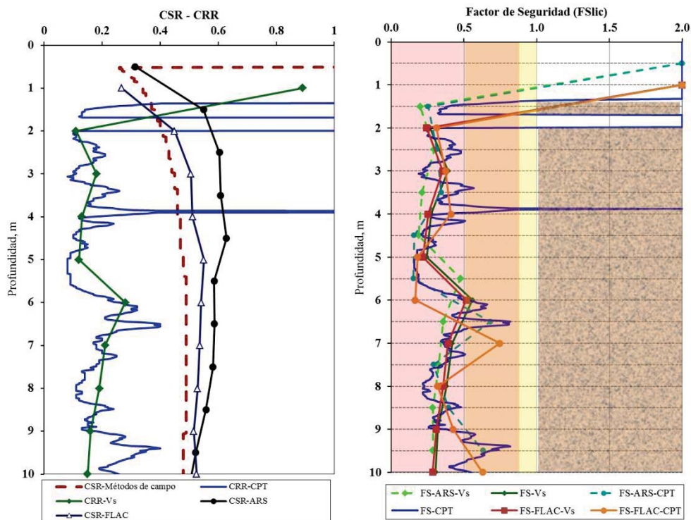
Figura 6.5. Comparación entre curvas de CSR-CRR y FS_{lic} determinadas por diferentes métodos y zonas potencialmente licuables del sondeo SH-8.
