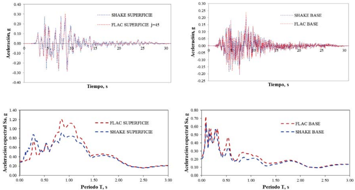
Figura 5.6. Calibración de los movimientos de campo libre, espectro de respuesta e historia de aceleraciones, correspondiente a los modelos SH-6 y SH-7.
