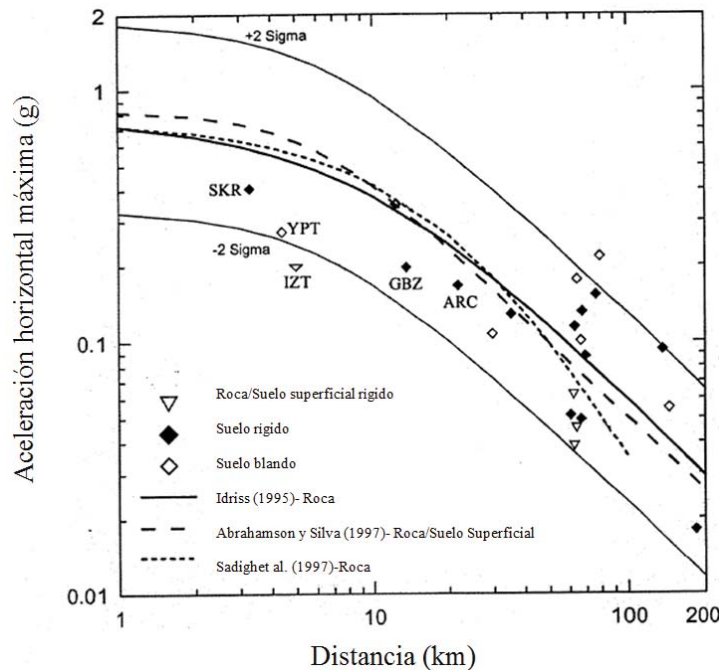
Figura 4.4. Comparación entre la media geométrica del registro de aceleración horizontal en las estaciones de sismos fuertes y las relaciones de atenuación propuestas por varios investigadores para magnitudes de M_w = 7.4 , (Bay y Cox, 2001).
