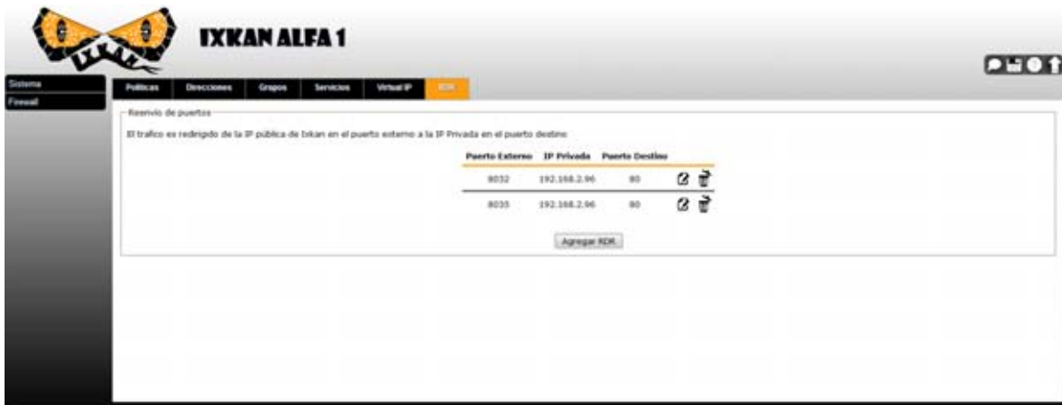
Figura 4-39 Redireccionamiento
