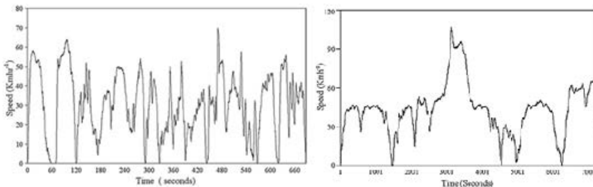
Figura 1.26. Ciclo de conducción para motocicletas, Edimburgo (EMDC).
