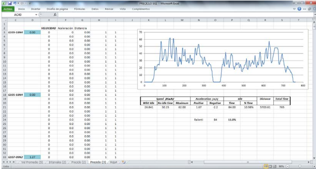
Figura 4.5. Preciclo de manejo sin alterar los valores de velocidad.
