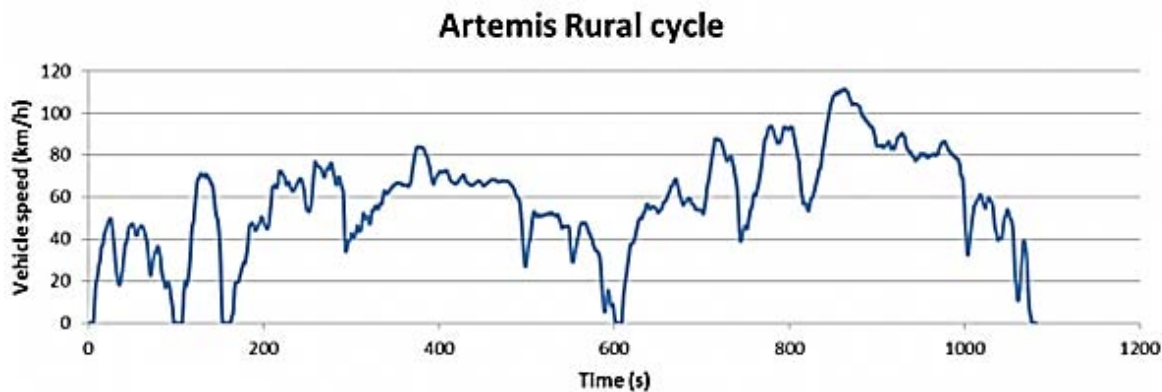
Figura 1.19. Ciclo de conducción Artemis, sección Rural.
