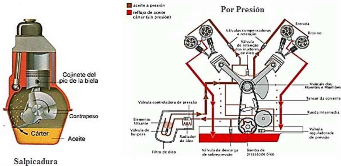
Figura 1.6. Sistemas de lubricación por Salpicadura (Izq.) y a Presión (Der.).
