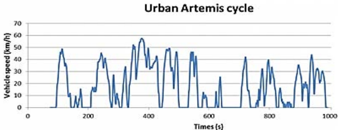
Figura 1.20. Ciclo de conducción Artemis, sección Urbana.
