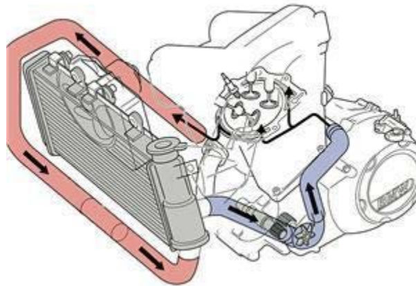
Figura 1.7. Sistema de enfriamiento por líquido.
