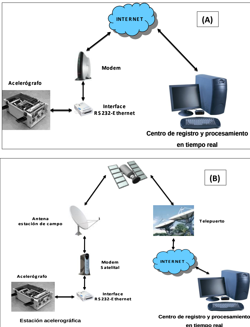
Figura 2.6 Sistema de comunicación empleada A) línea telefónica con servicio de tipo Infinitum y B) una antena satelital con servicio de Internet (ref. 43)
