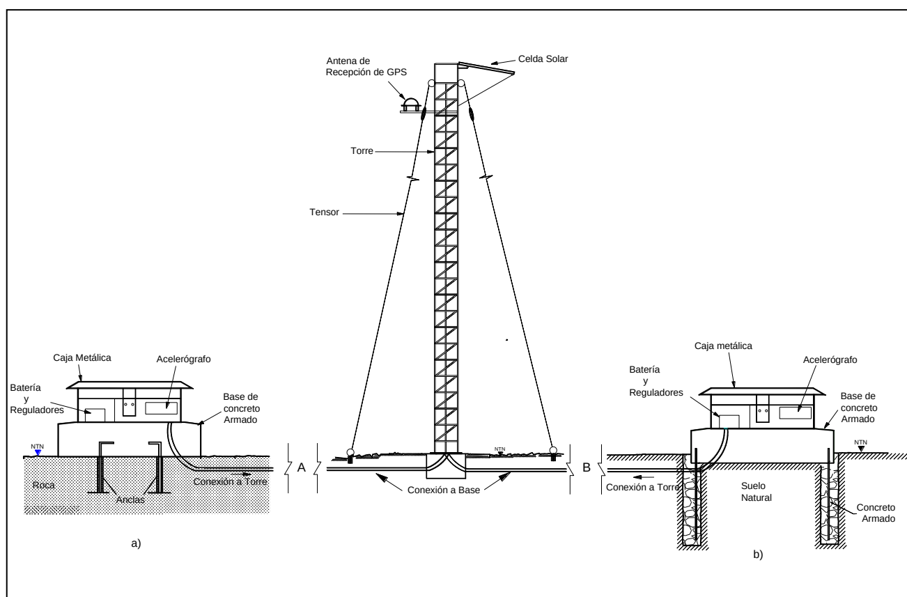
Figura 2.4 Estación Acelerográfica (ref. 40)
