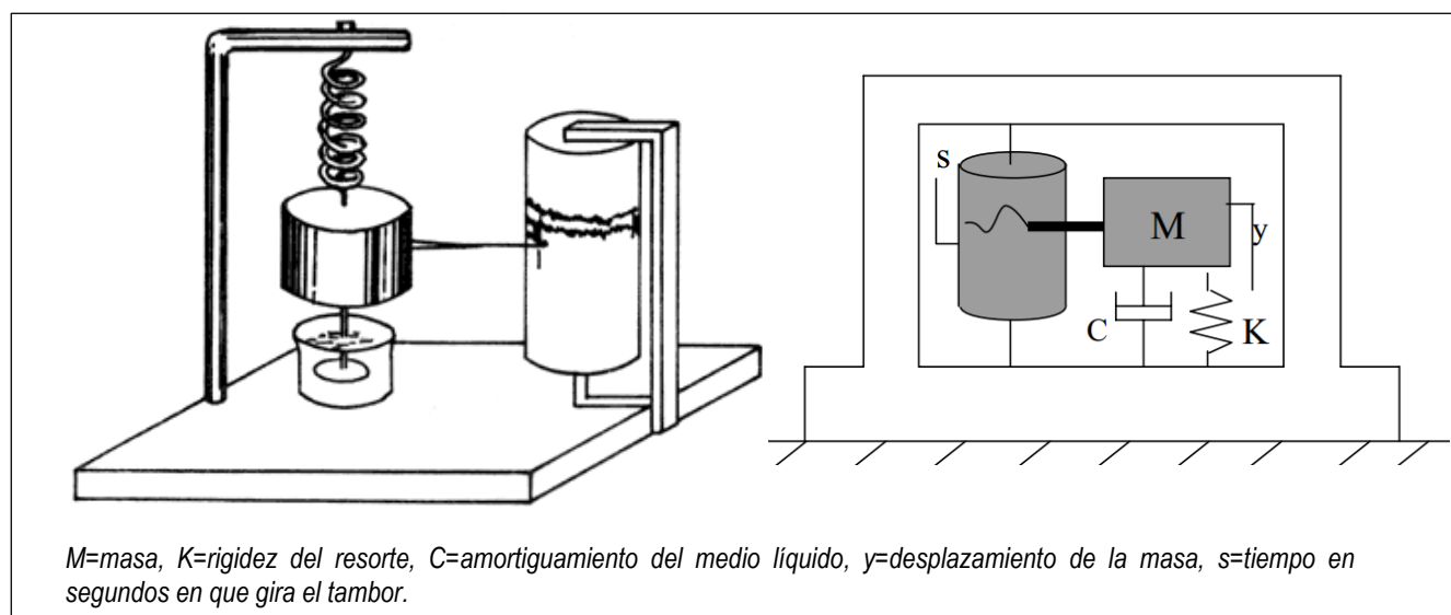
Figura 2.1 Principio del funcionamiento de un sismógrafo (ref. 36)
