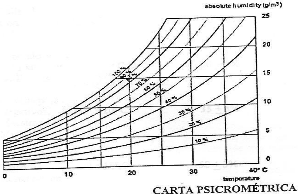
Figura 12. Carta psicrométrica.
