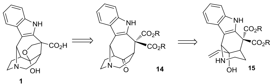
Esquema 4. Análisis retrosintético de Overman.
