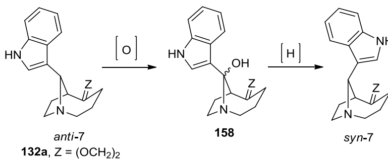
Esquema 60. Propuesta de síntesis del isómero syn - 132a vía un proceso de hidroxilación bencílica.
