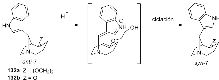
Esquema 54. Intento de síntesis del isómero syn de 132a vía una retro reacción de Mannich-reciclación.
