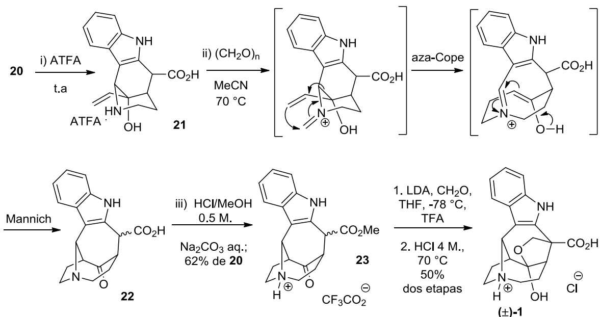
Esquema 6. Síntesis del éster pentacíclico 23 , mediante un proceso “one-pot” y culminación de la síntesis total de (±)-1 .
