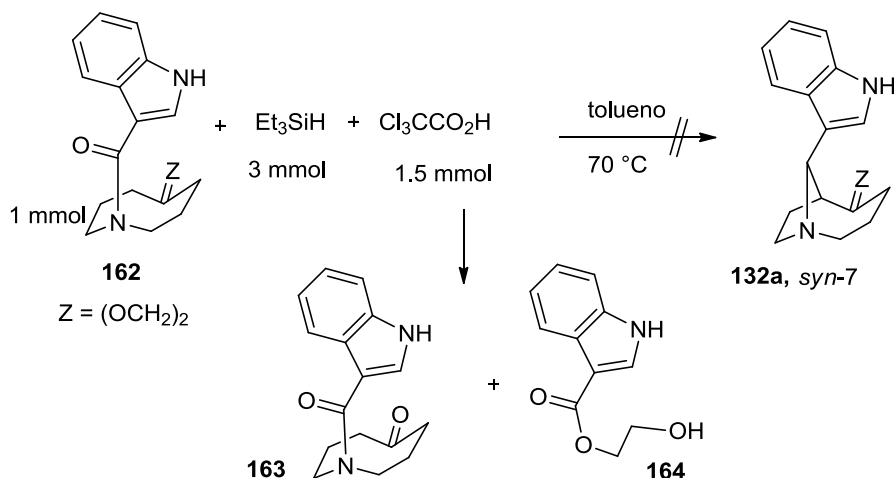
Esquema 63. Intento de síntesis del isómero syn -132a basado en los experimentos de Zhang.
