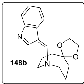
9-((3 H -indol-3-ilidene)metil)-1,4-dioxa-9-azaespiro[4.7]dodecano.
