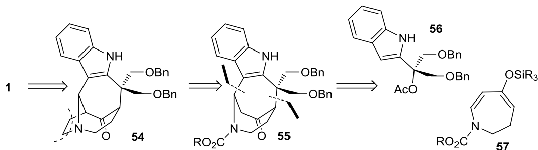
Esquema 16. Análisis retrosintético de Martin.
