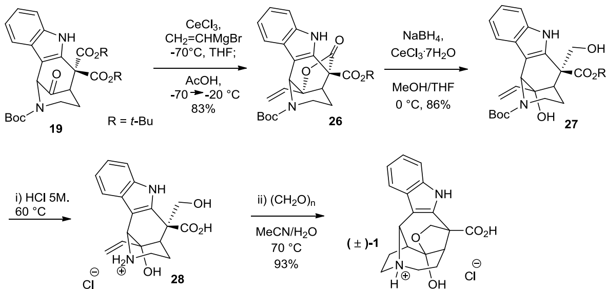
Esquema 8. Ruta sintética mejorada para la obtención de ( \pm )- 1 a partir de 19 .
