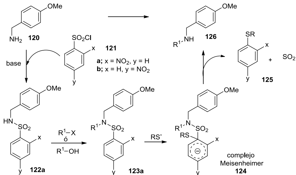
Esquema 34. Conversión de una amina primaria a su correspondiente amina secundaria usando la estrategia Ns. El método se ilustra con la p -metoxibencilamina como ejemplo.
