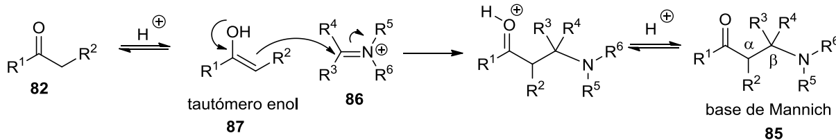
Esquema 25. Mecanismo de la reacción de Mannich en condiciones ácidas.
