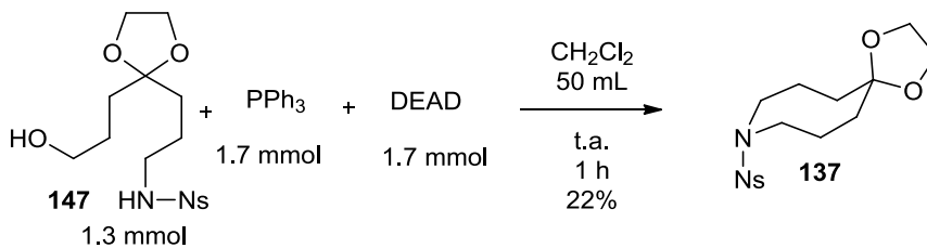
Esquema 48. Síntesis de 137 mediante una reacción de Mitsunobu intramolecular.
