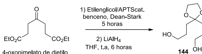
Esquema 45. Síntesis de la cadena dihidroxilada 144 .
