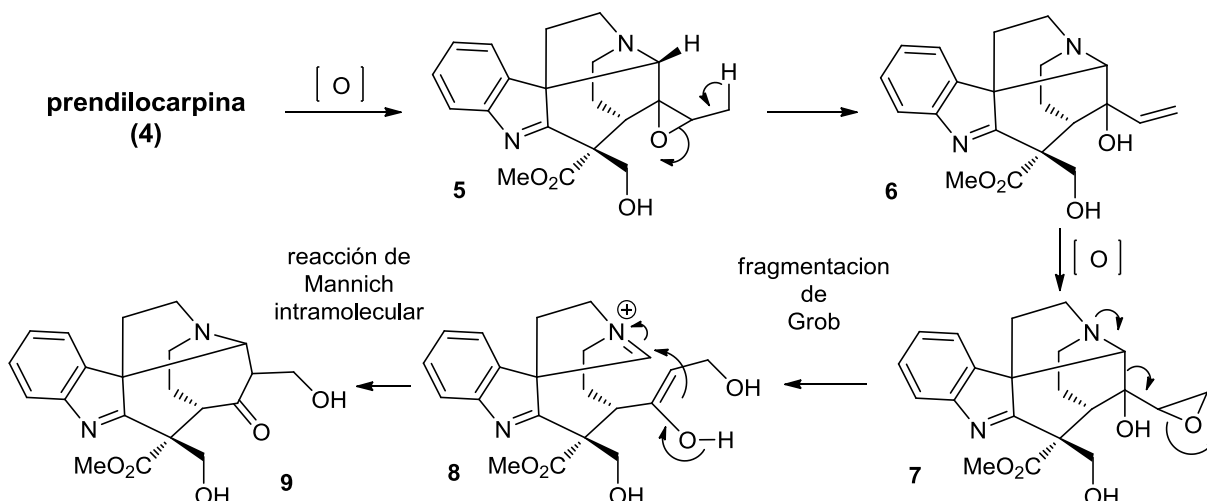
Esquema 2. Propuesta de biosíntesis para el ácido actinofílico a partir de la prenilocarpina.
