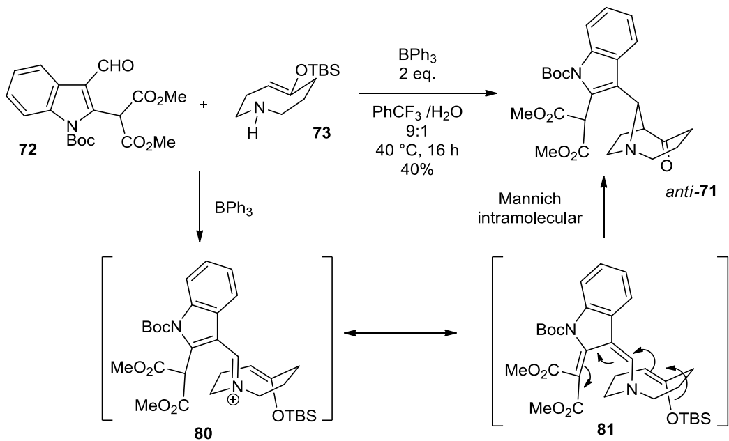
Esquema 23. Síntesis del 1- azabiciclo [4.2.1] nonano mediante una reacción de Mannich intramolecular mediada por un ácido de Lewis.
