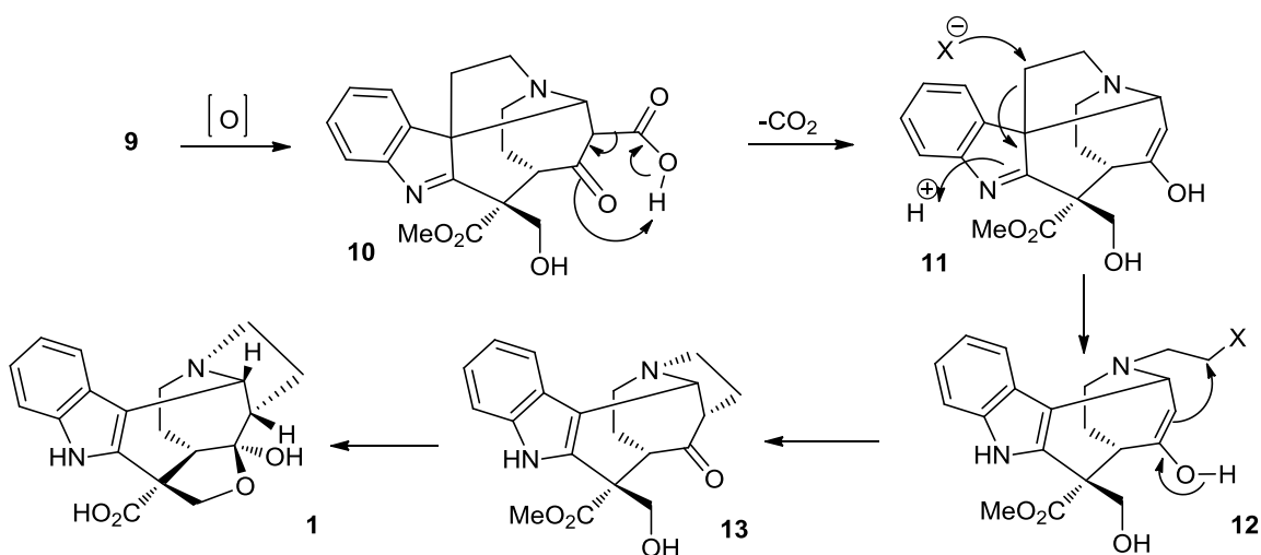
Esquema 3. Propuesta de biosíntesis del ácido actinofílico informada por Carroll y colaboradores.
