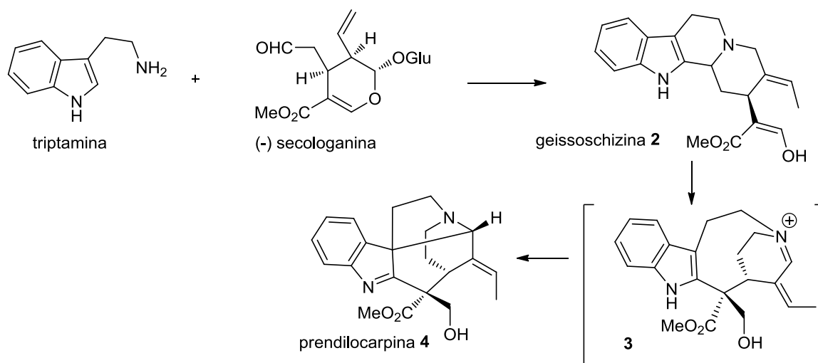
Esquema 1. Biosíntesis de la prenilocarpina a partir de triptamina y (-)-secologanina.
