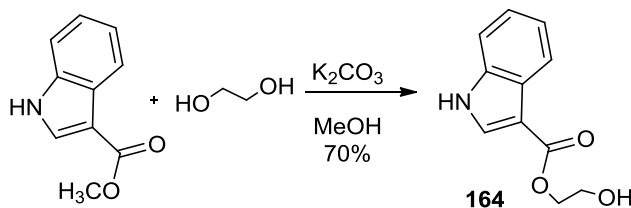
Esquema 64. Síntesis del indol-3-carboxilato de 2-hidroxietilo 164 mediante una reacción de transesterificación.
