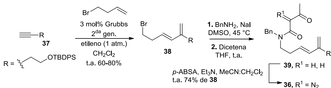
Esquema 11. Preparación de la diazoacetamida 36 .
