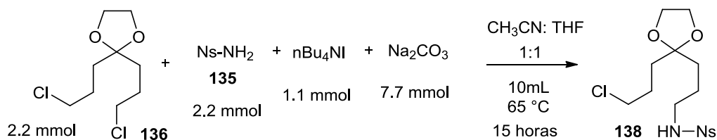
Esquema 42 . Preparación del producto monoalquilado 138 .
