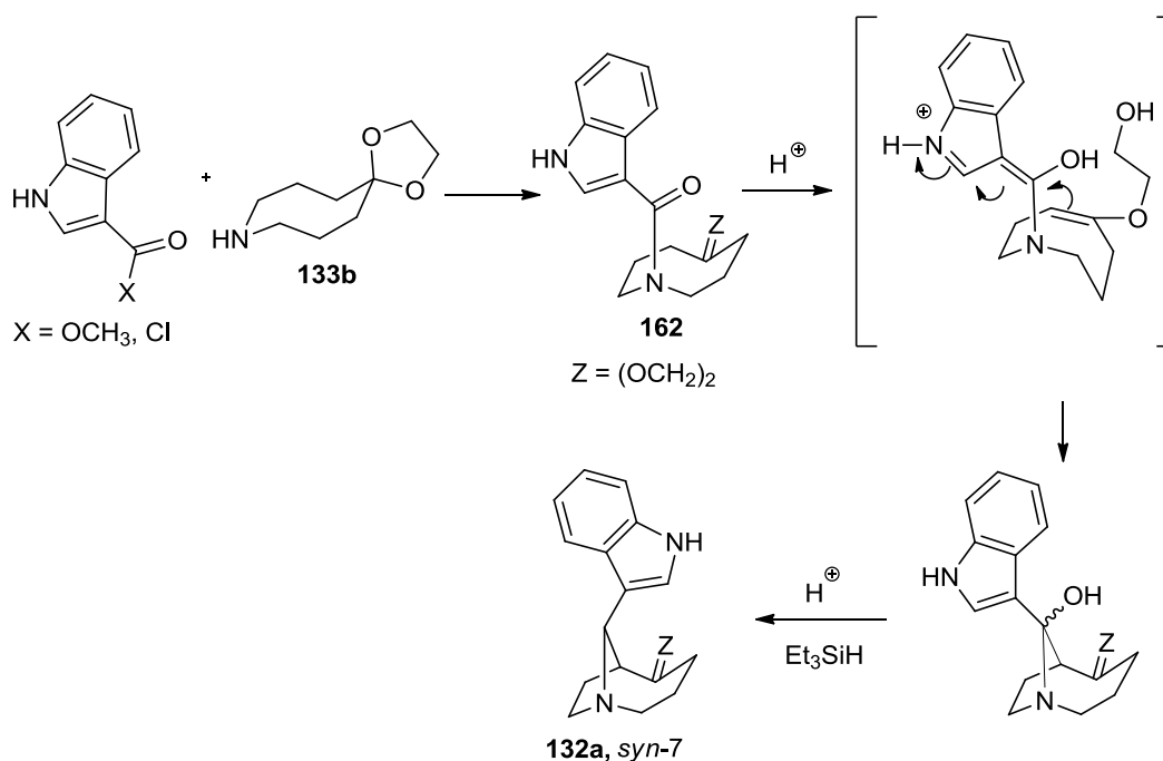
Esquema 62. Propuesta de síntesis tendiente a rectificar la estereoquímica de 132a .
