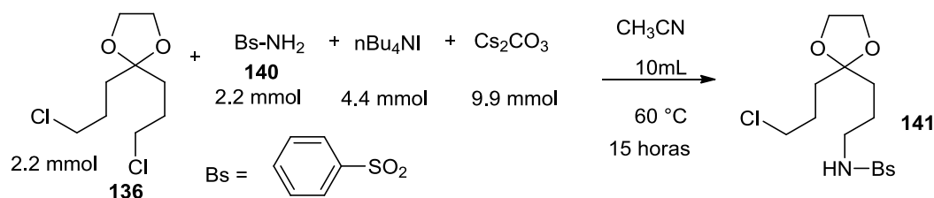
Esquema 39. Experimento para la obtención de 141 .
