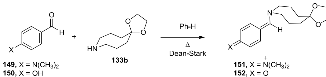
Esquema 53. Propuesta sintética para acceder a homoazafulvenos.
