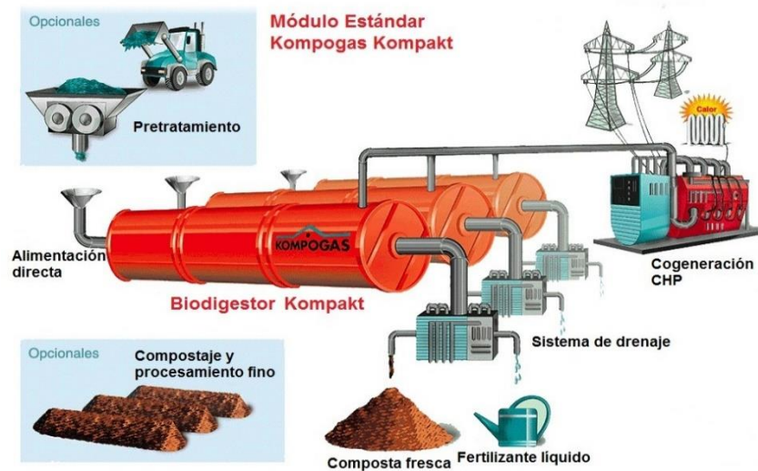
Proceso Kompogas
