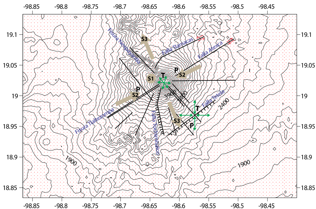
Figura 4.2 Modelo de esfuerzos debajo del volcán Popocatépetl, se muestran las fallas y fisuras propuestas por De Cserna et al. (1987) y SECOFI (1998). Los esfuerzos regionales (flechas grandes) S1, S2 y S3 corresponden al esfuerzo principal (vertical), intermedio y mínimo, respectivamente. Las flechas en verde representan los ejes de presión (P) y tensión (T) encontrados en el Popocatépetl por Arámbula-Mendoza et al. (2010).
