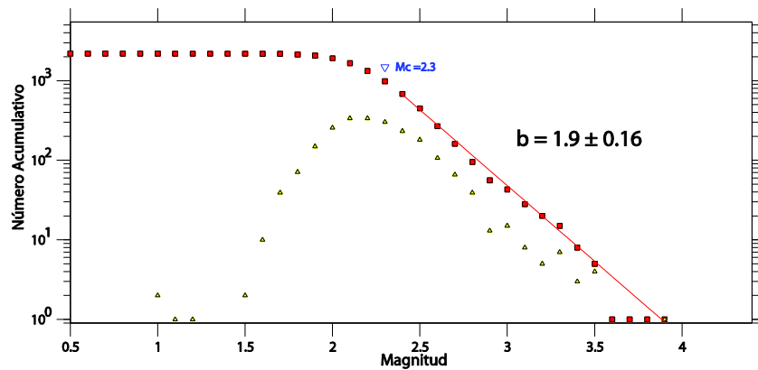
Figura 7. 1 Determinación del valor b para el catálogo general mediante el método de máxima verosimilitud. Los triángulos muestran la distribución frecuencia-magnitud para el número de eventos y los cuadros el número acumulativo. Se determinó una M_c = 2.3 , b = 1.9 y a = 6.14 .
