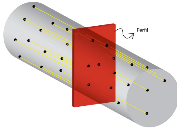
Figura 6. 6 Esquema de un volumen cilíndrico horizontal encerrando los sismos vulcano-tectónicos que son proyectados hacia la línea del perfil.
