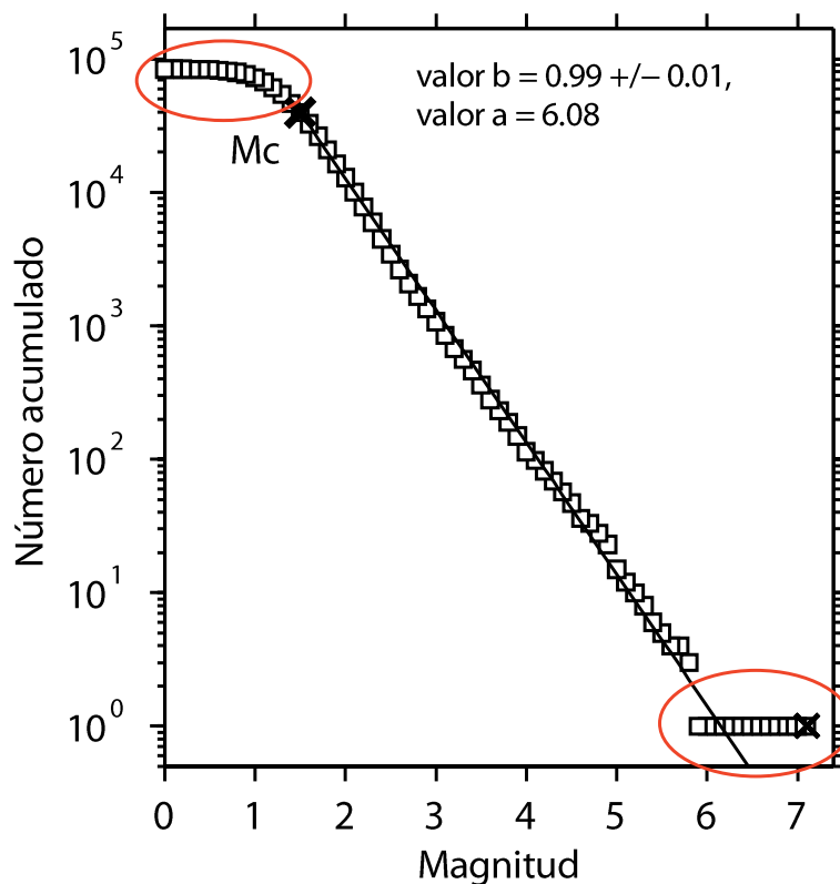
Figura 3.2 DFM para el catálogo sísmico del sur de California entre 1995 y 2000. Se puede observar las desviaciones del ajuste lineal ocasionadas por el rango de eventos menores a M_c detectados por la red (magnitudes pequeñas) y por el número reducido de todos los eventos grandes (Modificada de Wiemer y Wyss, 2002).
