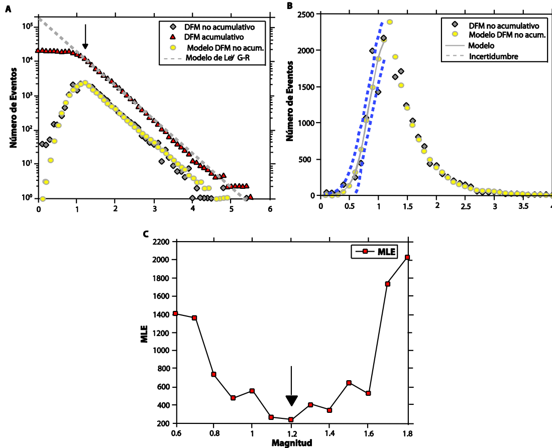
Figura 3.5 Método EMR aplicado a los datos del catálogo sísmico de la Red Sísmica del Norte de California (NCSN) entre 1998 y 2001: M_c = 1.2 , b = 0.98 , a = 5.25 , \mu = 0.73 , \sigma = 21 . (A) DFM acumulativa y no acumulativa en una escala logarítmica con la flecha indicando M_c . (B) Ajuste de la función de distribución acumulativa (CDF) normal (línea gris) a los datos con magnitud menor a M_c = 1.2 en una escala lineal. Se muestra la desviación estándar del modelo (línea punteada), los datos originales (diamantes) y la DFM no acumulativa del modelo EMR (círculos). (C) Elección del mejor modelo de las estimaciones por máxima verosimilitud (Modificada de Woessner y Wiemer, 2005).
