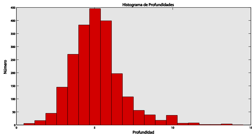
Figura 5. 6 Histograma de profundidades. Se puede observar que a 3km comienza a haber un gran aumento en la sismicidad hasta llegar a una media de 5 km donde vuelve a disminuir y encuentra los valores mínimos debajo de los 7 km.
