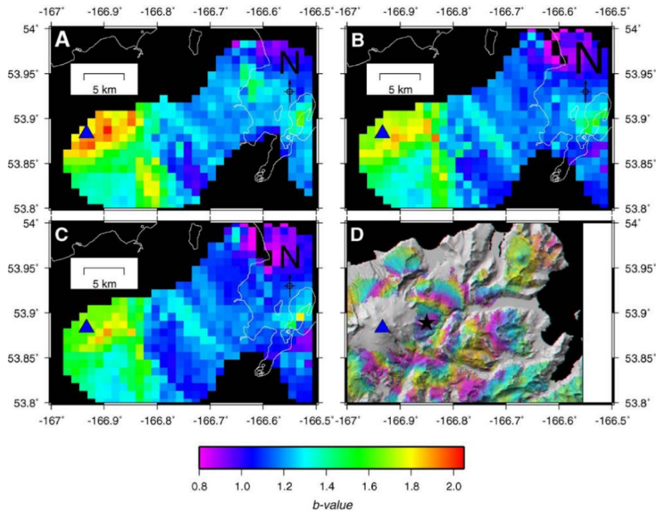
Figura 4. 10 Distribución espacial del valor b a: A) 4 km de profundidad, B) 6 km de profundidad y C) 7 km de profundidad. El triángulo azul muestra la ubicación del conducto principal. D) Resultados del trabajo de interferometría de Lu et al. (2002) mostrando el levantamiento observado en franjas de distintos colores (Bridges y Gao, 2006).
