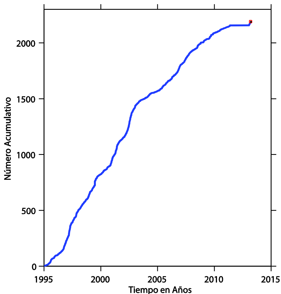
Figura 5.4 Serie de tiempo para el catálogo revisado. Se puede notar que el enjambre de 1996 ha desaparecido y el resto de la serie, excepto por el periodo 2011-2012, parece tener un incremento regular.
