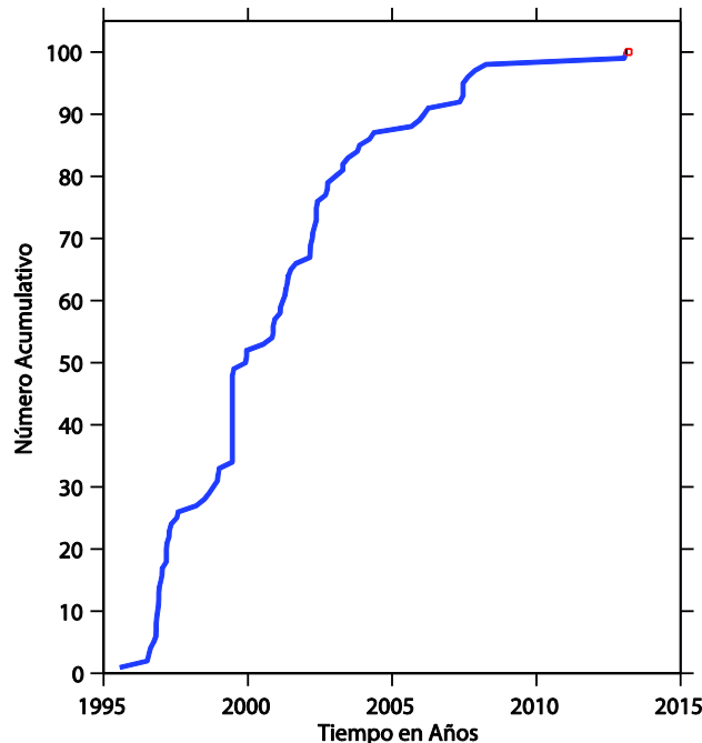
Figura 7.9 Serie de tiempo para uno de los volúmenes mapeados en la zona más somera al SE del cráter (3 en Figura 7.10 ). Se puede ver que los 100 eventos en este volumen se distribuyen en pequeños enjambres de eventos y por eso en lugar de tener una curva suave se tiene una forma de escalera.
