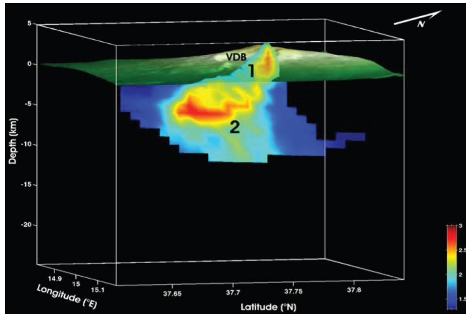
Figura 4.12 Imagen 3D de los valores b debajo del volcán Etna. Se eligió un mallado de 0.4 \text{ km} \times 0.4 \text{ km} \times 0.4 \text{ km} . La anomalía marcada como 2 se interpreta como una cámara magmática somera y la anomalía 1 como una reserva magmática que podría representar el conducto volcánico (Murru et al., 2007).
