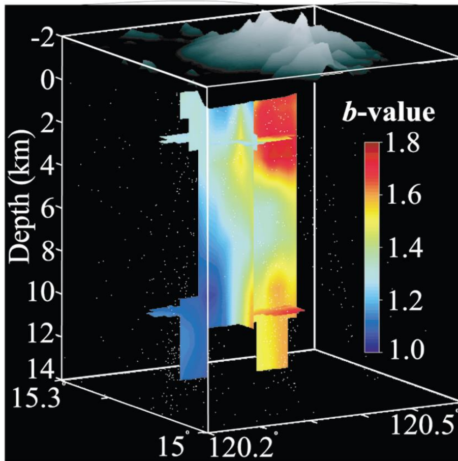
Figura 4.9 Modelo 3D del valor b debajo del volcán Pinatubo. Se muestran las dos anomalías de valor b relacionadas al sistema de salida de magma y una reserva magmática a profundidad ( > 8 km) (Sánchez et al., 2004).
