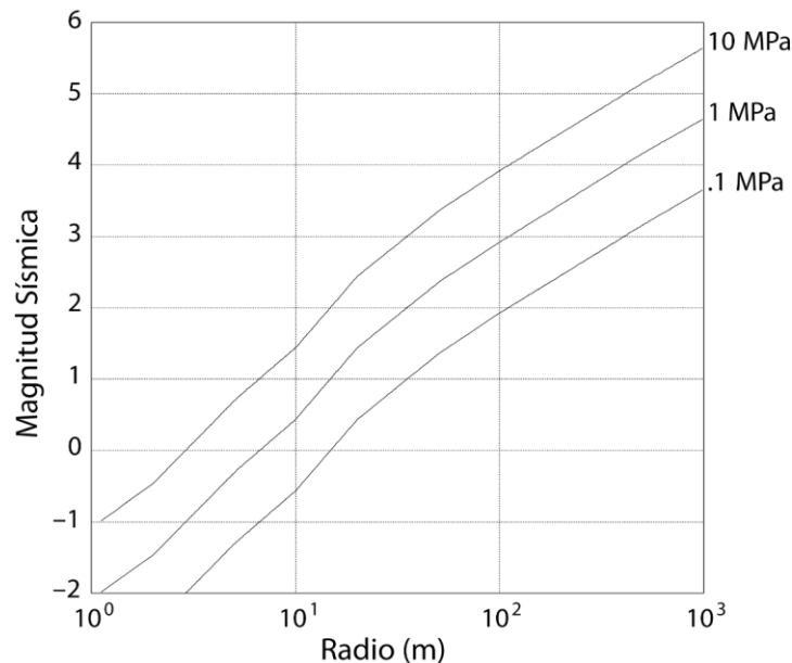
Figura 2. 14 Relación entre la magnitud de explosiones volcánicas y el radio del conducto observado. Las líneas muestran una relación teórica para las presiones de exceso iniciales asumidas en Megapascales (Modificada de Nishimura, 1998).
