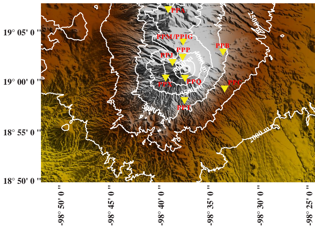
Figura 5.1 Red de monitoreo sísmico del volcán Popocatépetl.
