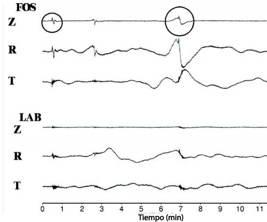
Figura 2.9 Señal de evento ULP registrada con un sismómetro de banda ancha Streckheisen STS2 en el volcán Stromboli. Se removió la respuesta del instrumento hasta 300 s y las trazas resultantes se integraron para reflejar el desplazamiento. Las primeras 3 trazas muestran las tres componentes de una estación situada a 400 m de la “chimenea” del volcán, mientras que las 3 trazas de abajo muestran las componentes de una estación situada a 1800 m del cráter. Como se puede observar las señales son claramente visibles solamente en el campo cercano. Los círculos muestran dos señales distintas de actividad estromboliana (Modificada de Wassermann, 2012).
