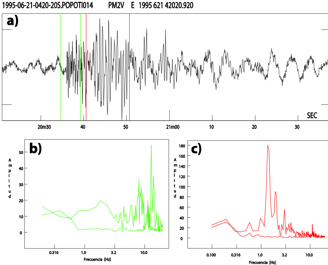
Figura 2.7 Ejemplo de un evento tipo híbrido en el volcán Popocatepetl. a) Sismograma de velocidades; b) Espectro de amplitud para el inicio de la señal (en verde) en donde se manifiestan las altas frecuencias atribuidas al fracturamiento de rocas; c) Espectro de amplitud para las fases de baja frecuencia (en rojo) asociadas al movimiento de fluidos.
