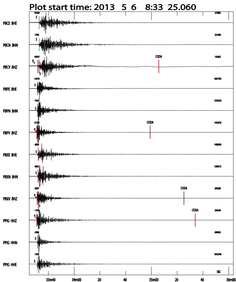
Figura 6.2 Picado de fases para un evento vulcano-tectónico registrado en el volcán Popocatépetl. La fecha y hora se muestran en la parte superior.
