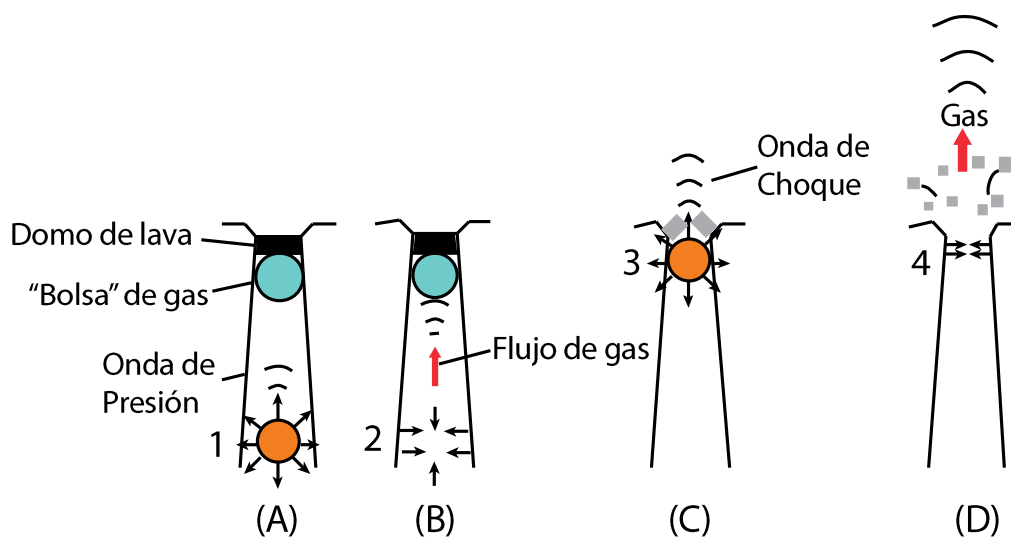
Figura 2. 12 (A) Ocurre una expansión isotrópica a profundidad (2 km en este ejemplo). Después se genera una onda de presión y se propaga a través del conducto hacia el cráter. (B) Se genera una contracción cilíndrica por el decremento de presión en la región de la fuente debido al escape de gases hacia arriba. (C) Expansión de la bolsa de gas debajo del domo de lava por el excitamiento producido por la onda de presión que se propaga desde una fuente a profundidad. Al mismo tiempo, una onda de choque es eyectada del cráter. (D) Se liberan los gases de la parte alta del conducto y comienza una contracción horizontal entre 1 y 2 s después del comienzo de la expansión (Modificada de Tameguri et al., 2002).
