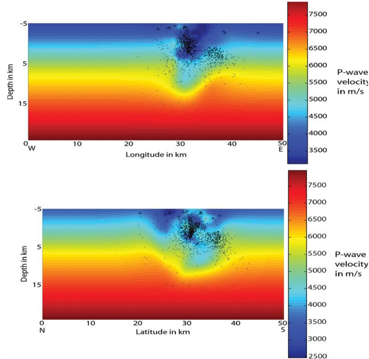
Figura 4.3 Modelos de velocidad de onda P. Los puntos negros indican los hipocentros de los sismos y los triángulos las ubicaciones de las estaciones sísmicas. El origen está ubicado en 19.3°N, 98.9°W y las profundidades están referenciadas al nivel del mar (Berger et al., 2011).
