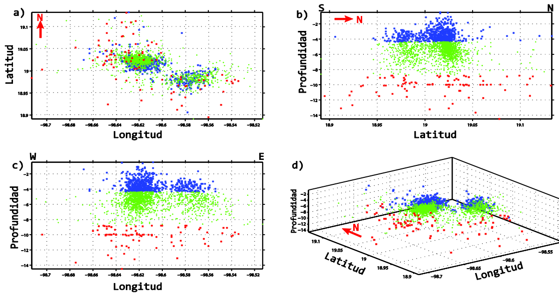
Figura 5.7 Distribución espacial de la sismicidad debajo del volcán Popocatepetl. El color azul muestra los eventos a profundidades z < 4.3\text{km} ; el color verde indica eventos con 4.3 < z < 8.7 ; el color rojo indica eventos cuya profundidad es z > 8.7 . a) Mapa de la sismicidad. b) Perfil S-N. c) Perfil W-E. d) Distribución tridimensional de los sismos.
