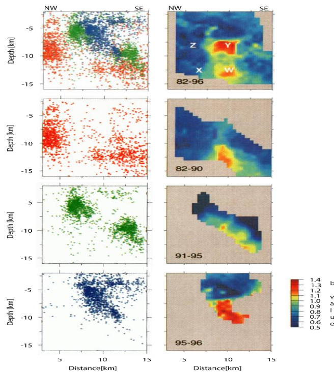
Figura 4.7 Secciones transversales paralelas al rumbo de la actividad sísmica fuera de la costa de Izu, Japón. A la izquierda se muestran los hipocentros y a la derecha los valores b para los diferentes enjambres (Wyss et al., 1997).
