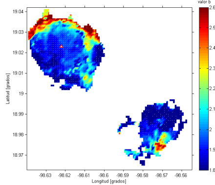
Figura 7.4 Mapa de valores b debajo del volcán Popocatépetl.
