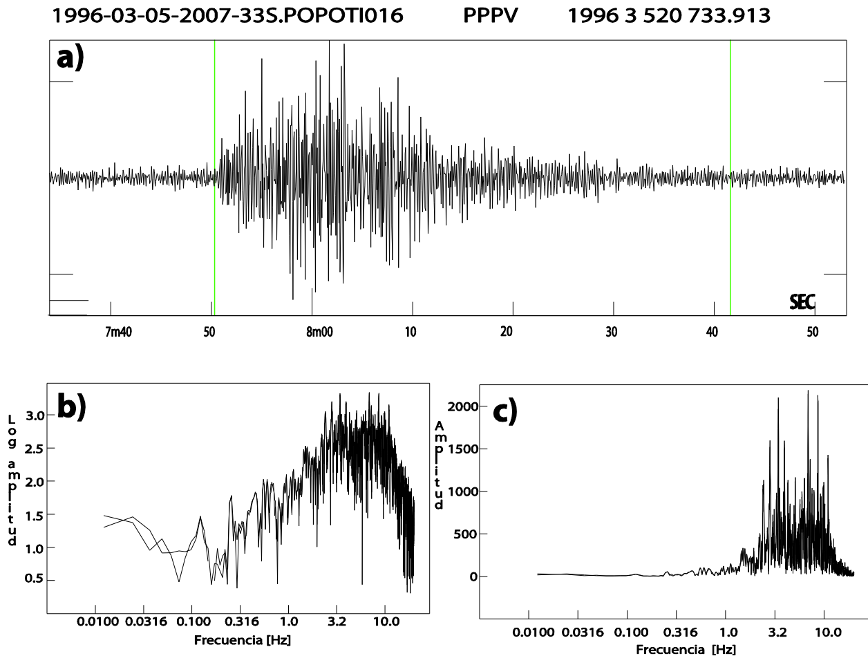
Figura 2. 2 Ejemplo de un evento vulcano-tectónico tipo B en el volcán Popocatépetl. a) Sismograma de velocidades; b) Espectro de log-amplitud; c) Espectro de amplitud. Las líneas en verde indican el segmento de traza para el cual se calculó los espectros y tanto la fecha como la hora del evento se muestra en la parte superior izquierda.
