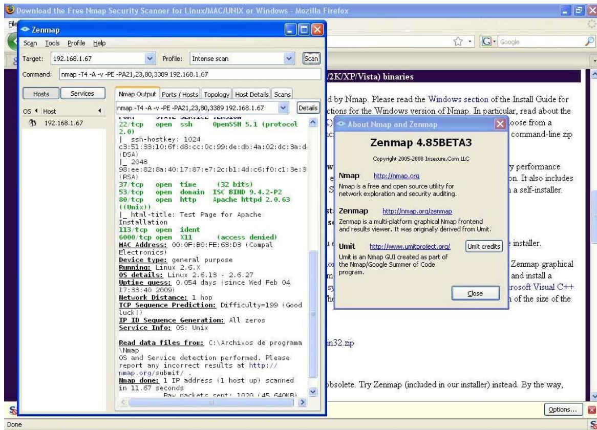
Figura 4.1 Zenmap es la versión gráfica de Nmap, en este caso es ejecutado en un sistema Windows
