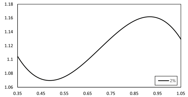
Figura 6.4.6: Valores de R_{\Omega} para una distorsión del 2%
