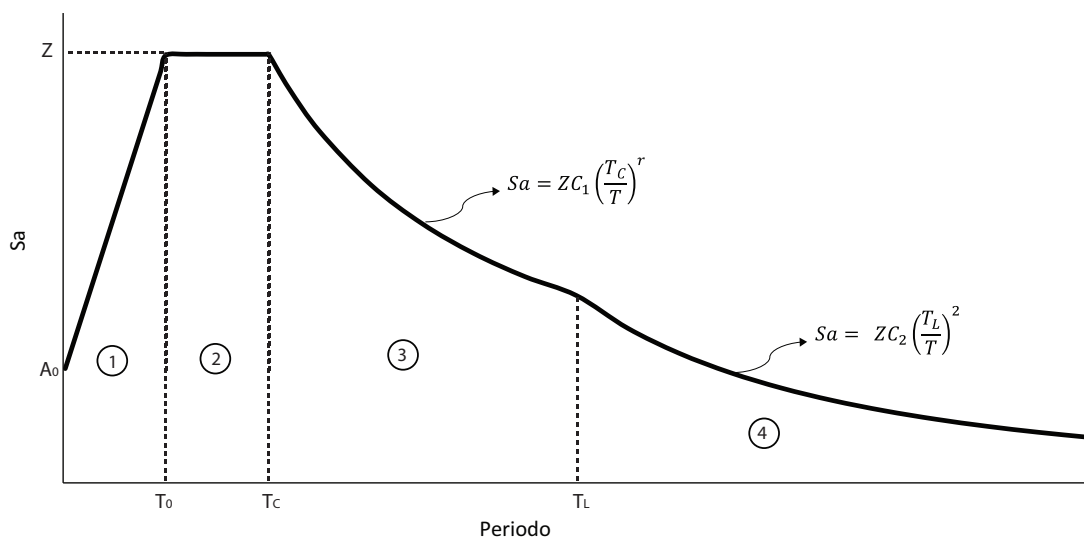
Figura 6.4.1: Espectro de diseño propuesto
