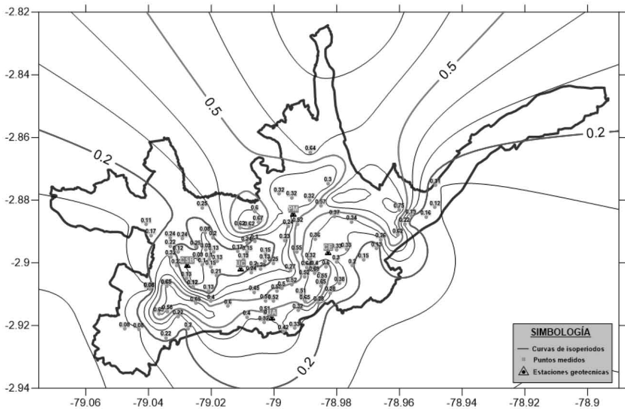
Figura 5.3.2: Curvas de isoperíodos. Puntos utilizados de estudio de Encalada (2000)
