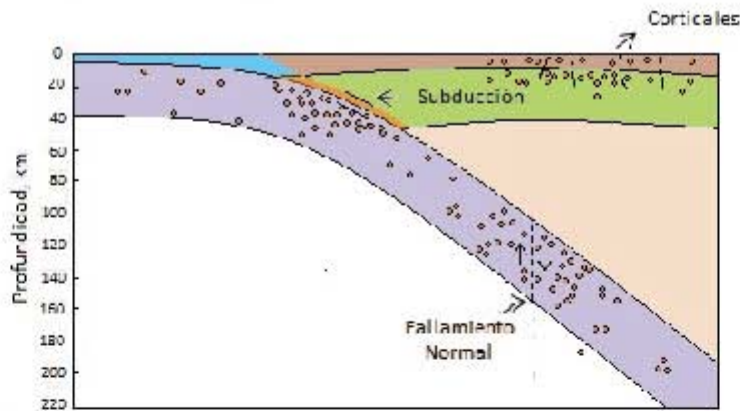
Figura 2.2.2: Tipos principales de sismos considerados
