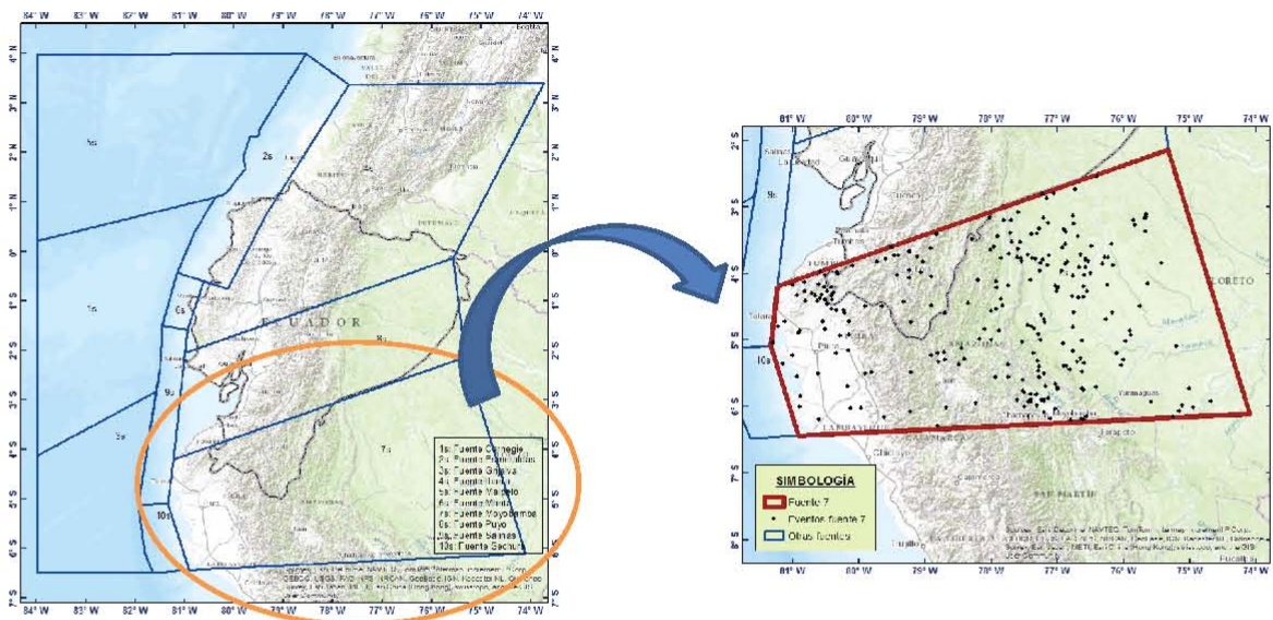
Figura 4.3.4: Eventos registrados en el catálogo para la fuente 7, (Moyobamba)
