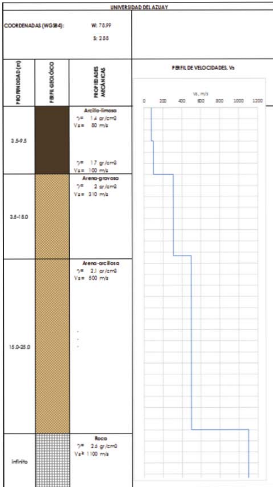
Figura 5.2.4: Perfil geológico, Universidad del Azuay
