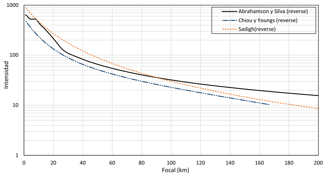
Figura 4.4.2: Comparación entre modelos de atenuación corticales para fallas tipo inversas
