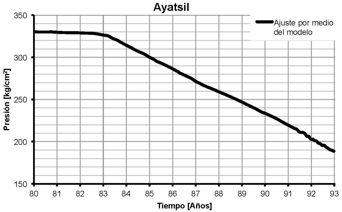
Fig. 4.17 Declinación de la presión promedio del yacimiento Ayatsil
