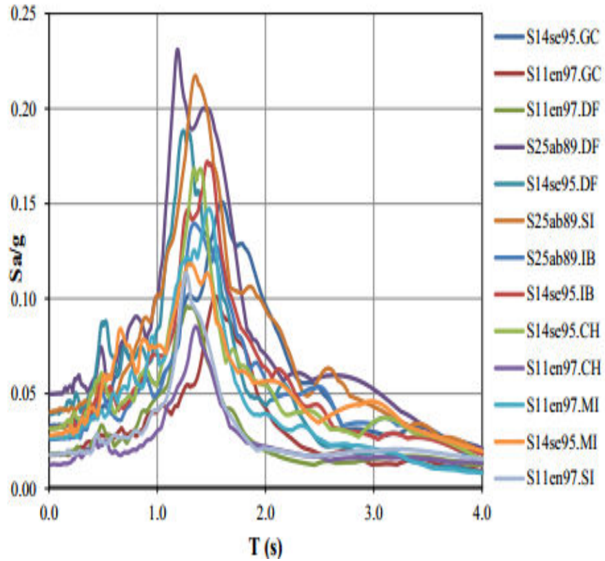
Figura 3.2 Conjunto de espectros de respuesta utilizados en el estudio, correspondientes a 5% de amortiguamiento crítico.
