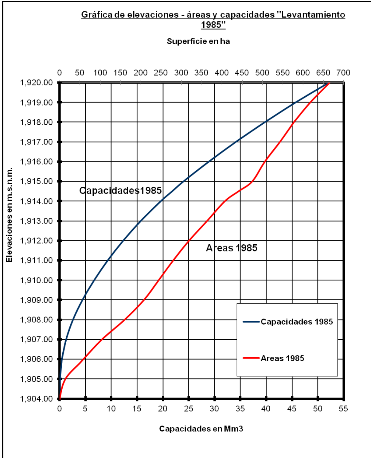
Gráfica de elevaciones - áreas y capacidades del levantamiento de 1985 (con datos de 1992)
