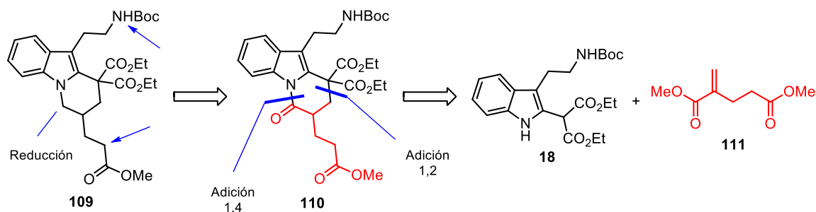
Esquema 32. Retrosíntesis planteada para el compuesto indólico 109 .
