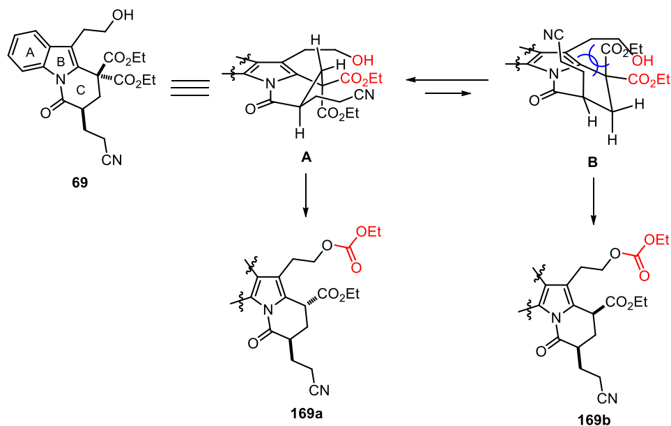
Esquema 69. Propuesta desarrollada para explicar la estereoquímica observada en el compuesto 169a .
