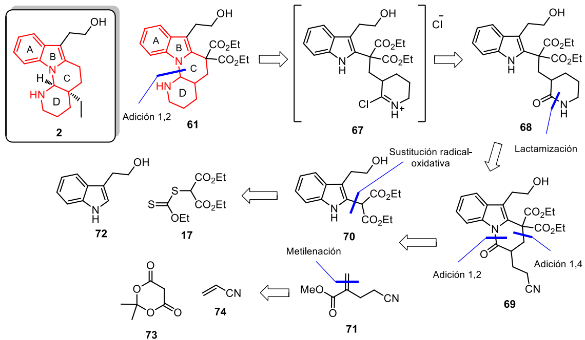
Esquema 16. Retrosíntesis planteada para el compuesto tetracíclico 61 .
