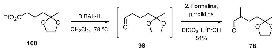
Esquema 28. Optimización de la síntesis del aldehído insaturado 78 .
