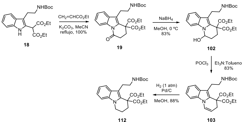
Esquema 33. Estudio modelo realizado para demostrar que la desoxigenación del compuesto 19 es posible.
