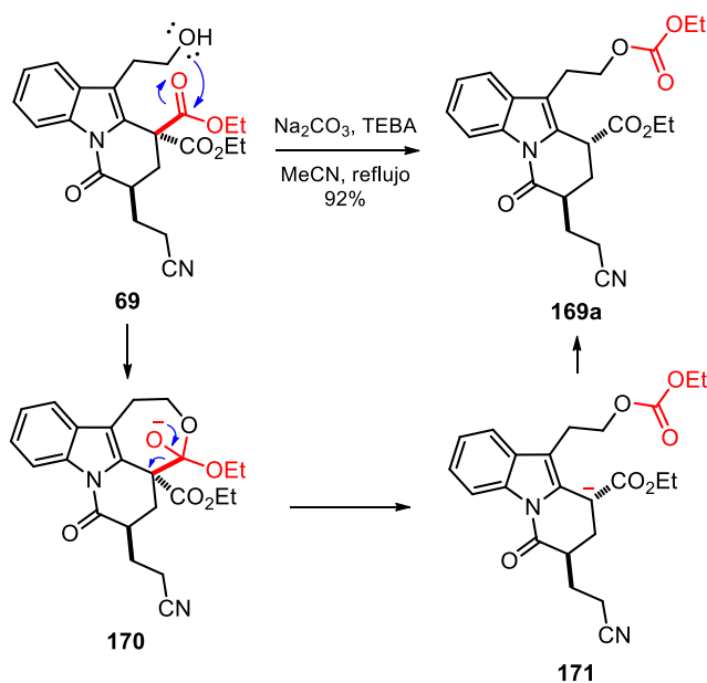
Esquema 68. Propuesta mecanística que explica la formación de 169a a partir del piridoindol 69 .
