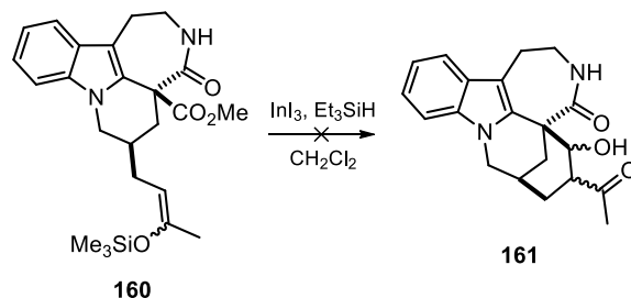
Esquema 63. Ensayo para la preparación del pentaciclo 161 a través de una reacción de Mukaiyama.
