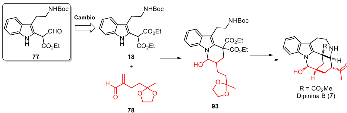
Esquema 25. Modificación de la ruta de síntesis para la dipinina B.
