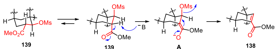
Esquema 51. Propuesta mecanística para la eliminación del mesilato por medio de un proceso S_N2' .
