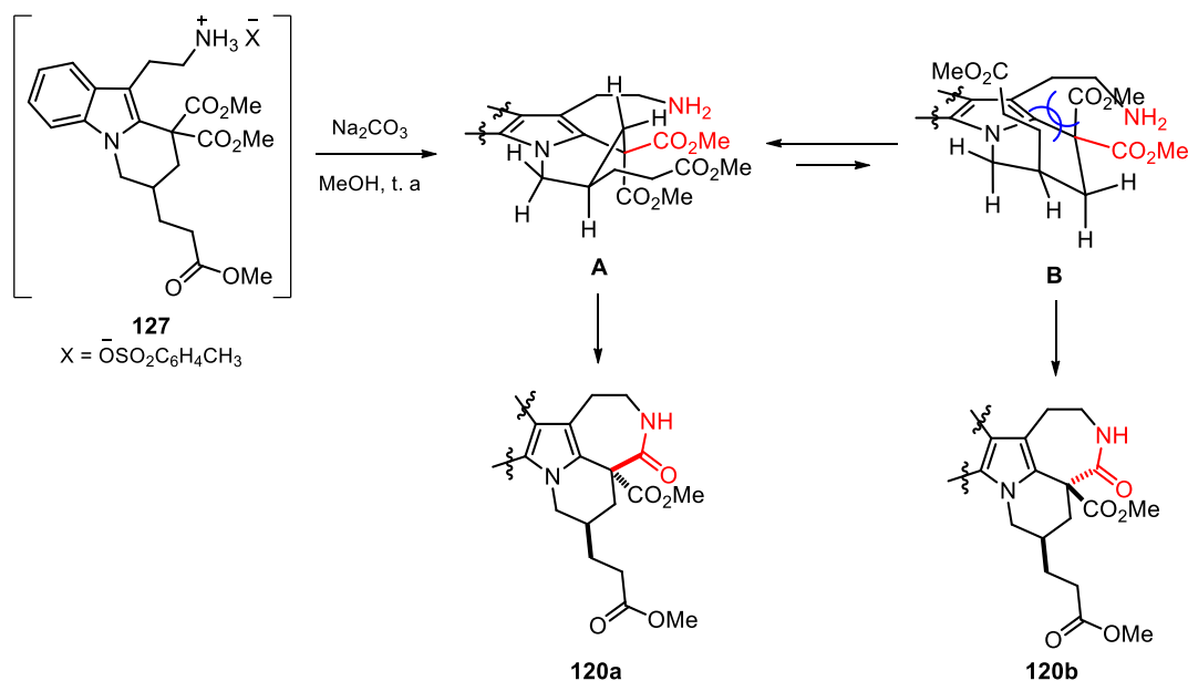
Esquema 42. Explicación del resultado estereoquímico para el compuesto 120a .
