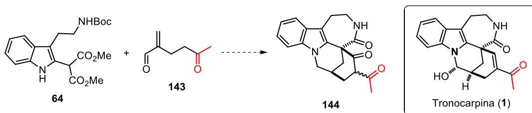
Esquema 54. Propuesta sintética para la preparación del intermediario pentacíclico 144 .
