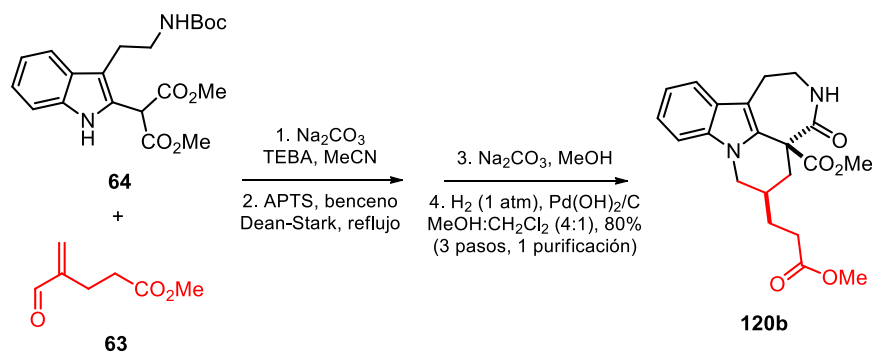
Esquema 44. Optimización de la síntesis de 120b .
