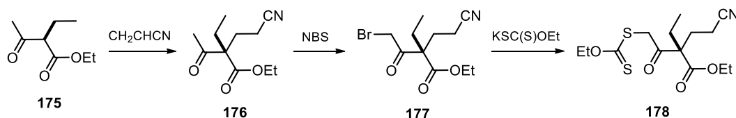
Esquema 71. Propuesta de síntesis para el xantato 178 .
