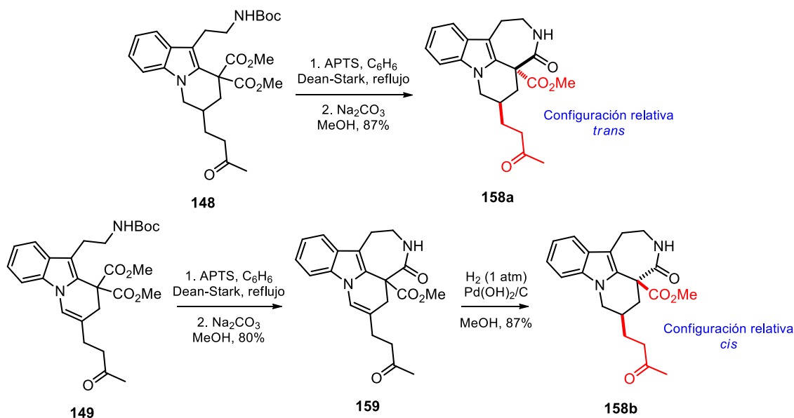
Esquema 59. Preparación de los diastereoisómeros tetracíclicos 158a y 158b .
