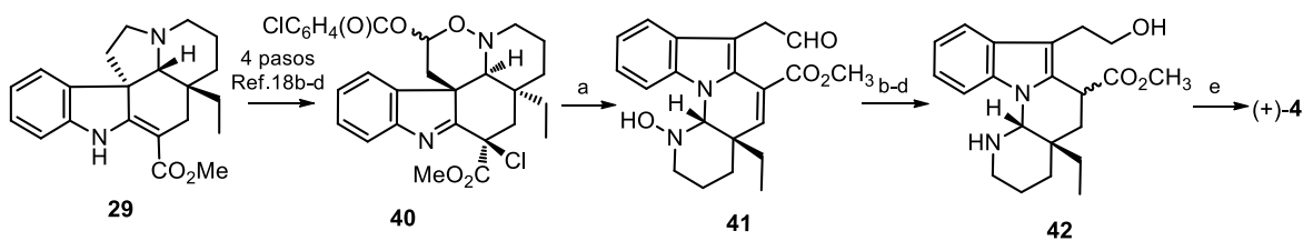
Esquema 8. Síntesis parcial de la goniomitina de Lewin.
