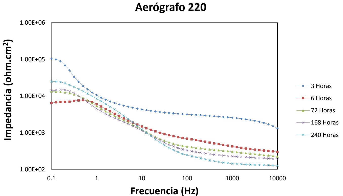
Fig. 5.1.3a Comportamiento del Sol-Gel en la placa de lija 220 en deposición de Aerógrafo en NaCl 0.1 M.
