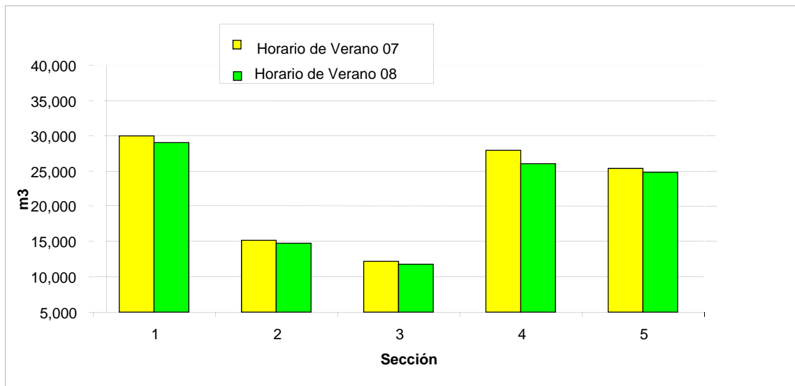
Gráfica 27. Consumo de energía térmica por sección de la Unidad Habitacional STUNAM Culhuacán para los periodos de Horario de Verano 2007 y Horario de Verano 2008 (en m 3 ).
