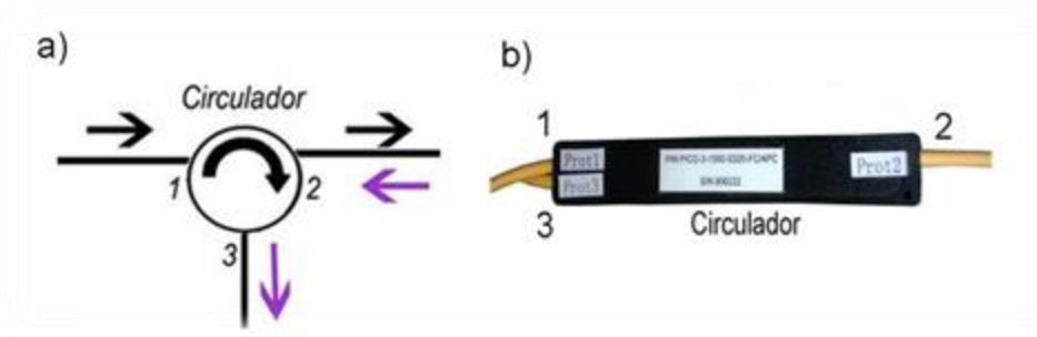
Figura 19. a) Ilustración del funcionamiento de un circulador óptico. b) Circulador óptico PIOC-3-1550-S320-FC/APC
