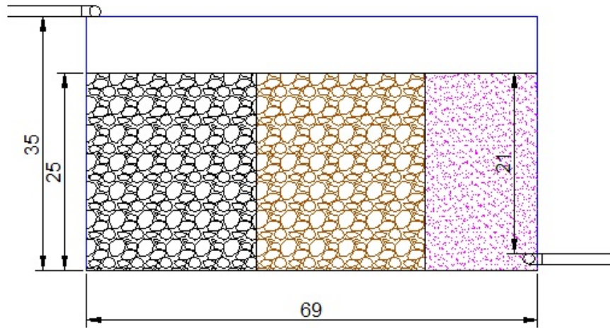
Figura 5-6. Esquema del HACEV (vista: lateral).
