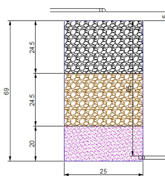
Figura 5-11. Esquema del HACEH (vista: lateral).
