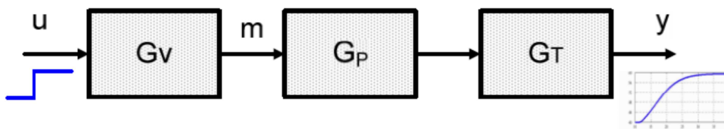
Figura 3.9 proceso Ziegler y Nichols
