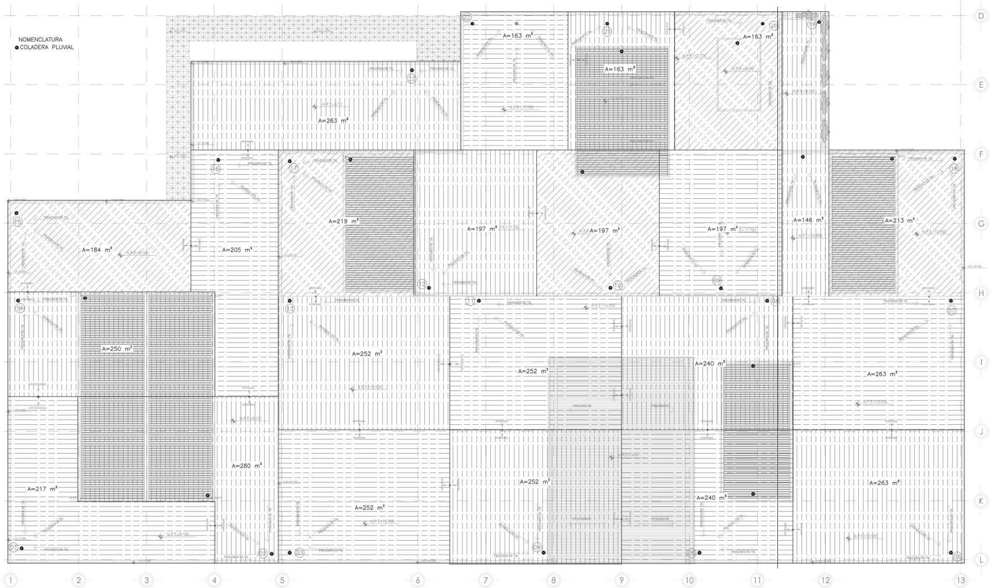
Figura 4.2. Distribución de coladeras en azotea
