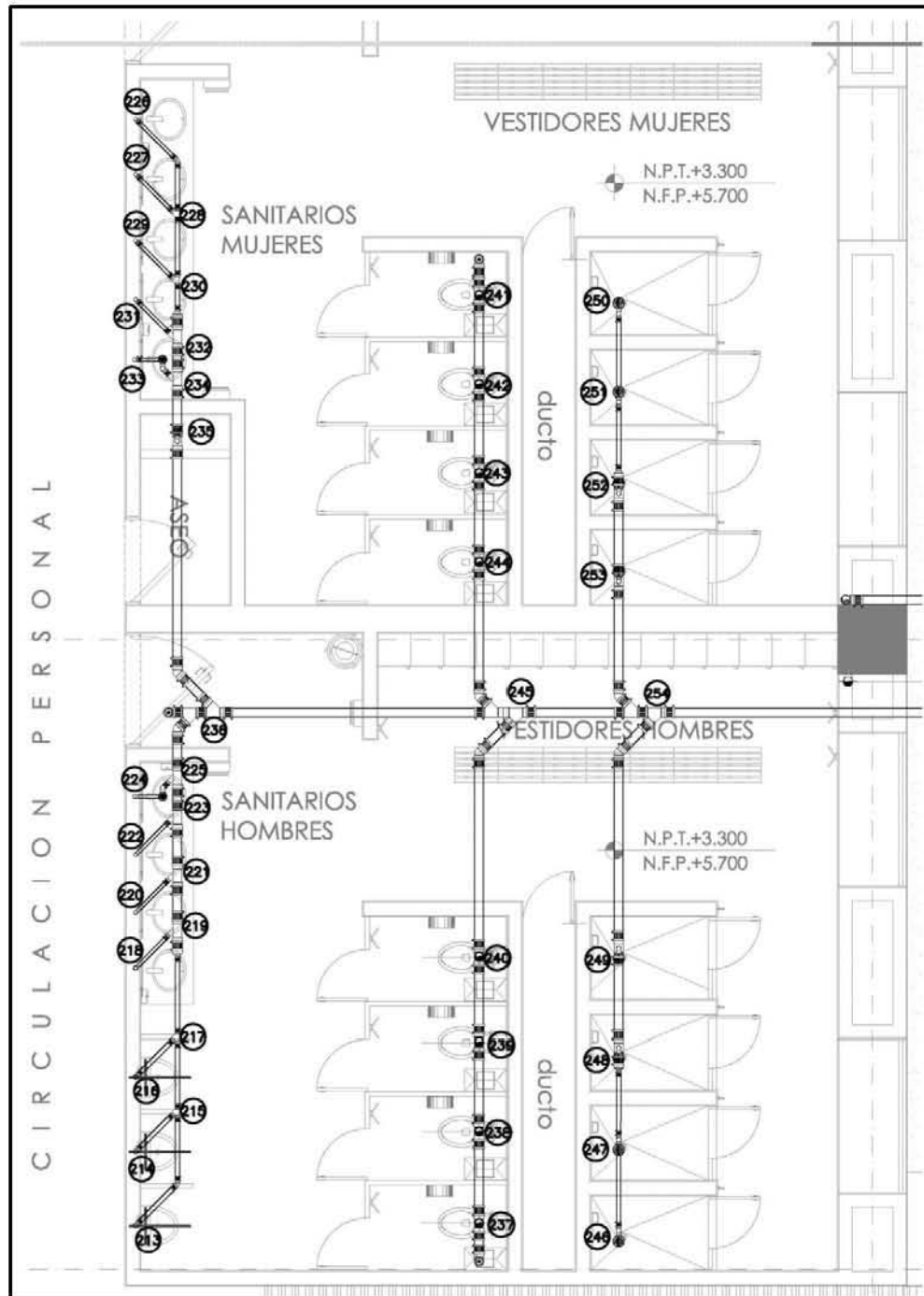
Figura 3.1. Núcleo 7 planta baja
