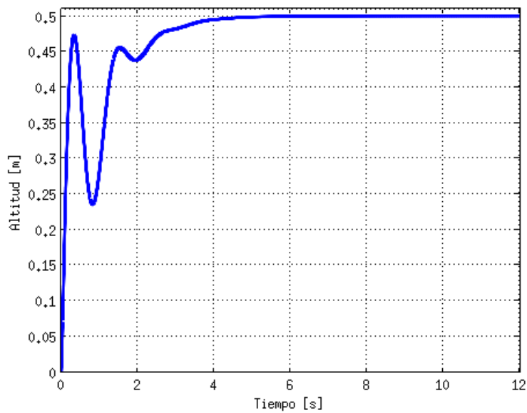
Figura 3.4 Simulación del controlador de altitud corregido.
