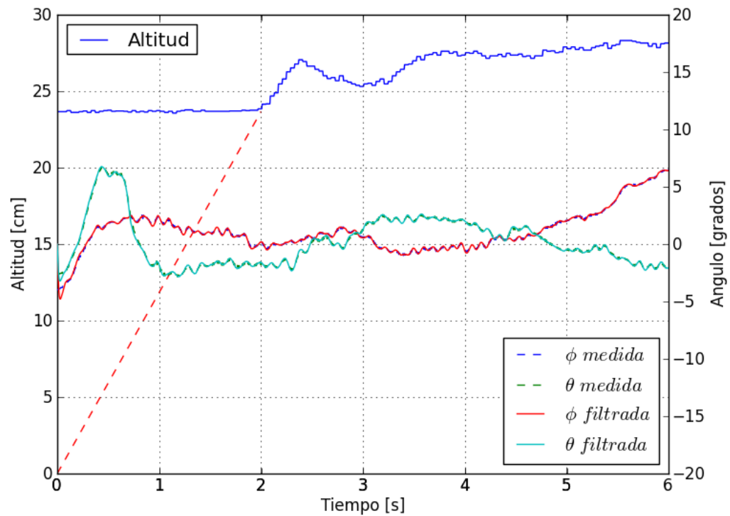
Figura 5.12 Ángulos y altitud en prueba de vuelo con perturbación. Control Supertwisting.
