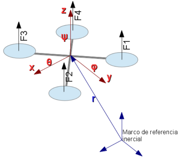
Figura 2.2 Modelo simplificado y marco de referencia.
