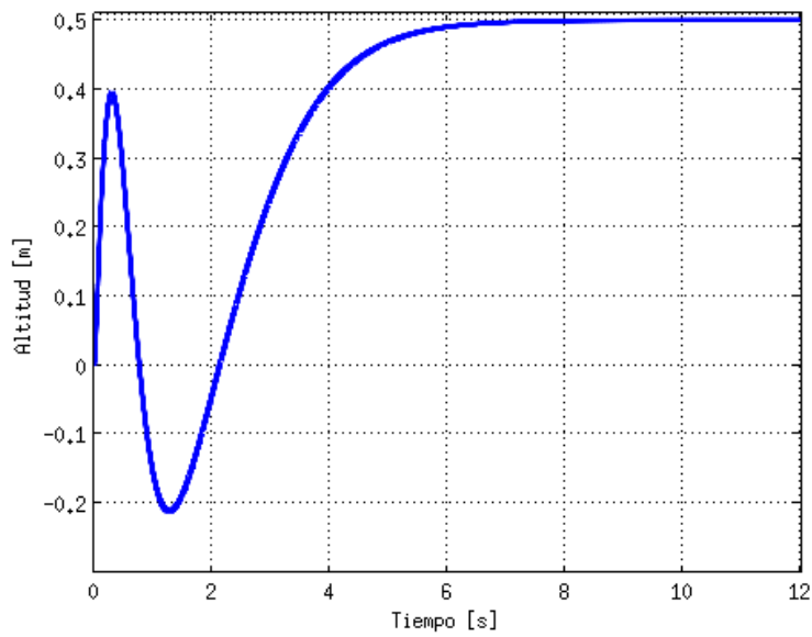
Figura 3.3 Primera simulación del control de altitud.
