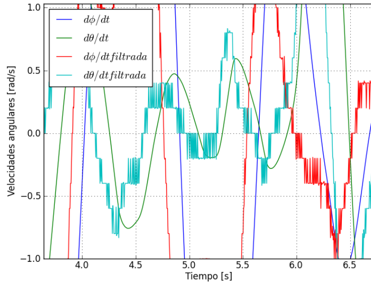
Figura 5.8 Velocidad angular filtrada
