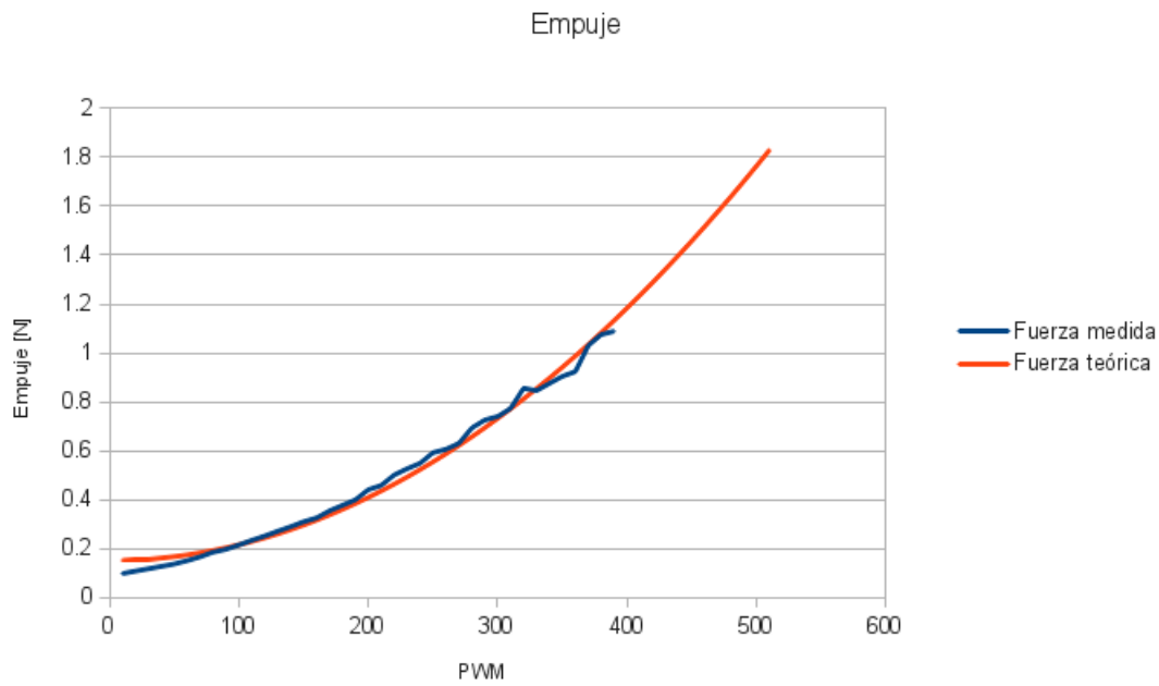
Figura 2.4 Empuje medido y regresión lineal.
