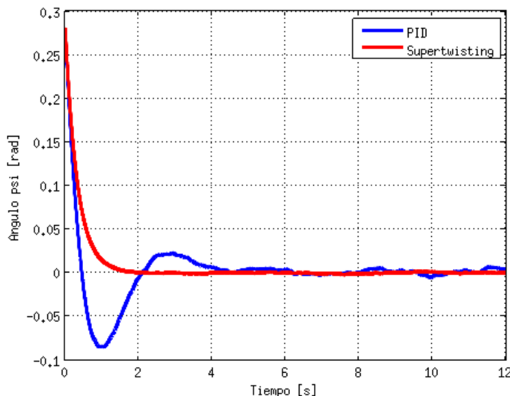
Figura 3.13 Comparación de control PID contra Super-twisting en ángulo \psi .
