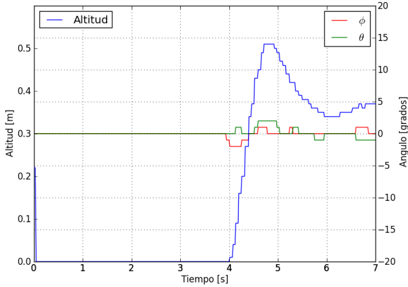
Figura 5.13 Gráfica del comportamiento del controlador de fábrica sin perturbaciones.
