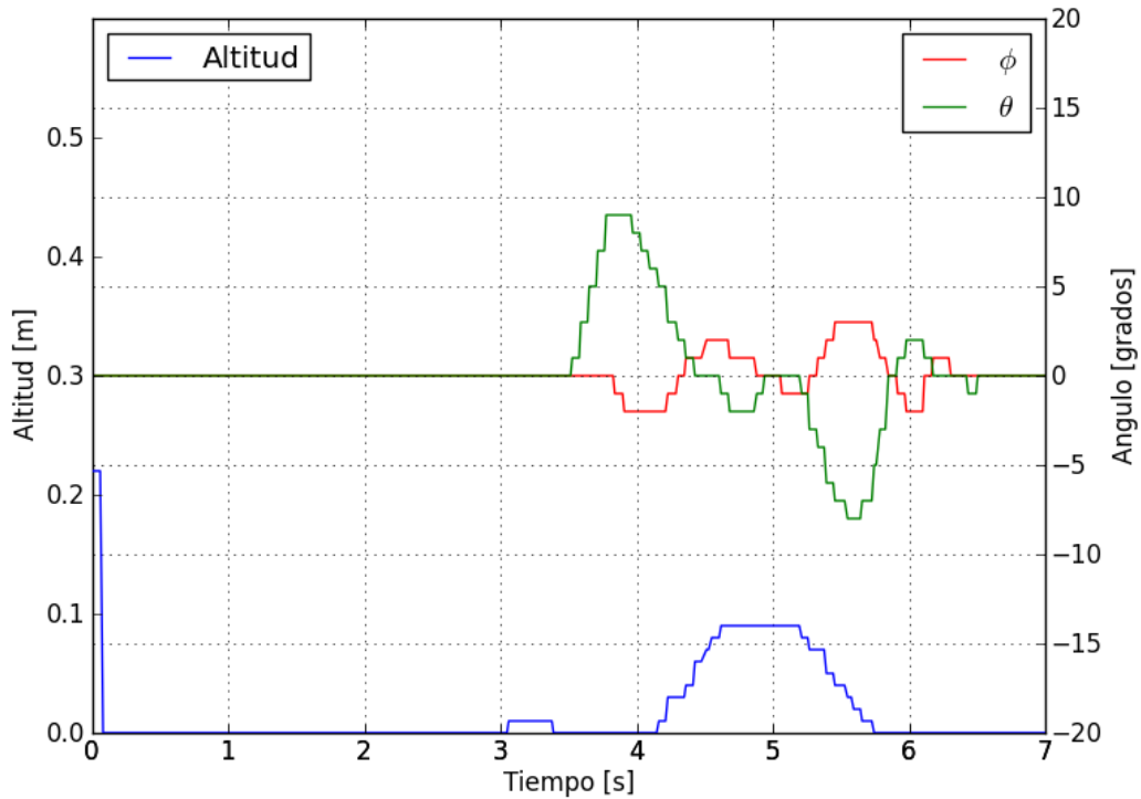
Figura 5.16 Ángulos y altitud en prueba de vuelo con perturbación. Control de fábrica.
