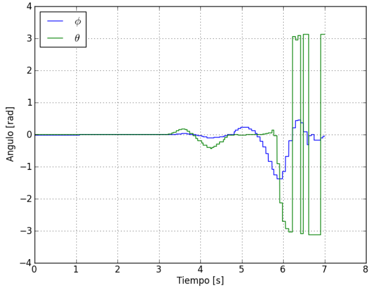
Figura 5.2 Ángulos en experimento de vuelo.
