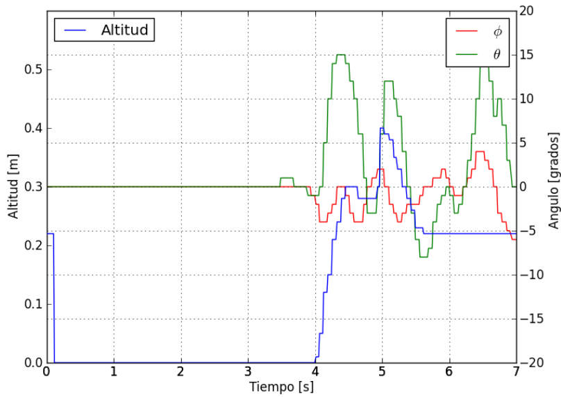
Figura 5.14 Ángulos y altitud en prueba de vuelo con perturbación. Control de fábrica.
