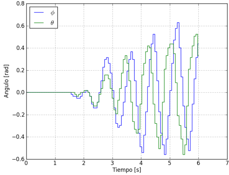
Figura 5.3 Ángulos en experimento de vuelo.
