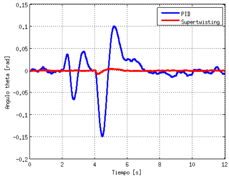
Figura 3.12 Comparación de control PID contra Super-twisting en ángulo \theta .
