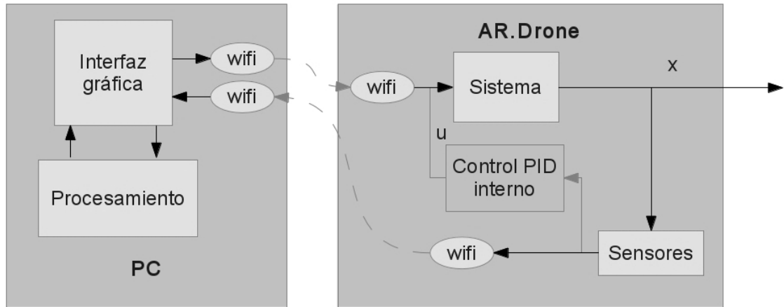
Figura 5.1 Modelo de funcionamiento propuesto.
