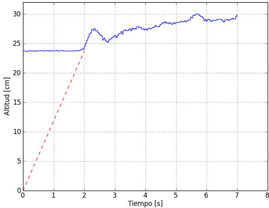
Figura 5.11 Altitud en prueba de vuelo .
