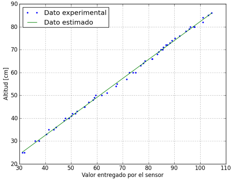
Figura 5.10 Calibración del sensor de altitud.
