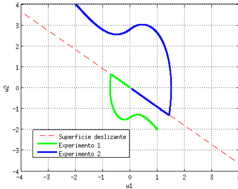
Figura 3.7 Simulación del modo deslizante.
