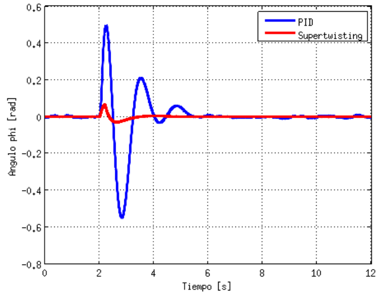
Figura 3.11 Comparación de control PID contra Super-twisting en ángulo \phi .
