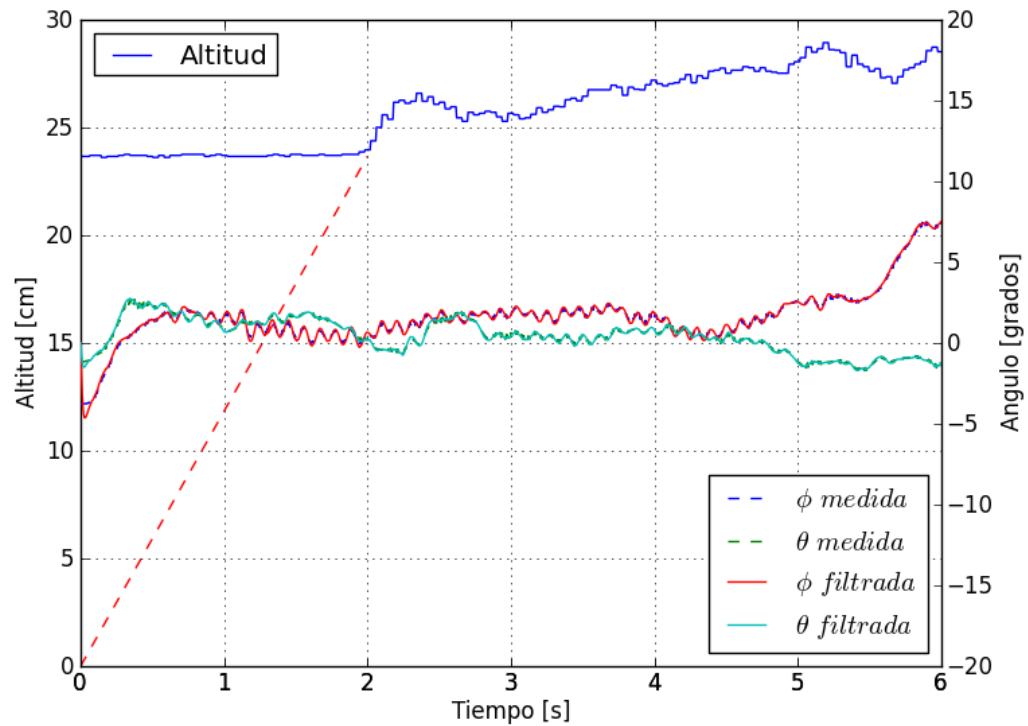
Figura 5.15 Ángulos y altitud en prueba de vuelo con perturbación. Control Supertwisting.
