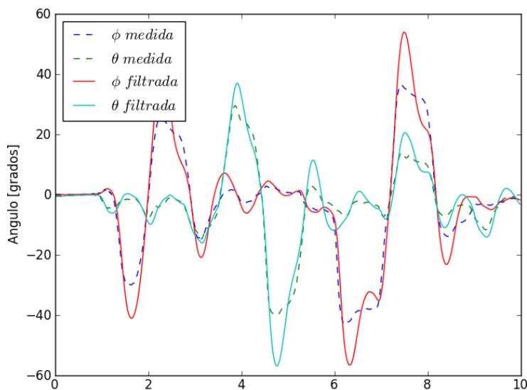
Figura 5.7 Señal de ángulos filtrada.
