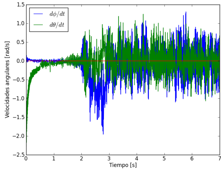
Figura 5.6 Derivada numérica de los ángulos medidos.
