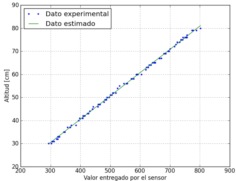
Figura 4.4 Calibración del sensor de altitud.
