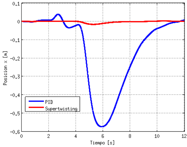
Figura 3.9 Comparación de control PID contra Super-twisting en eje x .
