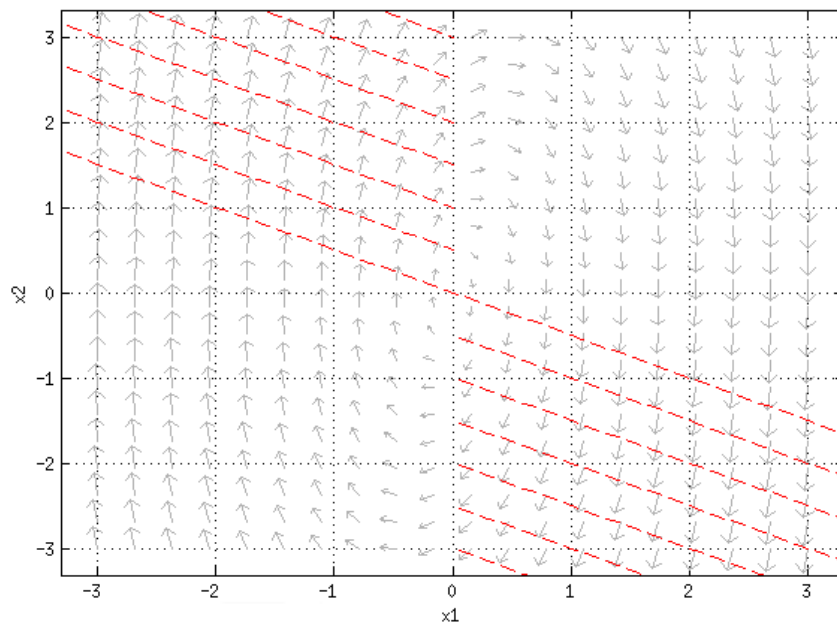
Figura 3.6 Plano de fase para la ganancia k = 6 .
