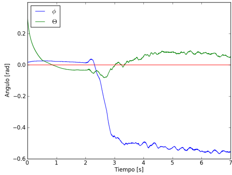
Figura 5.5 Experimento de medición de ángulos.
