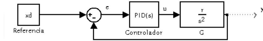
Figura 3.1 Diagrama de bloques del controlador PID.
