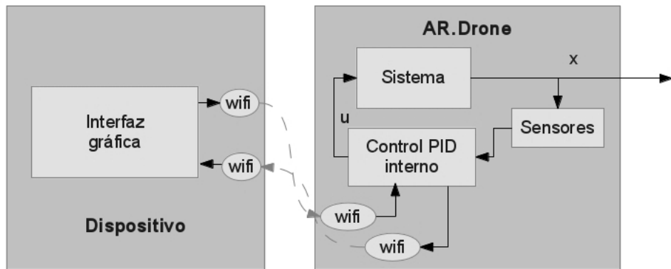
Figura 4.1 Modelo de funcionamiento de fábrica.
