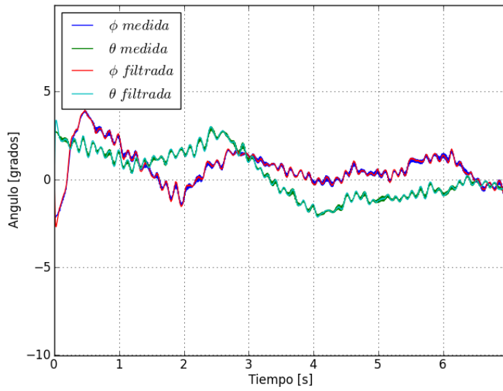
Figura 5.9 Prueba de vuelo. Señal de ángulos filtrada.
