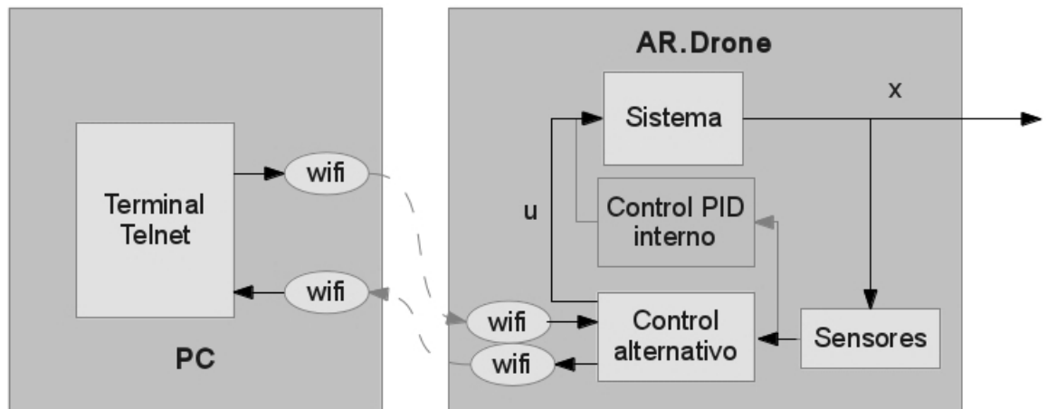
Figura 5.4 Modelo de funcionamiento propuesto.
