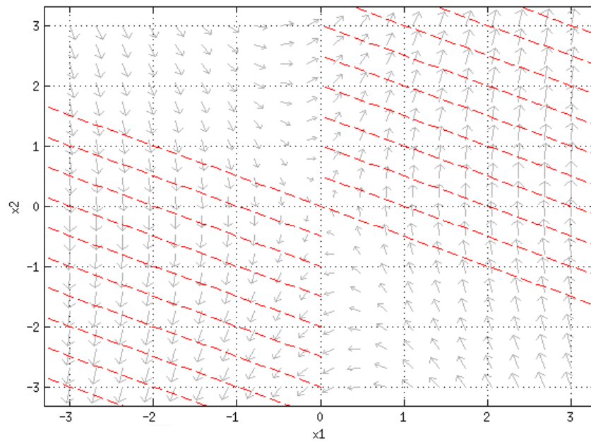
Figura 3.5 Plano de fase para la ganancia k = -6 .
