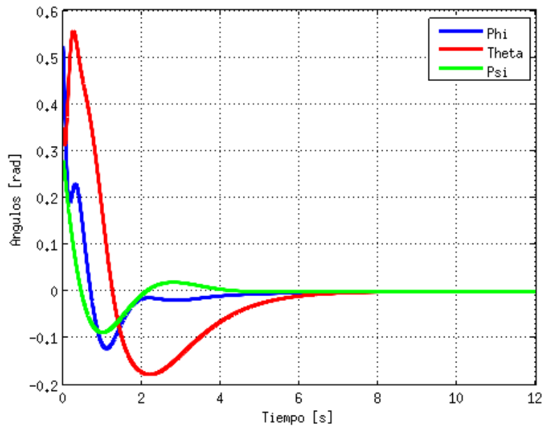
Figura 3.2 Simulación de estabilización de los ángulos.
