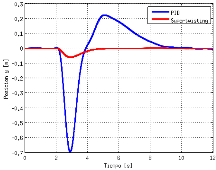
Figura 3.10 Comparación de control PID contra Super-twisting en eje y .
