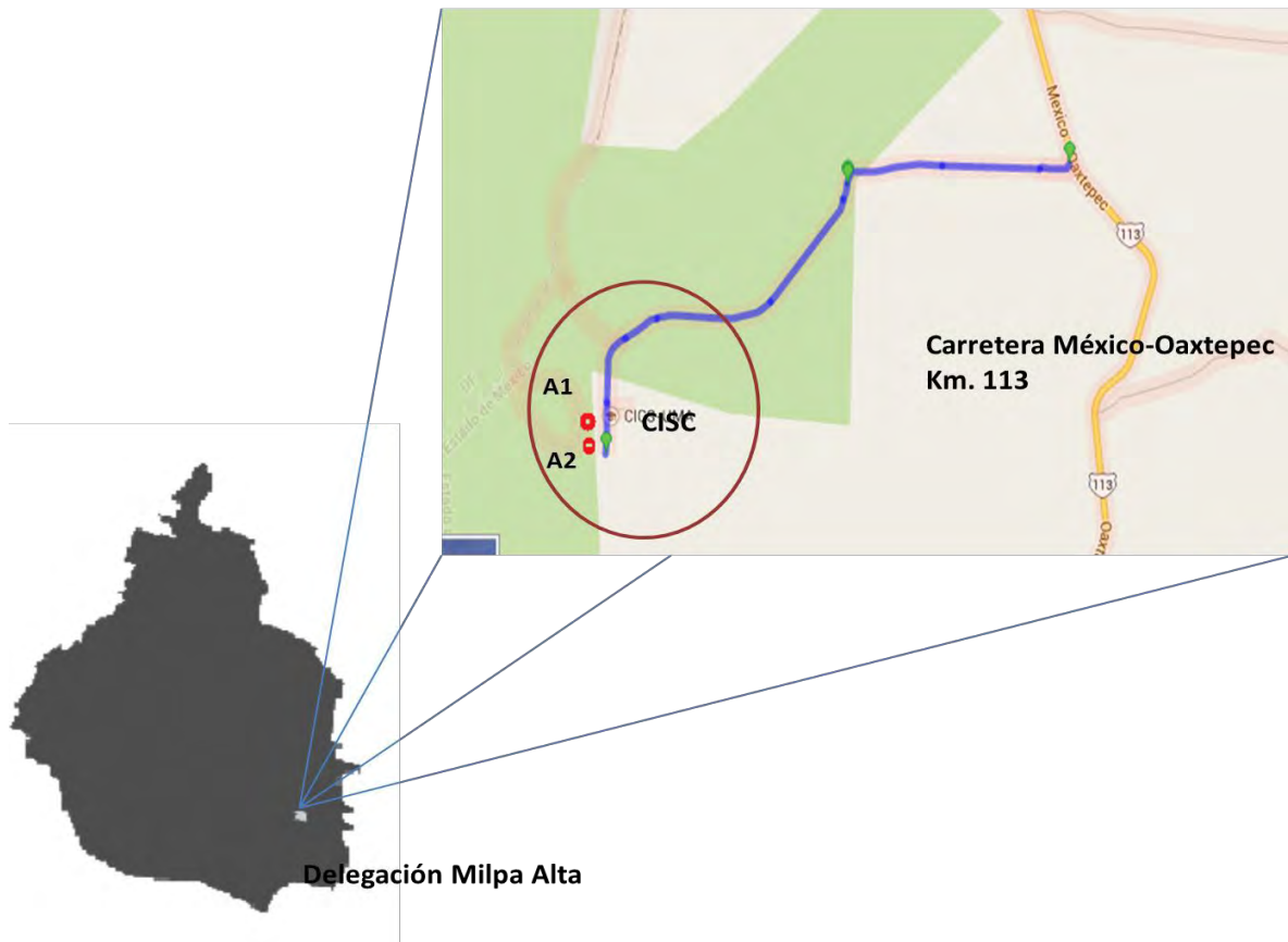
Figura 5. Ubicación del área de estudio para Sceloporus torquatus , la parte superior muestra en círculos rojos (A1 y A2) los sitios de colecta y el círculo guinda representa El CISC (Centro Interdisciplinario de Ciencias de la Salud). (Fuente: Google, INEGI, 2013).
