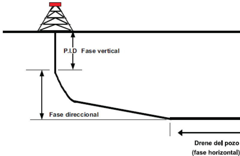
Figura 3.8 Perforación horizontal.
