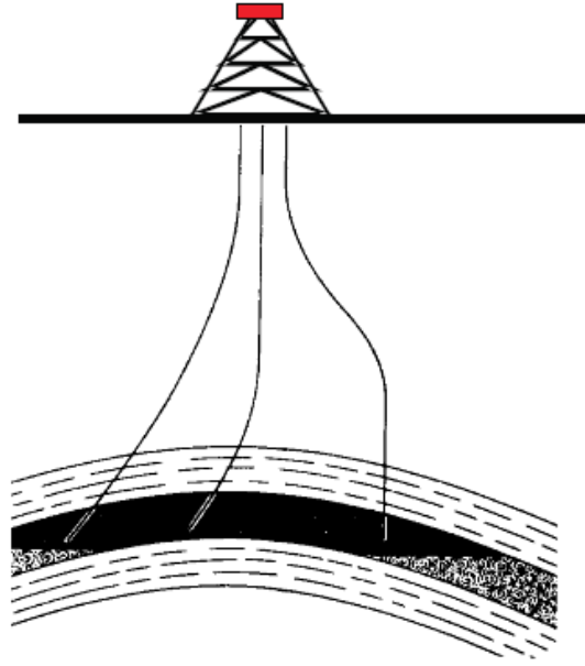
Figura 3.6 Perforaciones múltiples desde un mismo sitio.
