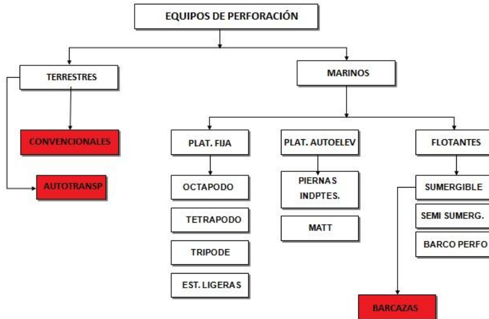
Figura 3.4. En rojo los equipos usados para perforar en zonas de humedales. (Soto Pineda, 2004).
