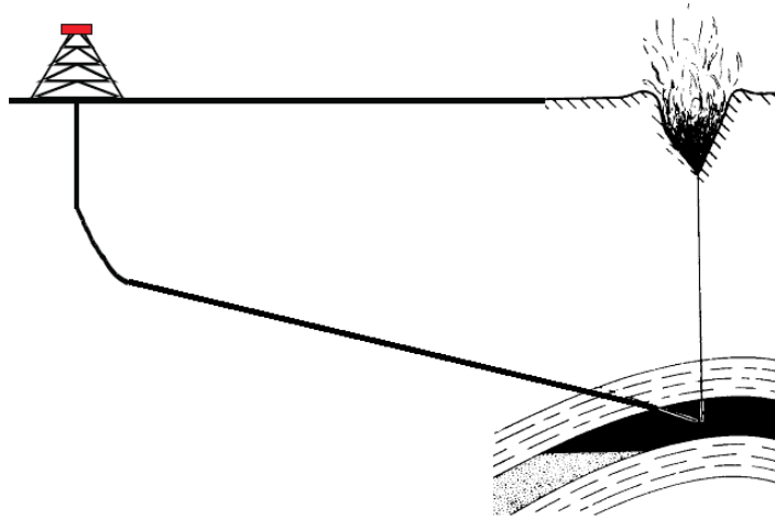
Figura 3.7 Perforación de pozos de alivio.
