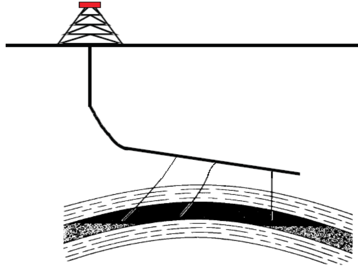
Figura 3.5 Perforación tipo multilateral.
