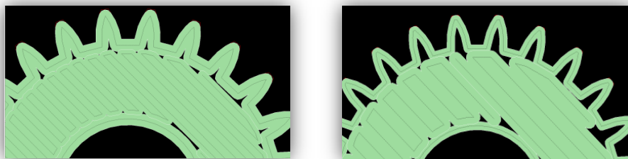
Figura 13. Trayectorias de deposición generadas con distintos parámetros para un mismo engrane.
