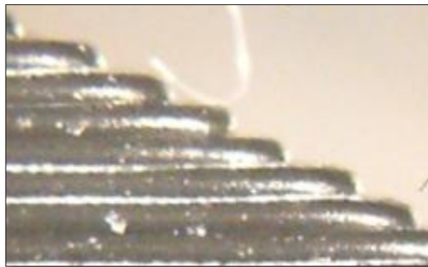
Figura 34. Efecto de escalonamiento en las construcciones FDM.
