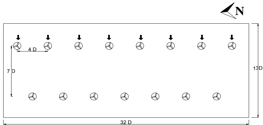
Figura 3.8 Distribución de aerogeneradores, arreglo No. 4
