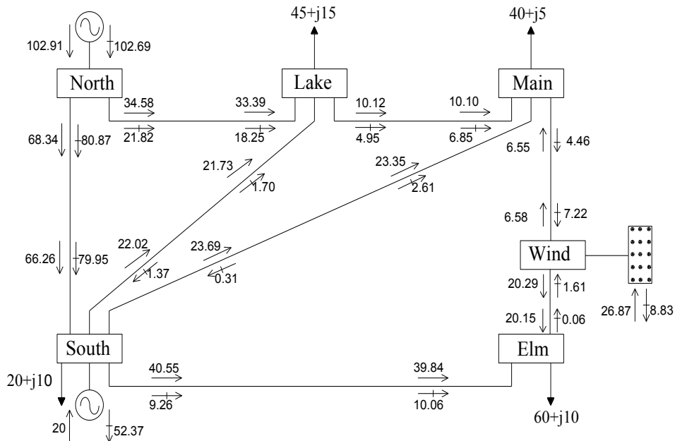
Figura 4.8 Flujos de potencia, arreglo No. 4
