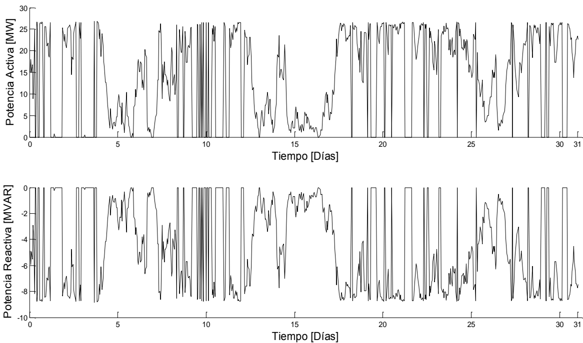
Figura 5.2 Potencia activa y reactiva entregada por el parque, arreglo No. 3
