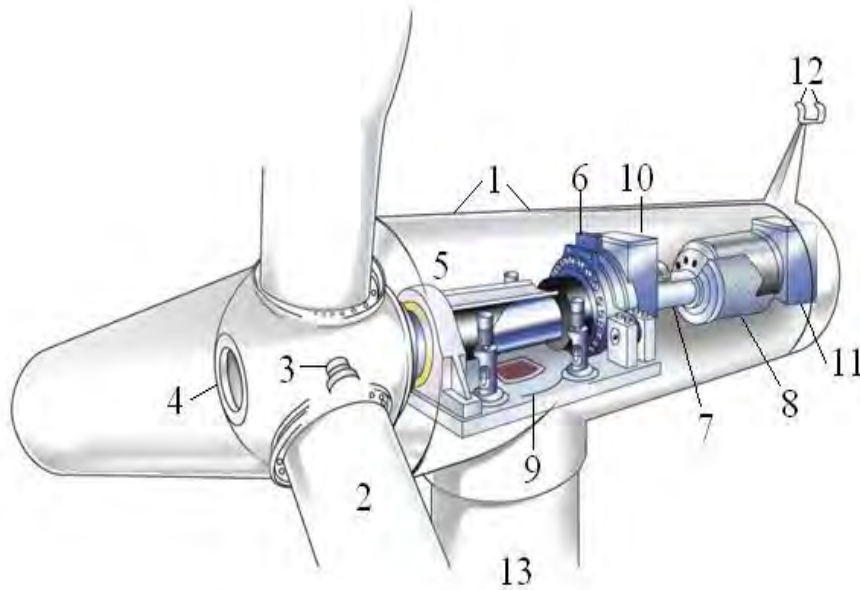
Figura 3.1 Sistemas de Conversión de Energía Eólica WECS
