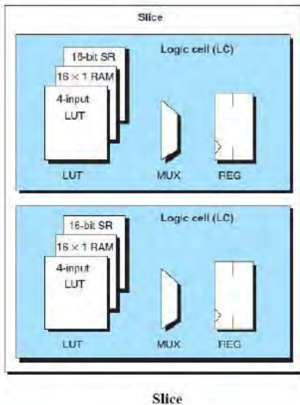
Figura 4.4 Configuración de una sección. [19]
