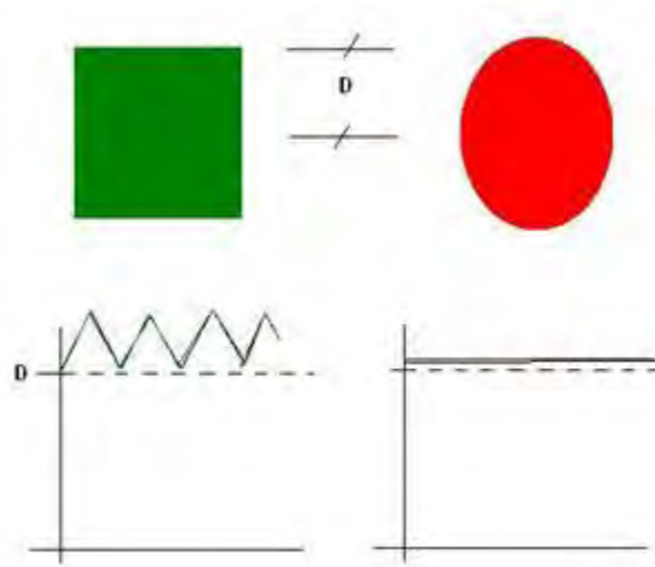
Figura 3.2 Función de frontera de un cuadrado y un círculo. Comparación del BOF de dos figuras regulares de dimensiones aproximadas. [Elaboración propia]
