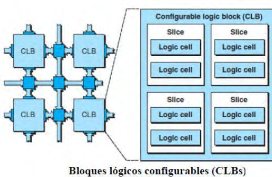
Figura 4.3 Configuración de un bloque lógico configurable. [19]
