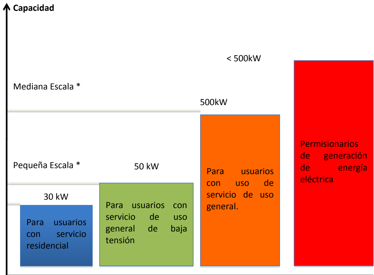
Gráfica II-1.- Escala para contratos de interconexión Fuente: Comisión Reguladora de Energía, (2010)
