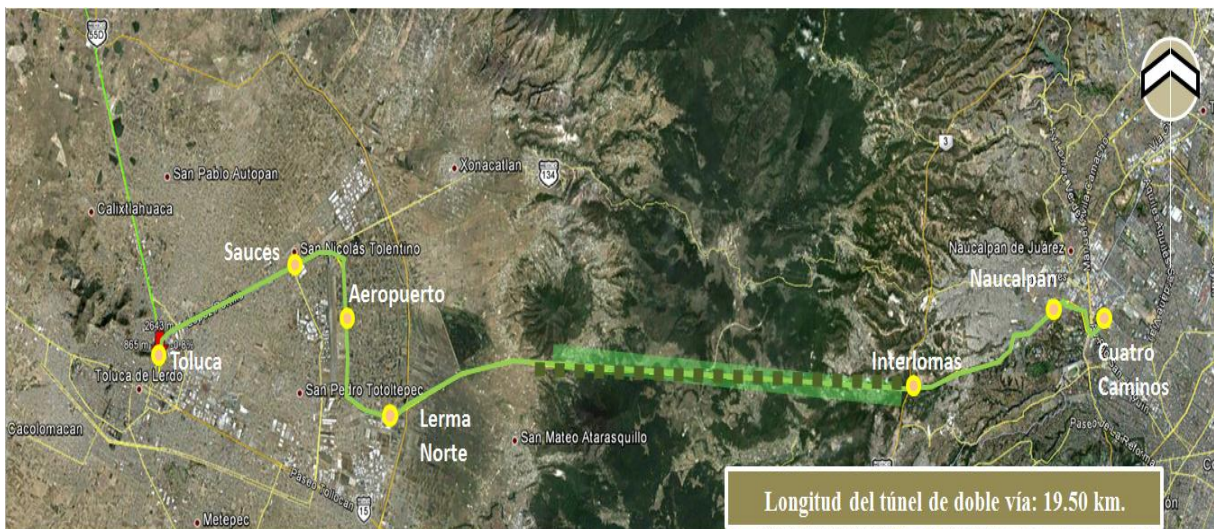
Figura # 4.18. Trazo propuesto del túnel de doble vía.
