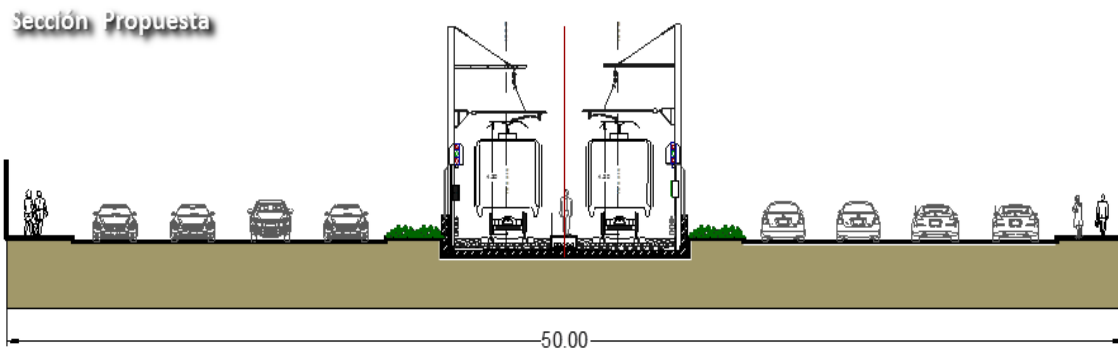
Figura # 4.14. Sección propuesta del proyecto en el Boulevard Aeropuerto.
