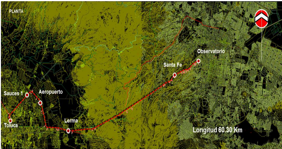
Figura # 3.2. Planimetría de INEGI del trazo Toluca – Observatorio.
