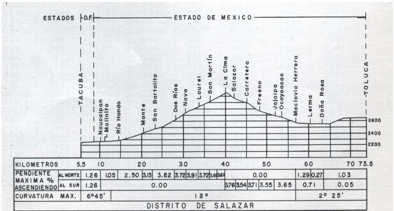
Figura # 2.2. Perfil longitudinal de la Línea N del Horario 11 de Ferrocarriles Nacionales de México.
