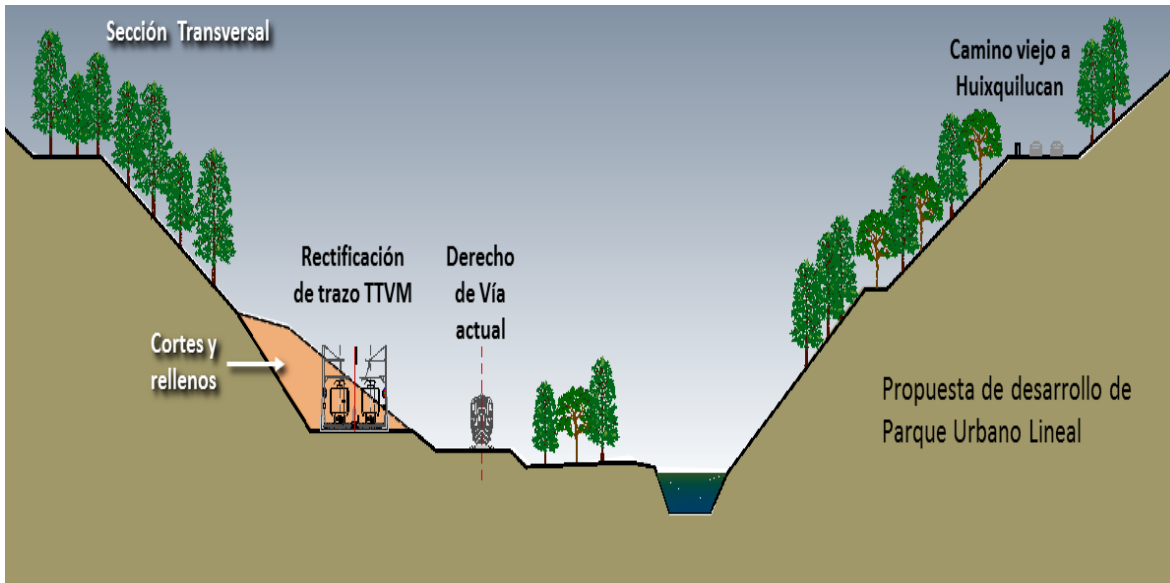
Figura # 4.24. Propuesta de sección transversal en la cañada.
