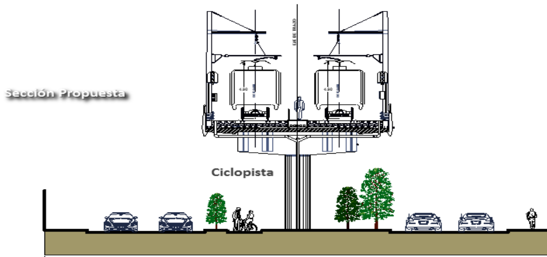
Figura # 4.28. Sección propuesta de trazo sobre el derecho de vía de la Línea N.
