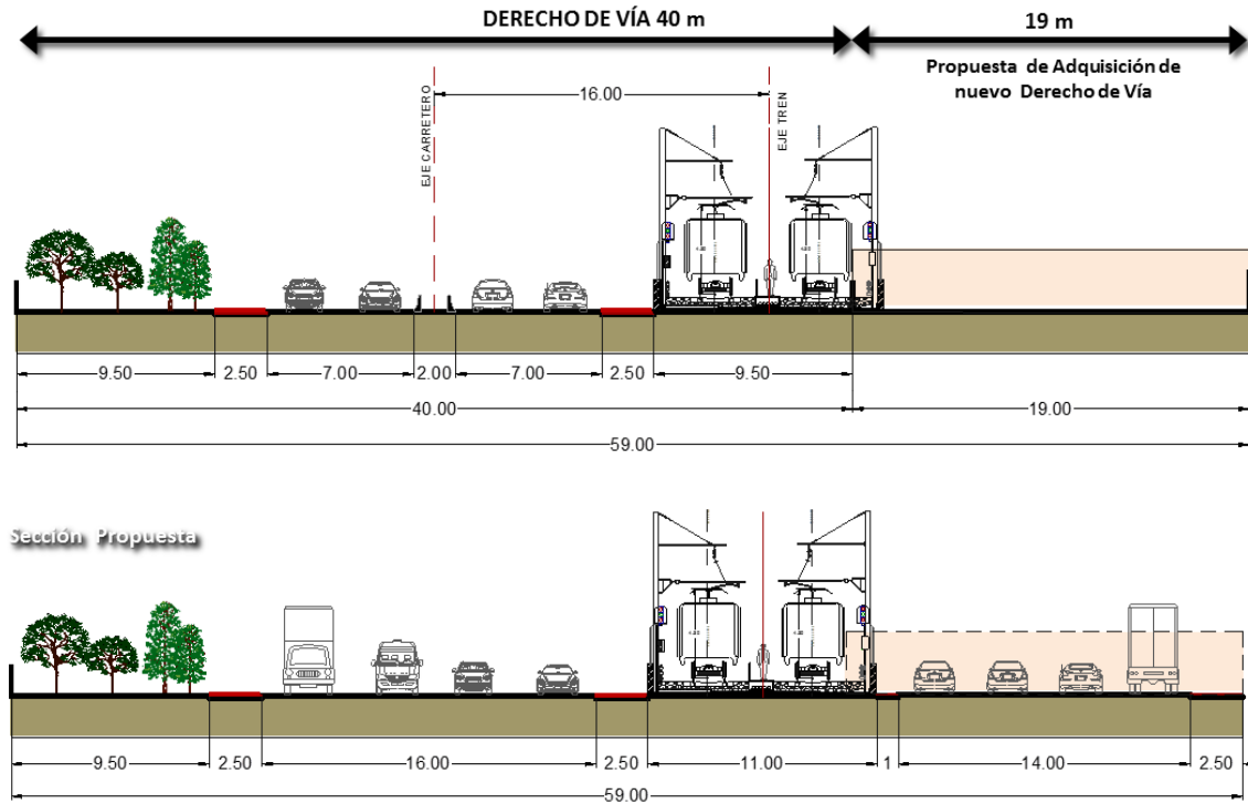
Figura # 4.17. Propuesta de sección transversal de la Autopista Toluca - Naucalpan.
