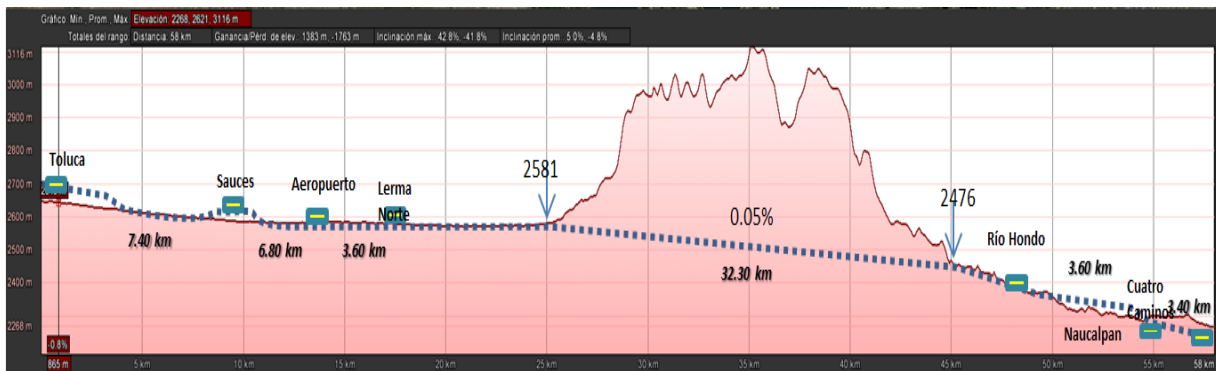
Figura # 4.3. Perfil del trazo Toluca – Cuatro Caminos.
