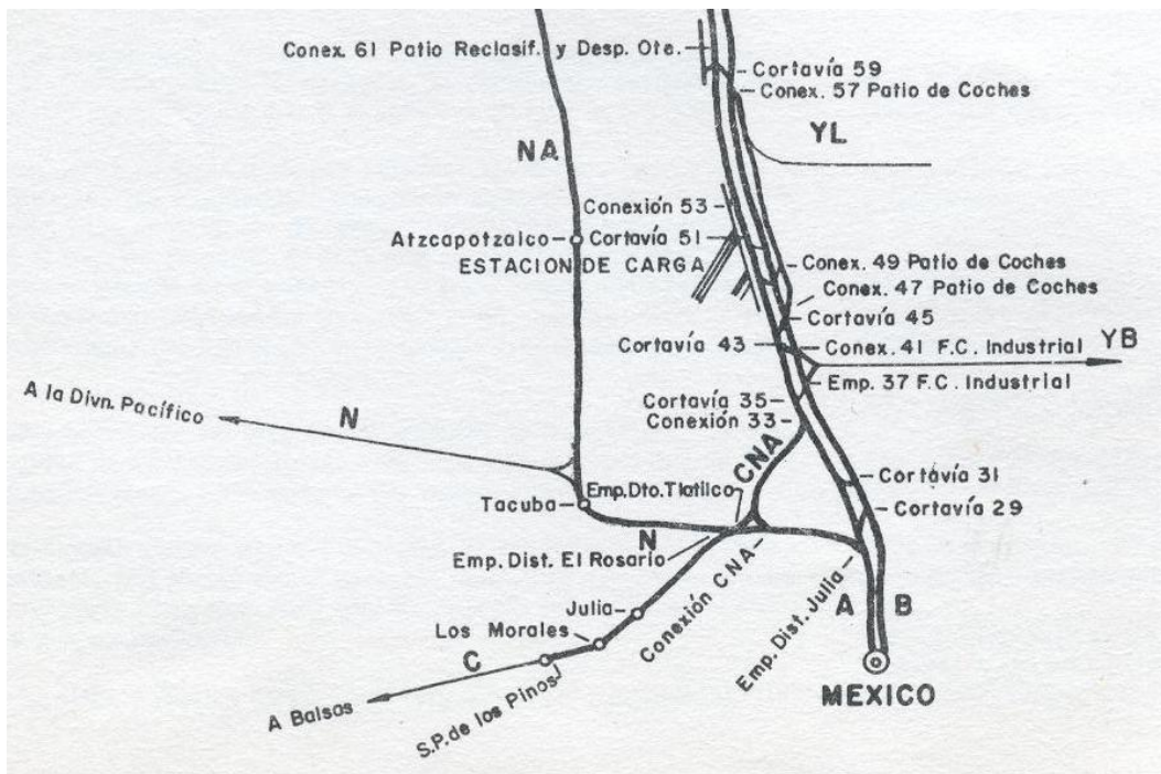
Figura # 2.1. Esquema de Ferrocarriles Nacionales de México sobre las vías en el Valle de México.
