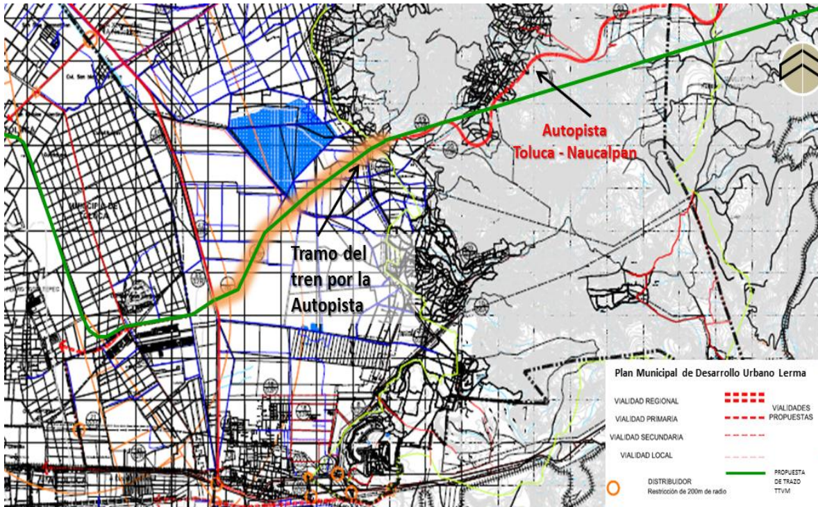
Figura # 4.15. Trazo propuesto del proyecto por la Autopista Toluca – Naucalpan.
