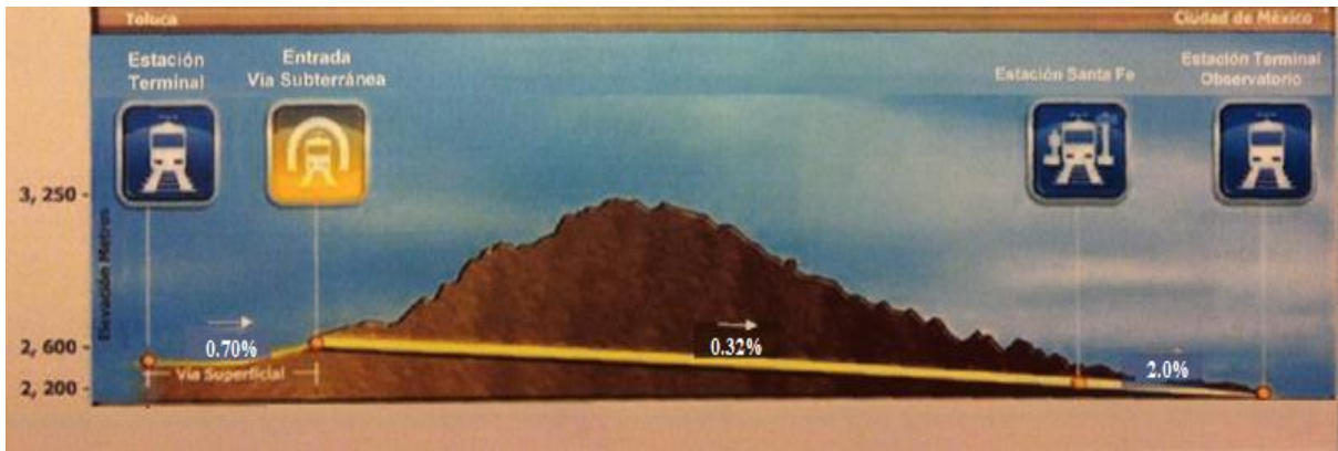
Figura # 3.4. Trazo y elevaciones de la ruta Toluca – Observatorio.
