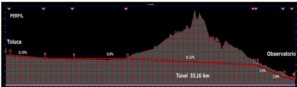
Figura # 3.3. Perfil del terreno y pendientes propuestas del trazo Toluca – Observatorio.
