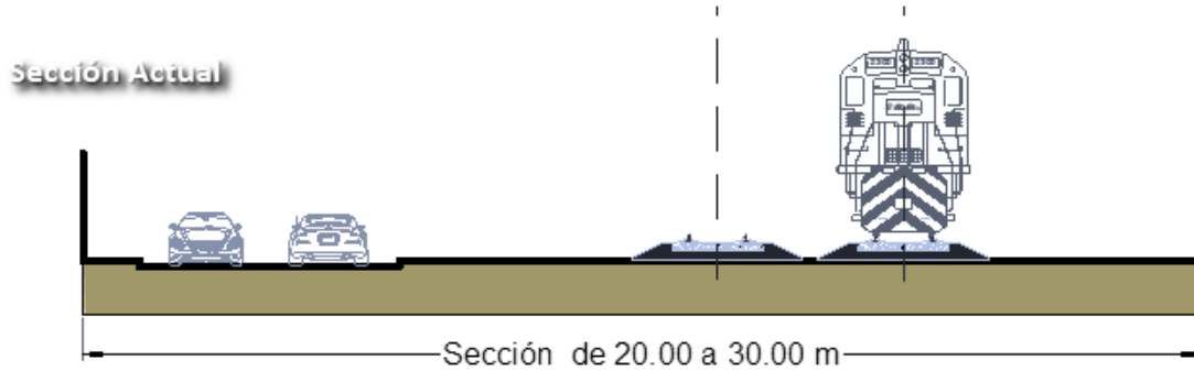
Figura # 4.27. Sección actual de la Línea N en Naucalpan.
