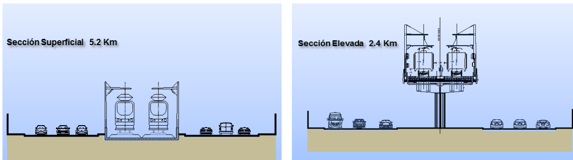
Figura # 4.7. Sección propuesta en la Avenida López Portillo.
