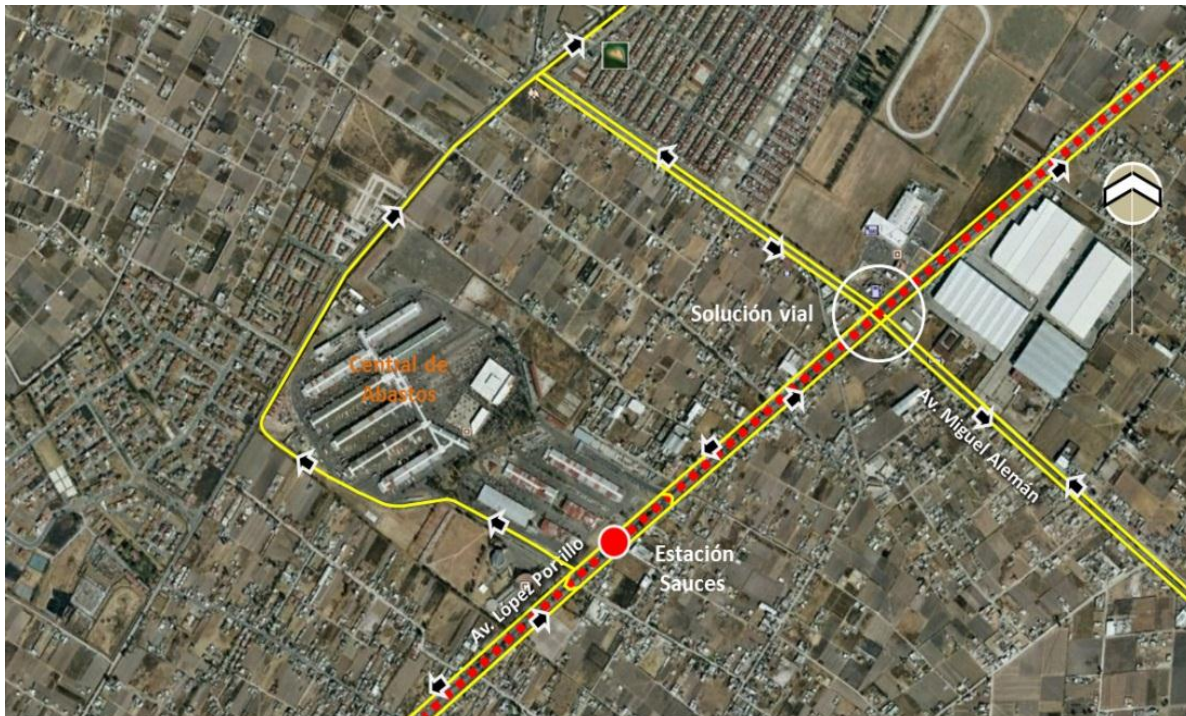
Figura # 4.10. Estructura vial propuesta de la estación Sauces.
