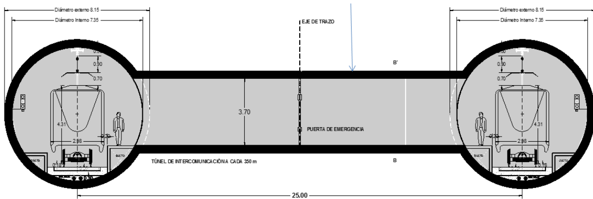
Figura # 4.19. Sección propuesta del túnel de doble vía.
