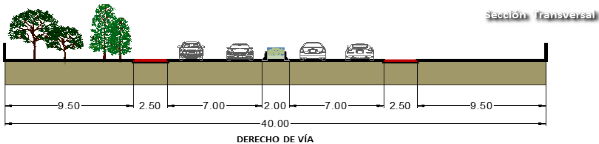
Figura # 4.16. Sección transversal actual de la Autopista Toluca - Naucalpan.
