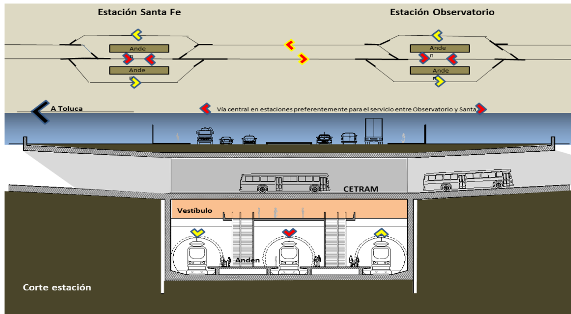
Figura # 3.9. Esquema de vías entre las estaciones Observatorio y Santa Fe.
