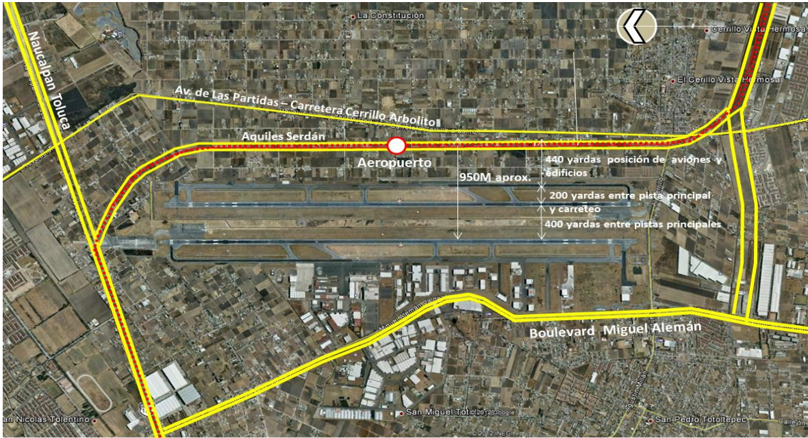
Figura # 4.11. Ubicación propuesta de la estación Aeropuerto de Toluca.
