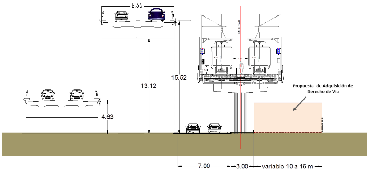
Figura # 4.9. Propuesta de sección transversal del proyecto y propuesta de adquisición de derecho de vía necesario para el tren en el puente de Alfredo del Mazo.
