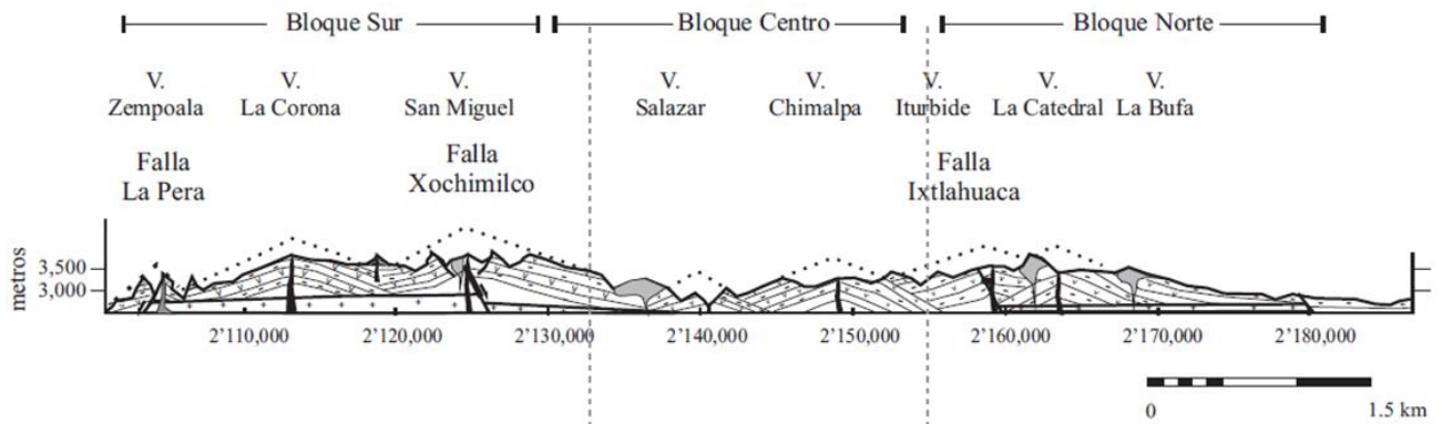
Figura # 2.9. Perfil geológico longitudinal sobre las ocho estructuras volcánicas de la Sierra de las Cruces.
