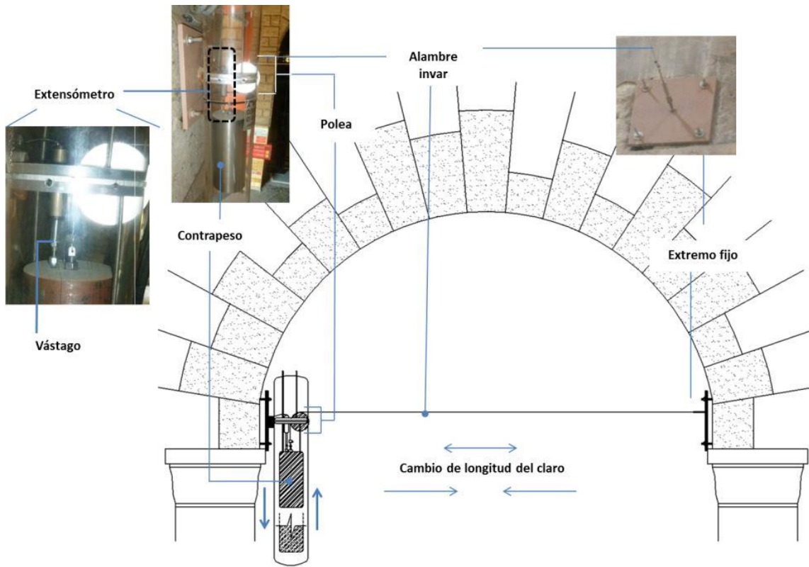
Figura 3.2 Configuración general de extensómetros
