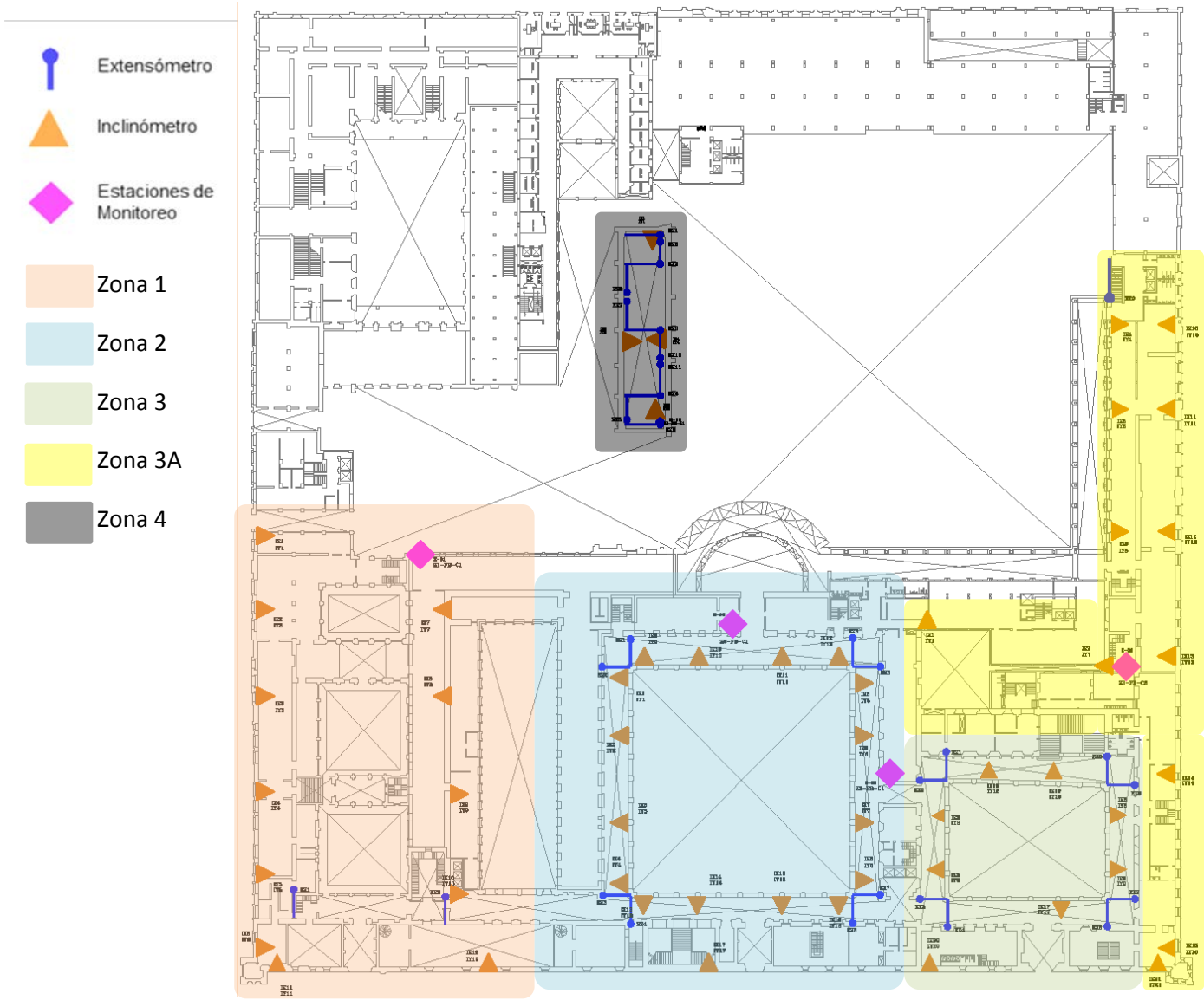
Figura 3.8 Zonas de monitoreo y ubicación de sensores
