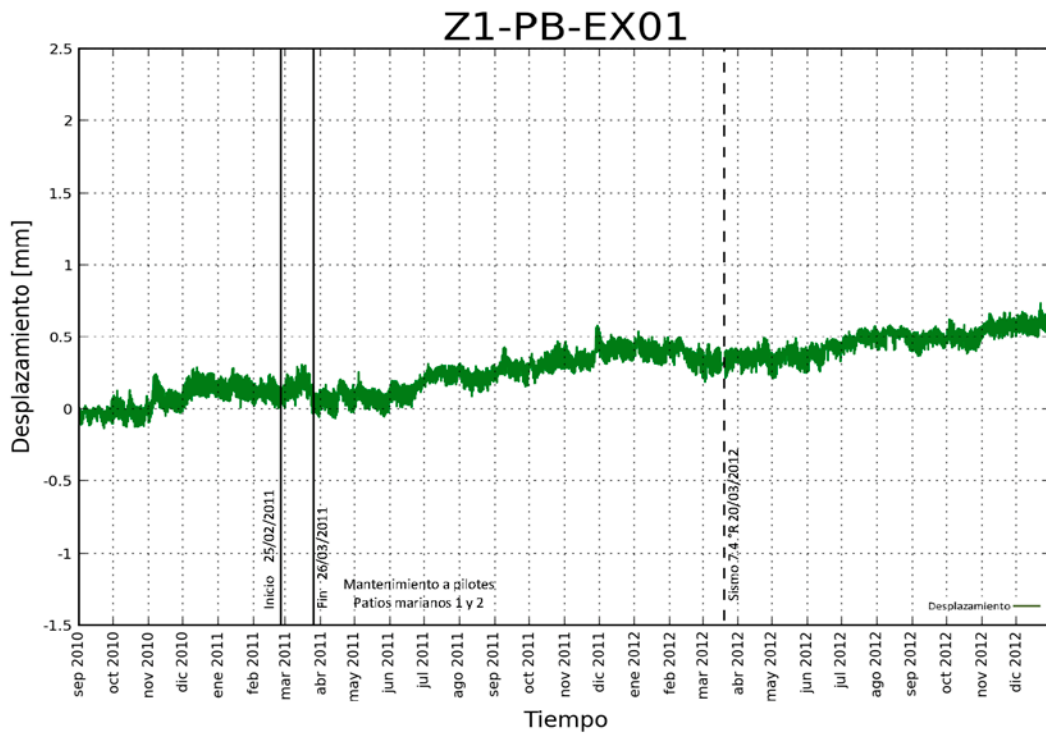
Figura 4.17 Gráfica correspondiente al extensómetro 1, zona 1
