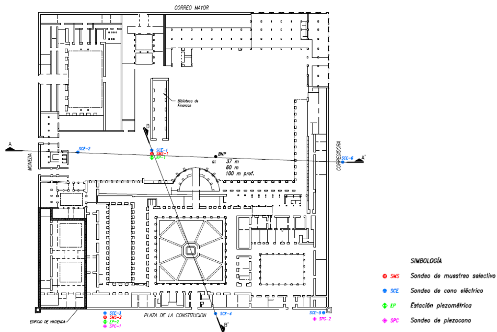
Figura 2.5 Ubicación de los Sondeos (Referencia 1)
