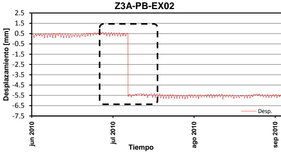
Figura 4.2 Corrimiento ocasionado por alteraciones al sensor sin salir del rango de operación
