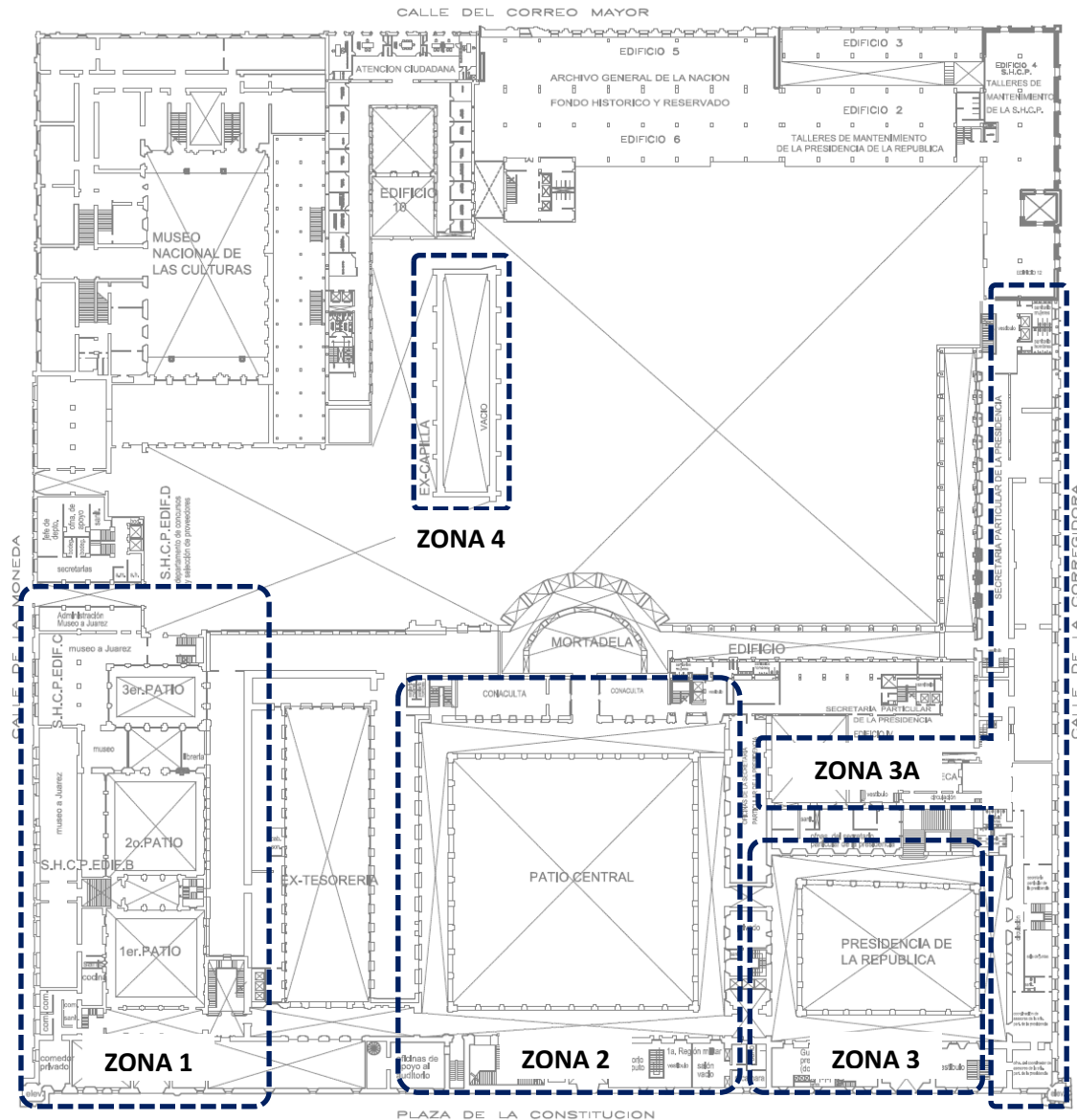
Figura 3.1 Distribución general de las zonas de monitoreo
