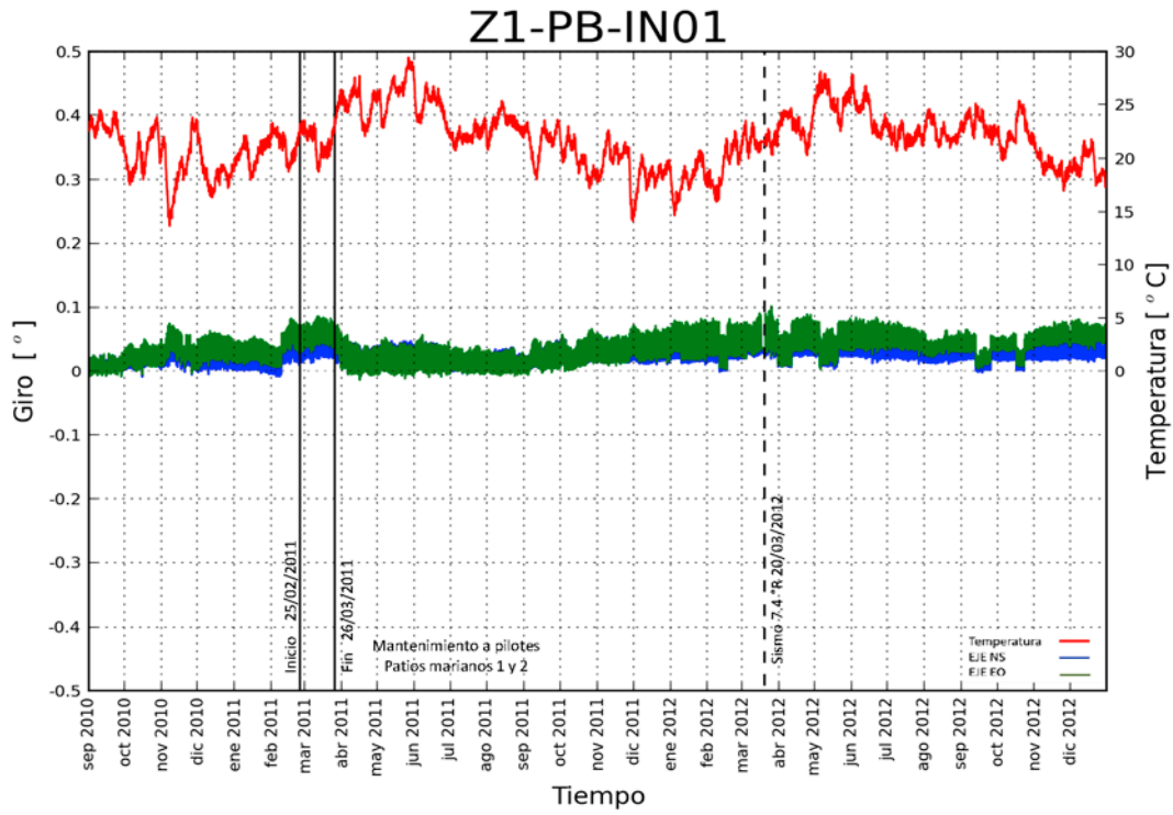
Figura 4.16 Gráfica correspondiente al inclinómetro 1, zona 1.
