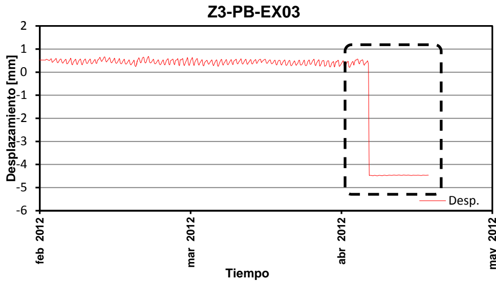
Figura 4.3 Corrimiento ocasionado por alteraciones al sensor y saliendo de su rango de operación
