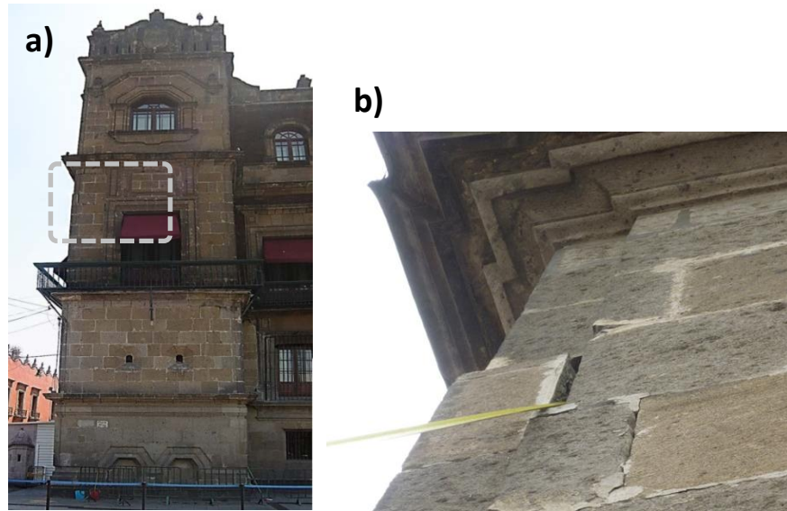
Figura 5.1-a) Apariencia y ubicación de los agrietamientos en el torreón norte; b) Detalle de agrietamiento en la fachada poniente del torreón norte
