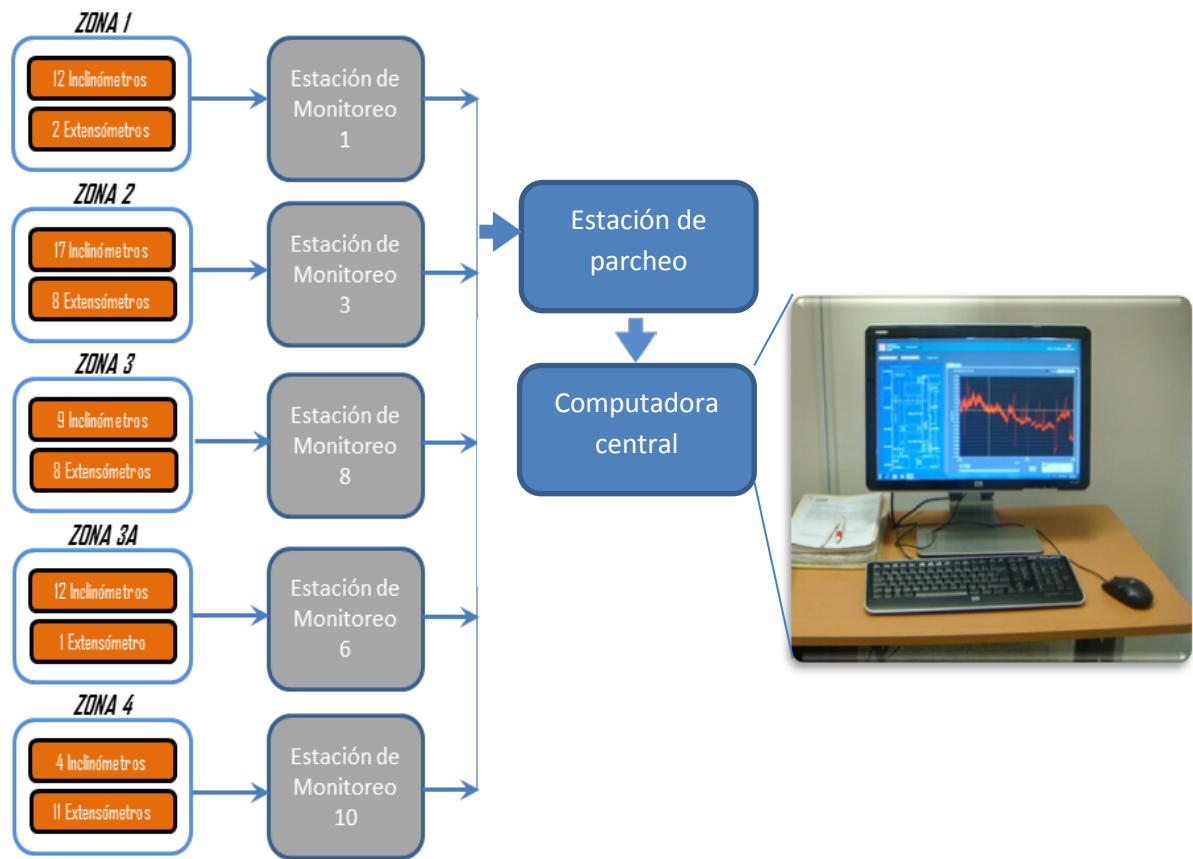
Figura 3.9 Funcionamiento General del Sistema de Monitoreo Continuo
