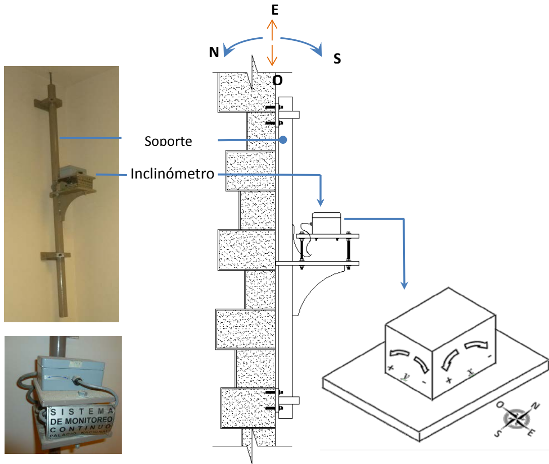
Figura 3.4 Instalación de un Inclinómetro
