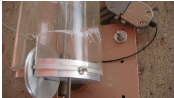
Figura 5.5 Extensómetro golpeado y dañado.
