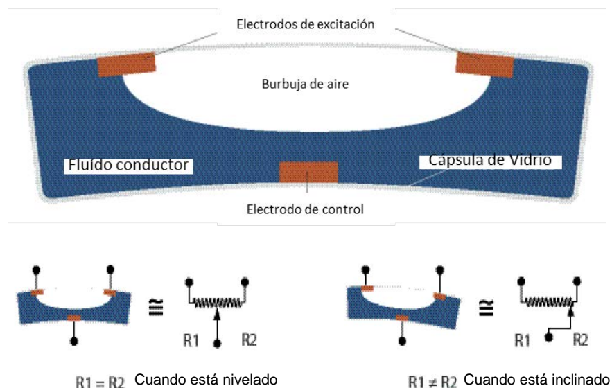
Figura 3.3 Inclinómetro potencimétrico-electrolítico
