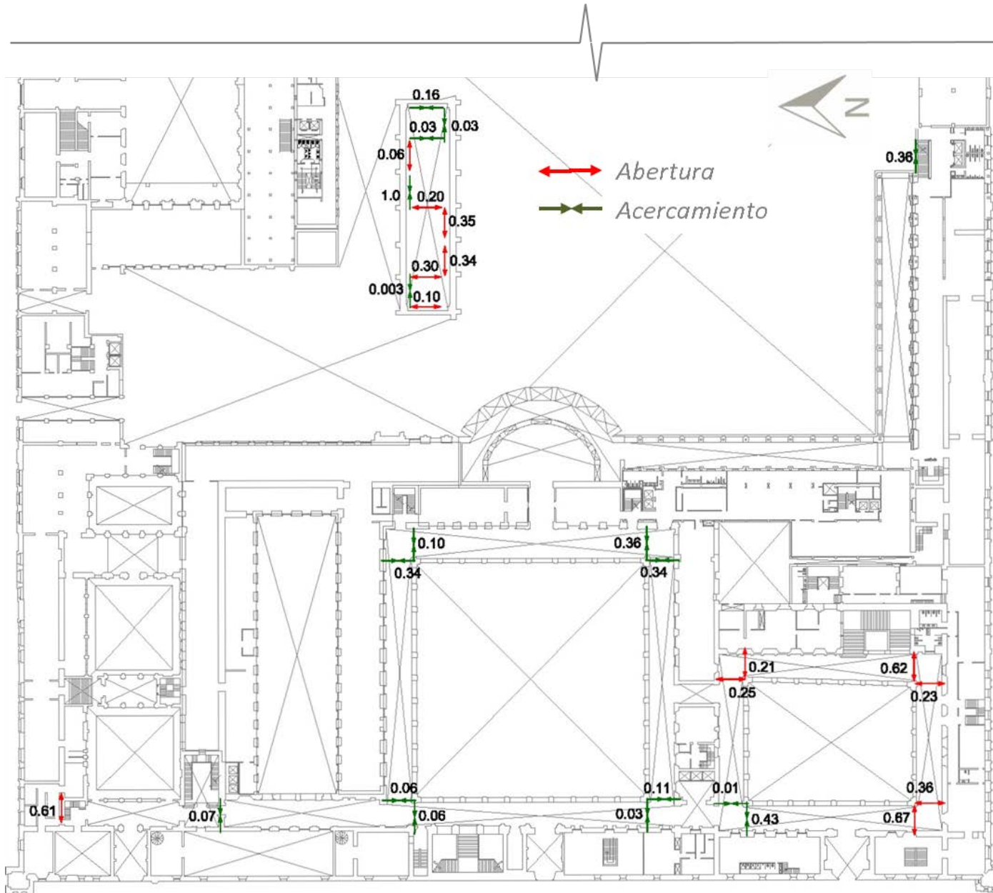
Figura 5.4-b Desplazamientos obtenidos por los extensómetros
