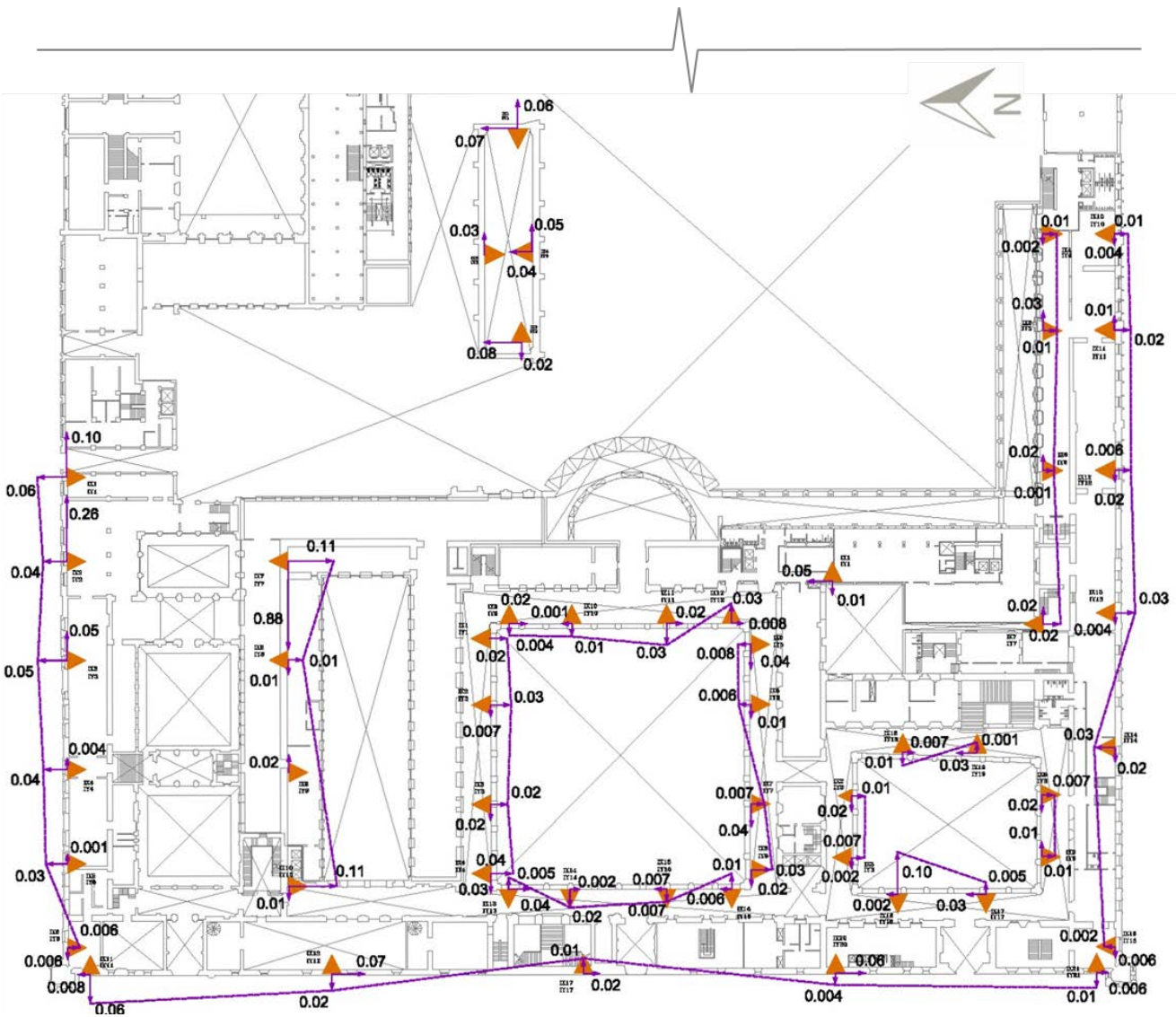
Figura 5.4-a Desplomes obtenidos por los inclinómetros
