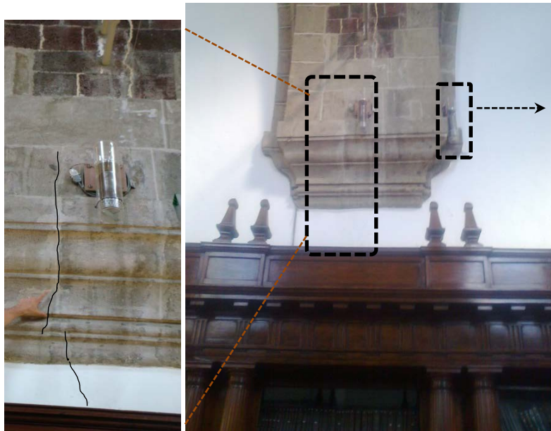
Figura 5.2. Ubicación de extensómetros 3 y 7, detalle de agrietamientos.
