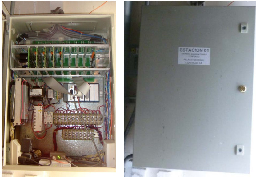
Figura 3.6 Vista interior y exterior de la estación de monitoreo 01
