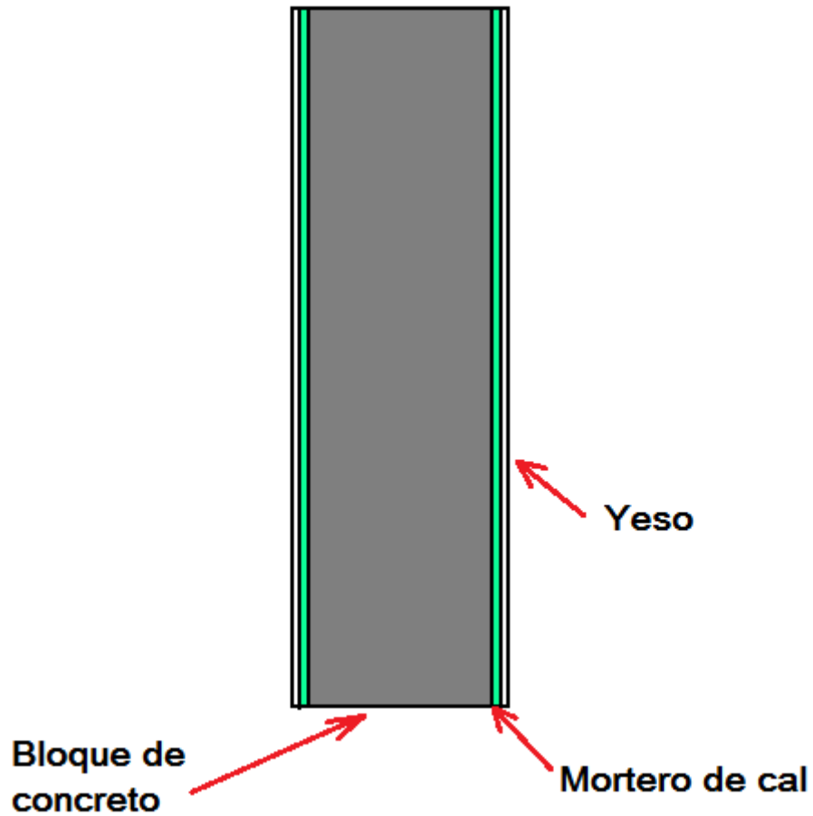
Figura 5.4 Capas que componen el muro de la vivienda prototipo
