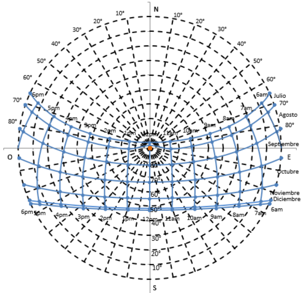
Figura 3.3 Gráfica solar estereográfica del DF, México, para el segundo semestre 18
