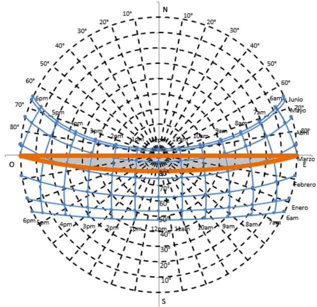
Fig. 3.10 Gráfica solar para un alero de 80° 21
