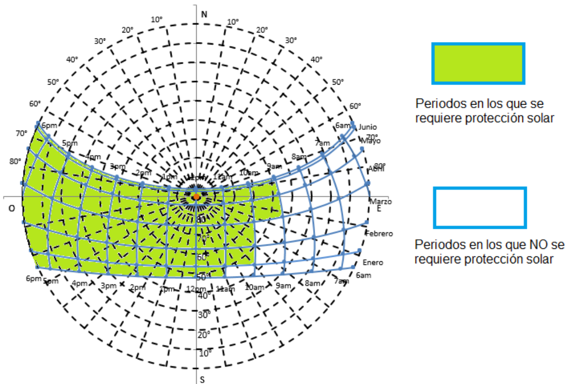
Figura 3.5 Consolidación de datos en una gráfica solar estereográfica 20
