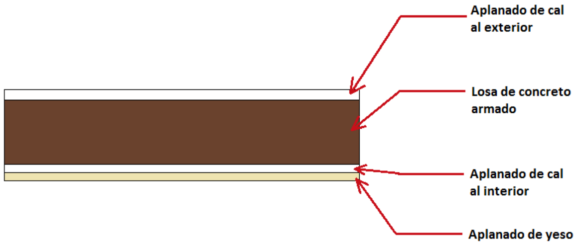
Figura 5.5 Capas que componen el techo de la vivienda prototipo
