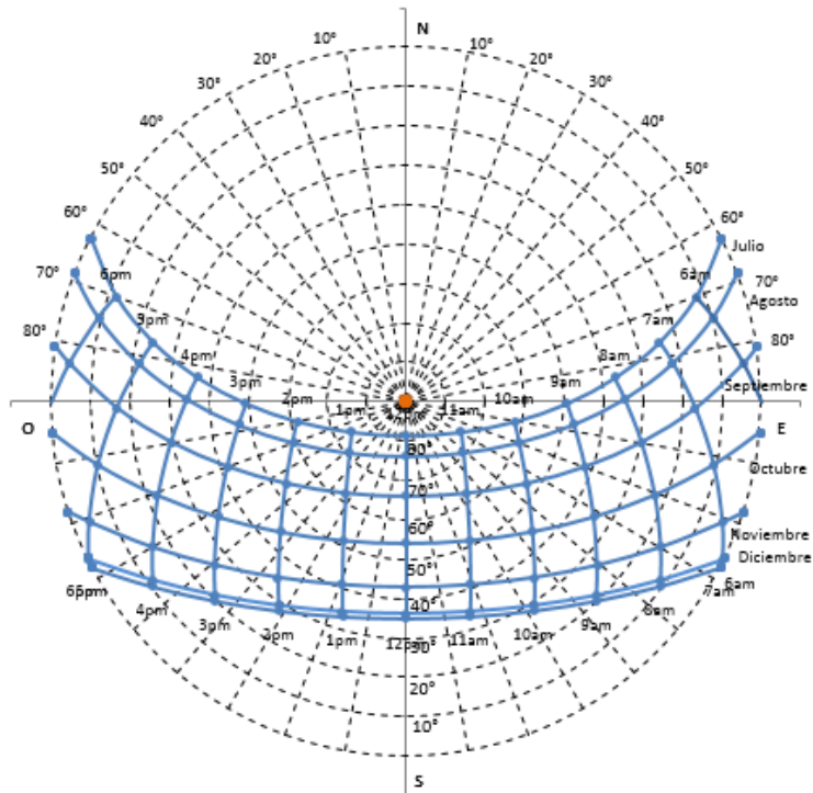
Fig. 4.4 Gráfica solar estereográfica de Ciudad Juárez para el segundo semestre 39
