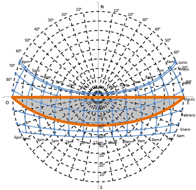
Fig. 3.12 Gráfica solar para un alero de 60° 22
