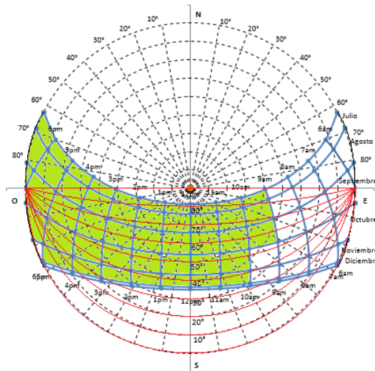
Figura 4.8 Superposición de la mascarilla de sombreado para la definición de aleros, segundo semestre 43
