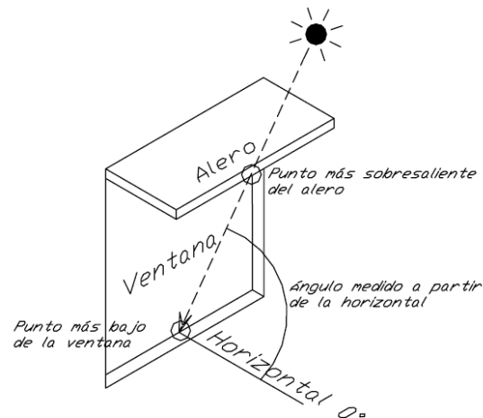
Fig. 2.1 Representación gráfica del ángulo de protección en el alero 3
