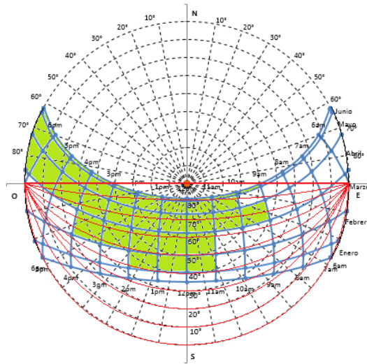
Figura 4.7 Superposición de la mascarilla de sombreado para la definición de aleros, primer semestre 42
