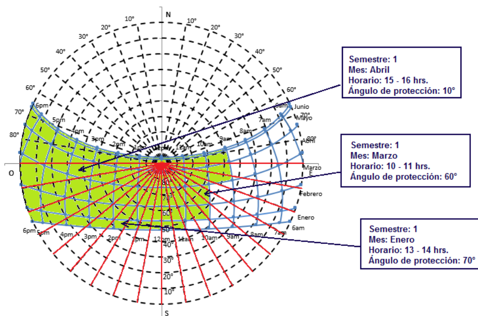
Figura 3.27 Ejemplos para la identificación de ángulos de protección para partesoles en la gráfica solar estereográfica 32
