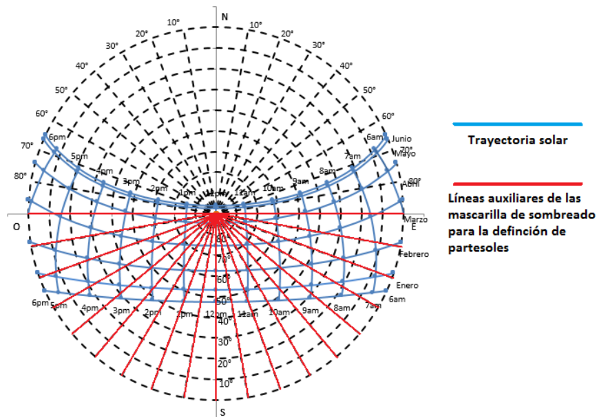
Figura 3.25 Mascarilla de sombreado sobrepuesta a la gráfica solar para la definición de partesoles 30
