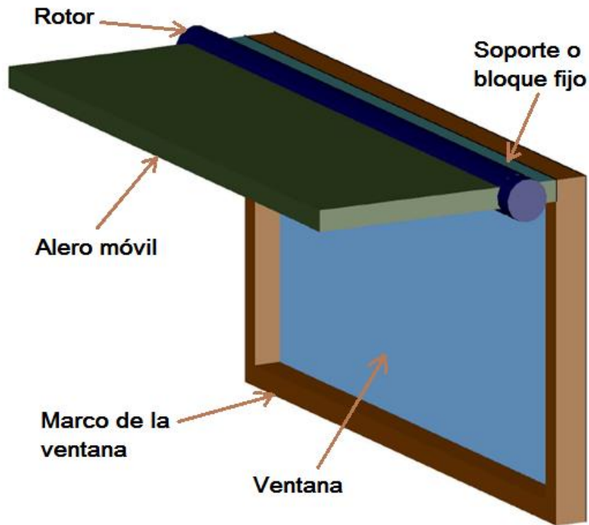
Fig. 3.29 Alero automatizado
