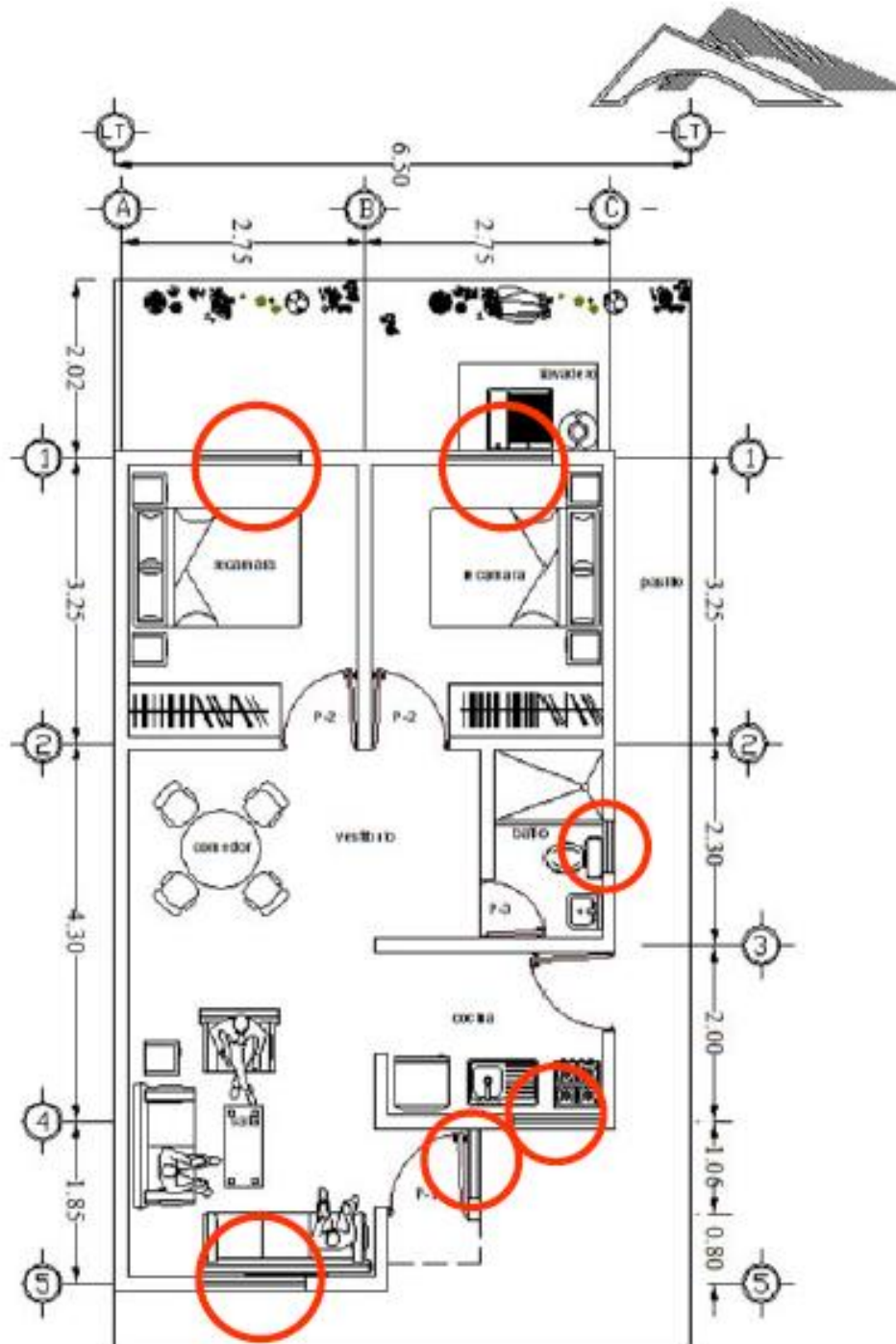
Figura 5.3 Planta arquitectónica de la vivienda de interés social con localización de las ventanas 58
