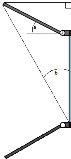
Fig 3.38 Relaciones trigonométricas en el partesol
