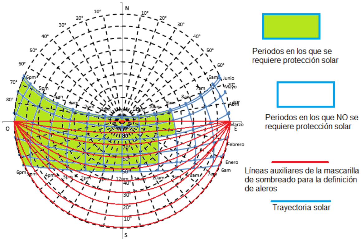
Figura 3.22 Mascarilla de sombreado superpuesta a la gráfica solar, con la representación de los requerimientos de protección, para la definición de aleros 28
