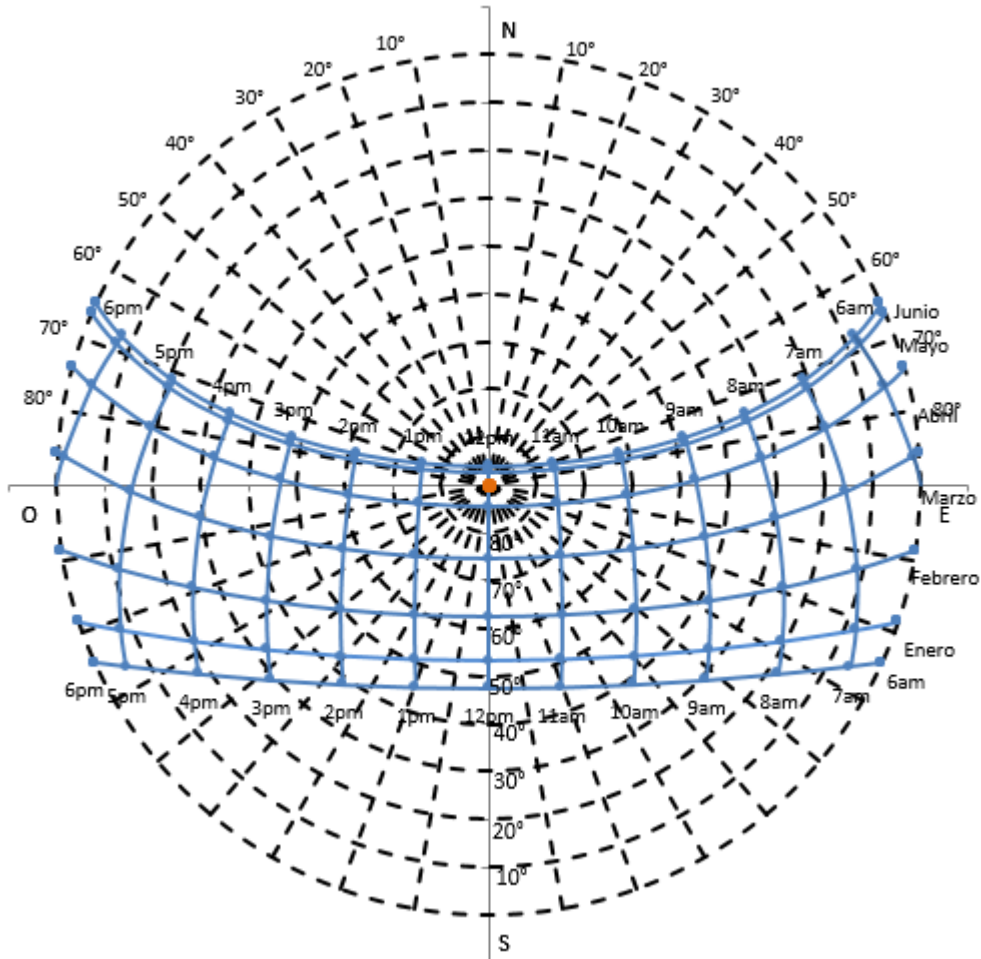
Figura 3.2 Gráfica solar estereográfica del DF, México, para el primer semestre 17
