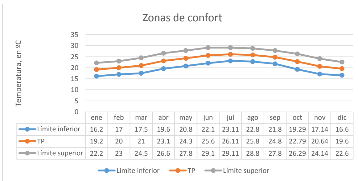
Figura 4.1 Gráfica de temperaturas de la zona de confort
