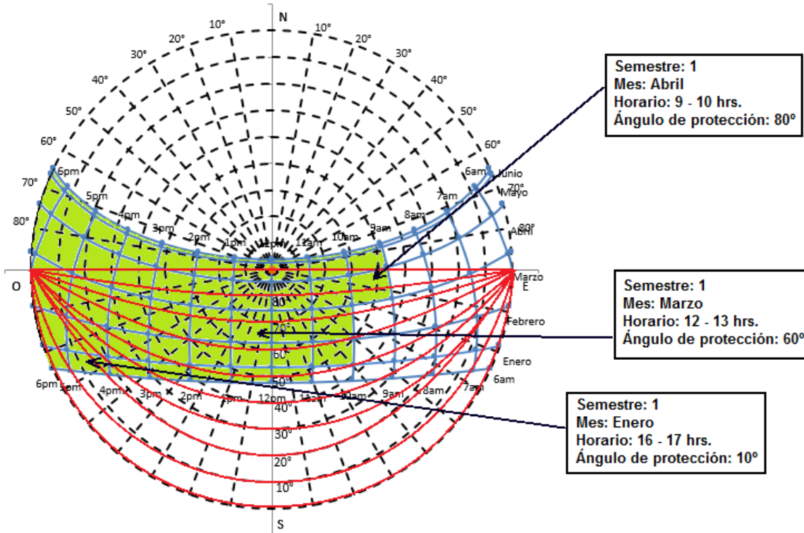
Figura 3.23 Ejemplos para la identificación de ángulos de protección en la gráfica solar estereográfica 29
