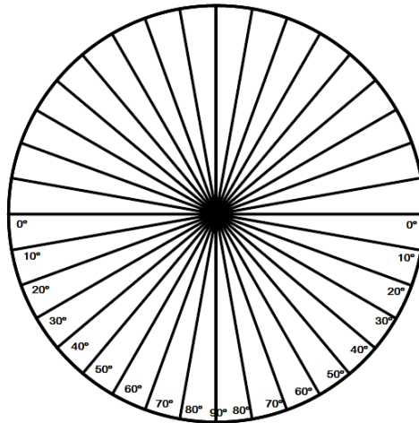
Figura 3.7 Líneas auxiliares de la mascarilla de sombreado para el análisis de la sombra efectuada por los partesoles
