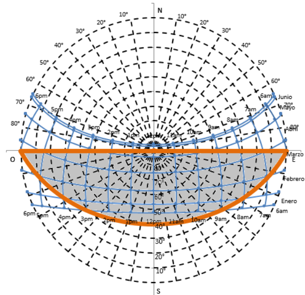
Fig. 3.14 Gráfica solar para un alero de 40° 23
