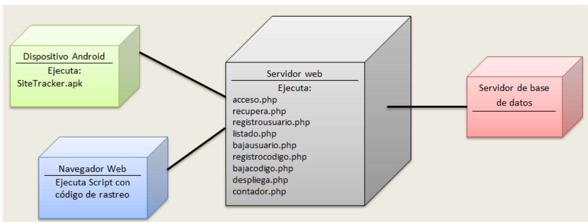
Figura 5.5. Diagrama de distribución. Diseño a nivel de componentes la solución propuesta.
