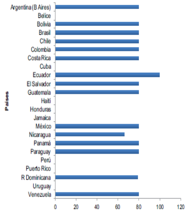
Gráfica 11 Estándar anual para SO 2
