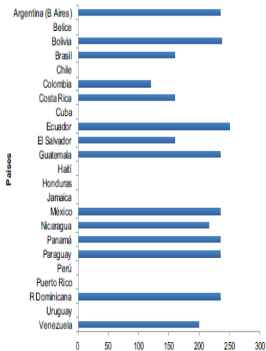
Gráfica 12 Estándar horario de O 3
