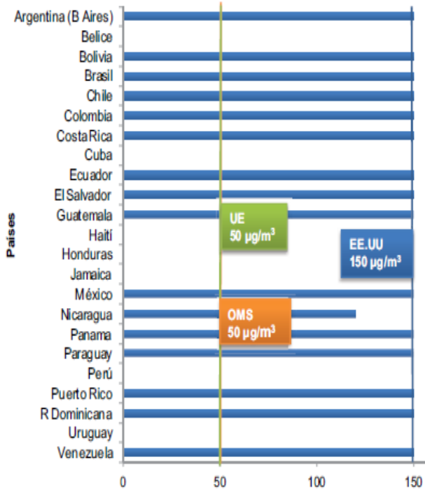
Gráfica 8 Estándar diario de PM 10
