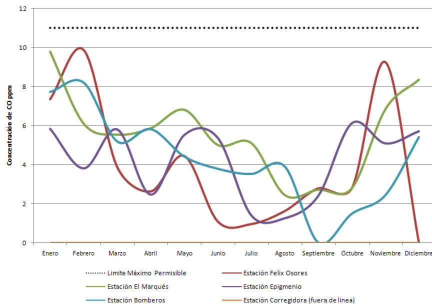
GRÁFICA 1 Concentraciones máximas de promedio móvil de ocho horas de CO.
