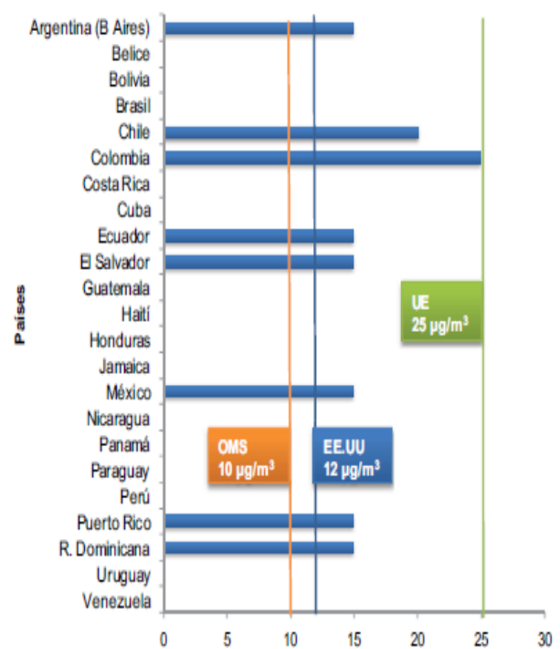
Gráfica 7 Estándar anual para PM 2.5
