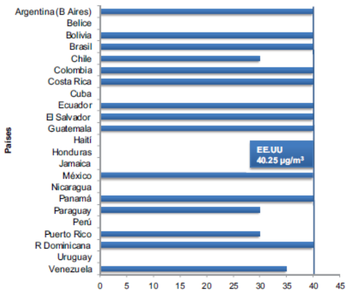
Gráfica 14 Estándar horario de CO
