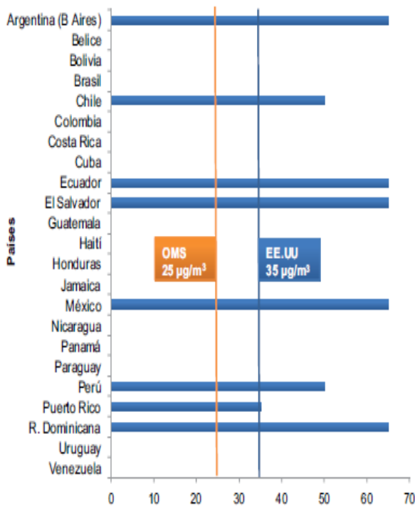
Gráfica 6 Estándar diario para PM 2.5
