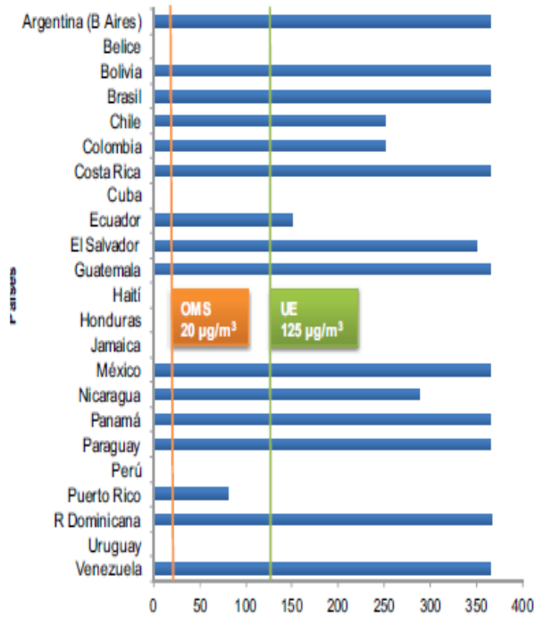
Gráfica 10 Estándar diario para SO 2
