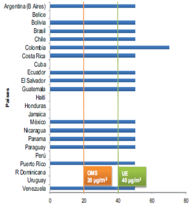
Gráfica 9 Estándar anual para PM 10
