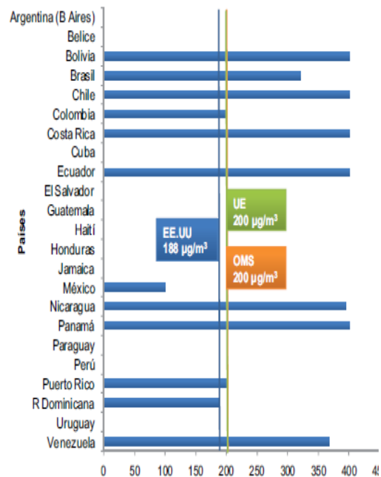
Gráfica 13 Estándar horario de NO
