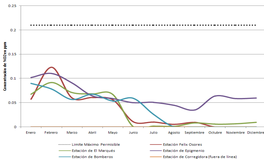
GRÁFICA 2 Máximos mensuales de concentración NO 2
