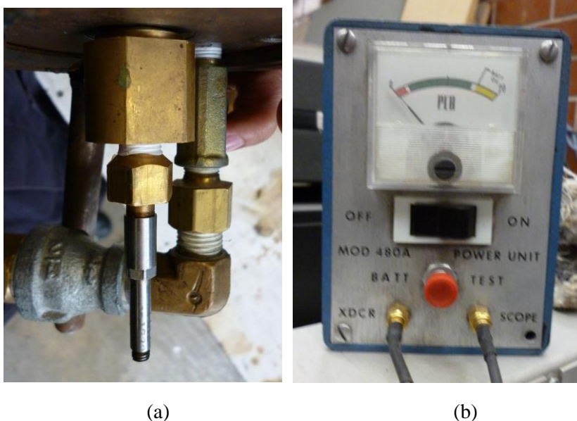
Figura 3.22 Sensor de presión de la cámara y acondicionador de señal.
