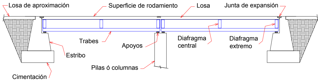
Figura 3.4 Principales componentes de un puente
