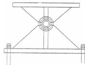
Apoyo de perno o pasador (Pin Bearing)
