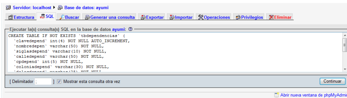
Figura 2. Estructura de la tabla tbdependencias en el editor de MySQL.
