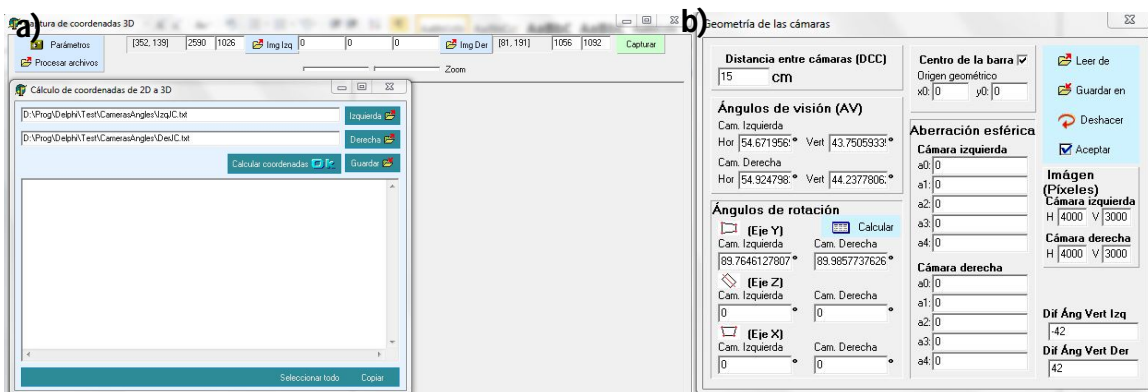
Fig. 13 LT3D. a) Interfaz grafica principal de LT3D con el rubro de cálculo de coordenadas 3D, b) es posible modificar parámetros de calibración como ángulos de visión, distancia entre cámaras, ángulos de rotación, resolución de imágenes.
